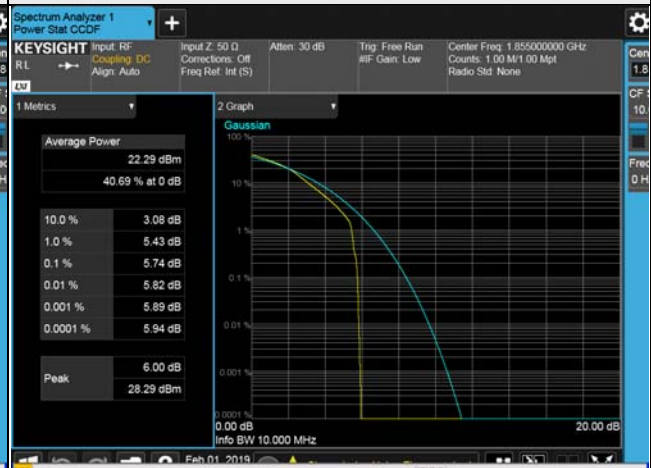
20MHz / 16QAM
