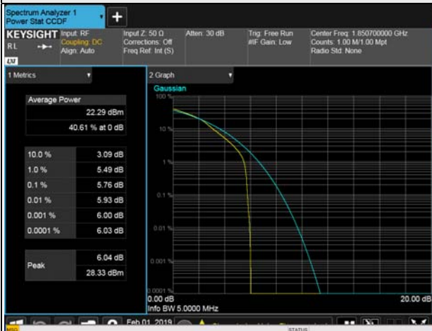
5MHz / 16QAM
