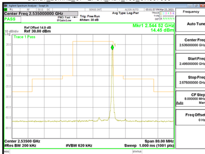
Band7_20MHz_CP-QPSK_RB1_105_CH507000
