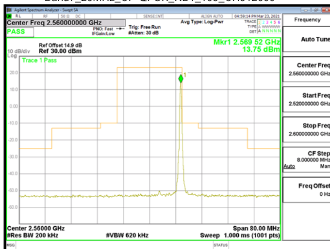
Band7_20MHz_CP-QPSK_RB1_105_CH512000
