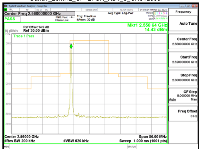
Band7_20MHz_CP-QPSK_RB1_0_CH512000
