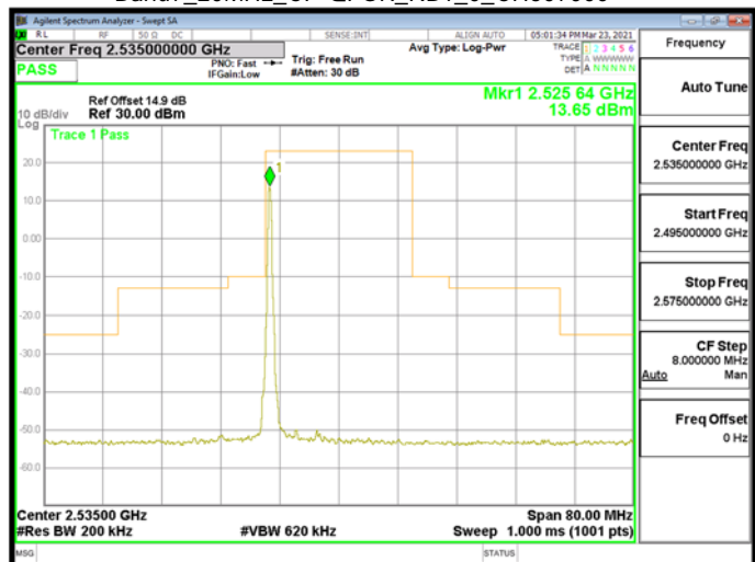
Band7_20MHz_CP-QPSK_RB1_0_CH507000
