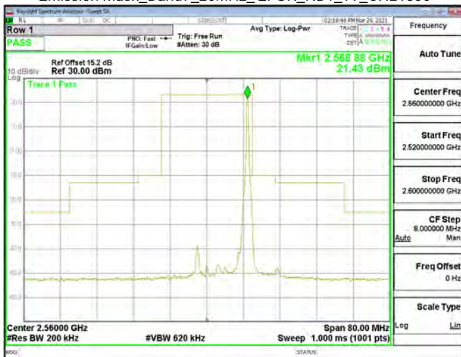
Emission Mask_Band7_20MHz_QPSK_RB1_99_CH21350
