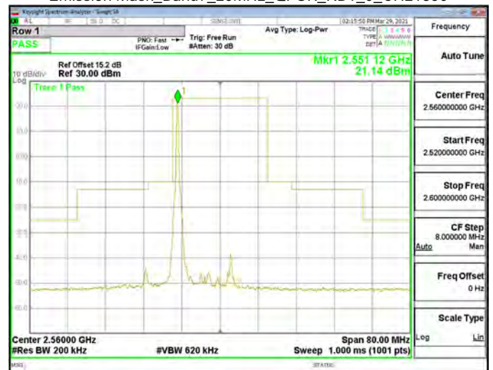
Emission Mask_Band7_20MHz_QPSK_RB1_0_CH21350
