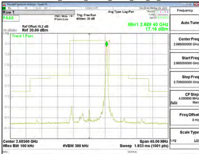
Emission Mask_Band41_10MHz_QPSK_RB1_49_CH41540
