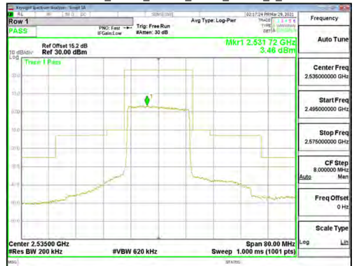
Emission Mask_Band7_20MHz_QPSK_RB100_0_CH21350
