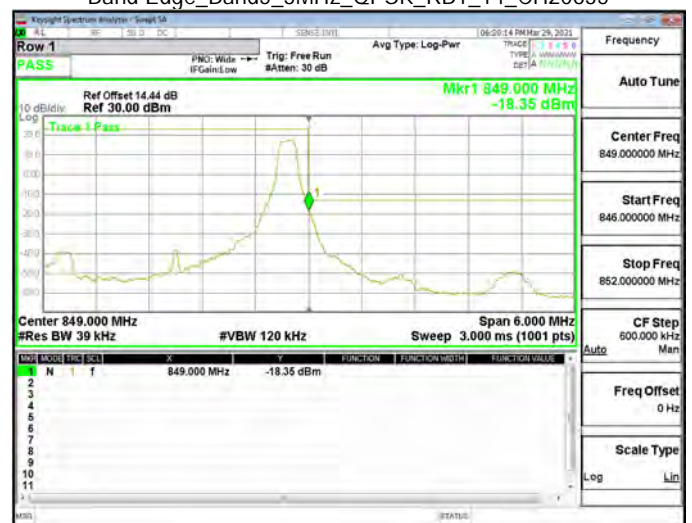
Band Edge_Band5_3MHz_QPSK_RB1_14_CH20635
