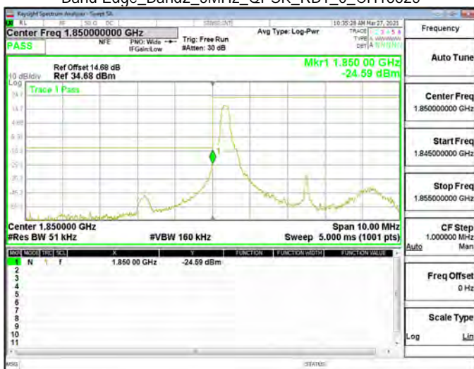
Band Edge_Band2_5MHz_QPSK_RB1_0_CH18625
