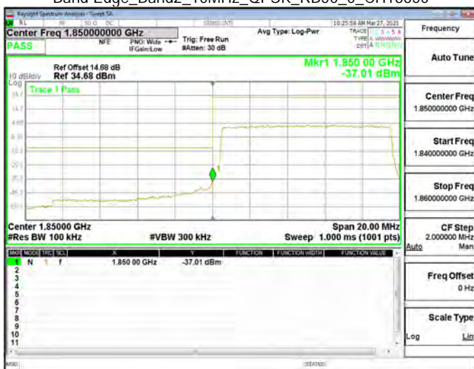
Band Edge_Band2_10MHz_QPSK_RB50_0_CH18650
