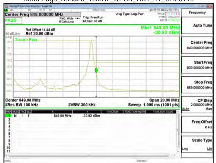
Band Edge_Band26_10MHz_QPSK_RB1_49_CH26990
