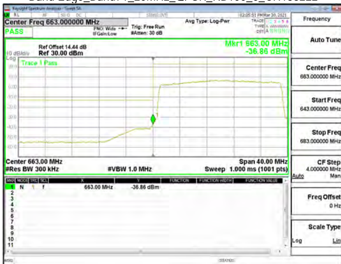
Band Edge_Band71_20MHz_QPSK_RB100_0_CH133222
