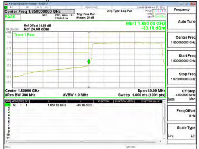
Band Edge_Band2_20MHz_QPSK_RB100_0_CH19100
