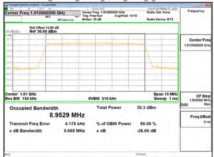
OBW_Band25_10MHz_QPSK_RB50_0_CH26640
