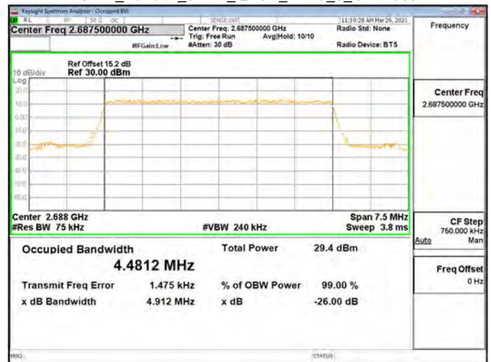
OBW_Band41_5MHz_QPSK_RB25_0_CH41565
