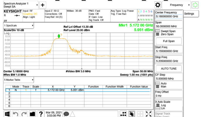
802.11ax_20MHz_Chain0_5180MHz_RU52_37
