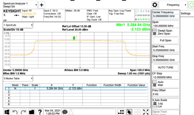
802.11ac_80MHz_Chain1_5290MHz
