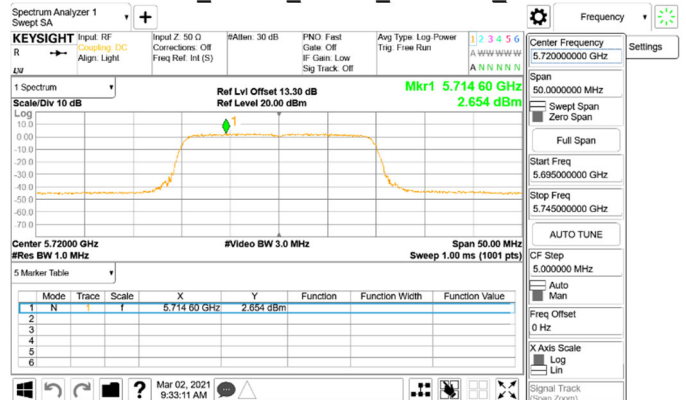
802.11ax_20MHz_Chain0_5720MHz_UNI2_2C
