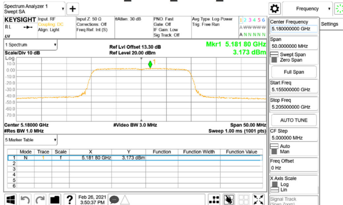
802.11ax_20MHz_Chain0_5180MHz
