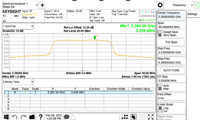
802.11ax_20MHz_Chain0_5260MHz
