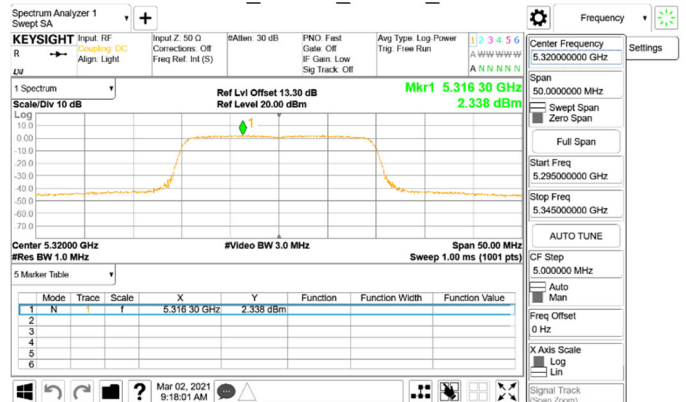
802.11ax_20MHz_Chain0_5320MHz_RU106_54
