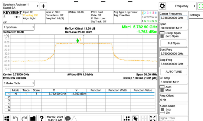
802.11ax_20MHz_Chain0_5785MHz
