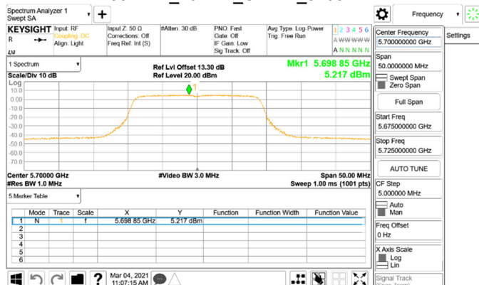
802.11n_20MHz_Chain1_5700MHz
