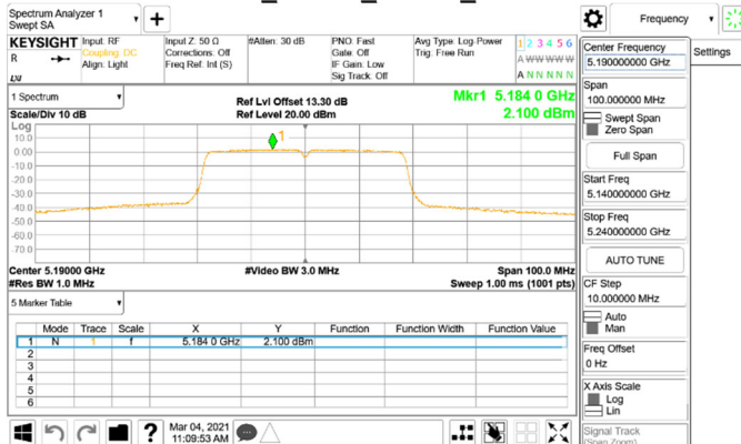
802.11n_40MHz_Chain0_5190MHz
