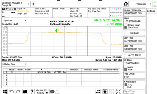
802.11ac_80MHz_Chain0_5530MHz
