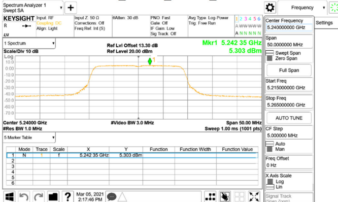
802.11n_20MHz_Chain1_5240MHz
