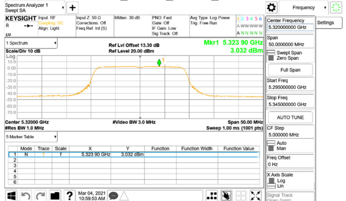
802.11n_20MHz_Chain1_5320MHz
