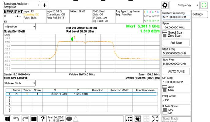
802.11n_40MHz_Chain0_5310MHz
