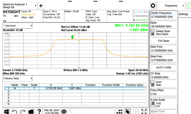
802.11n_20MHz_Chain1_5745MHz
