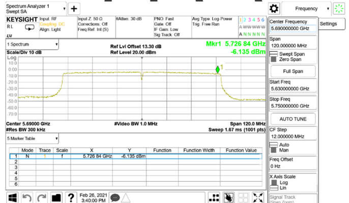
802.11ac_80MHz_Chain0_5690MHz_UNII 3
