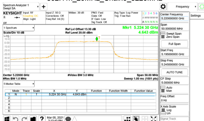
802.11n_20MHz_Chain0_5220MHz
