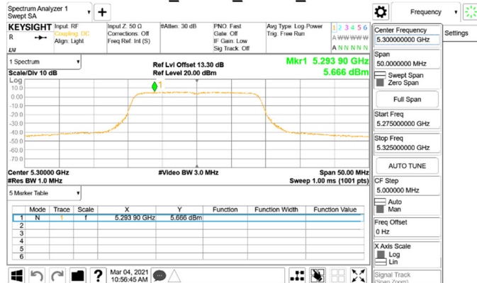
802.11n_20MHz_Chain0_5300MHz
