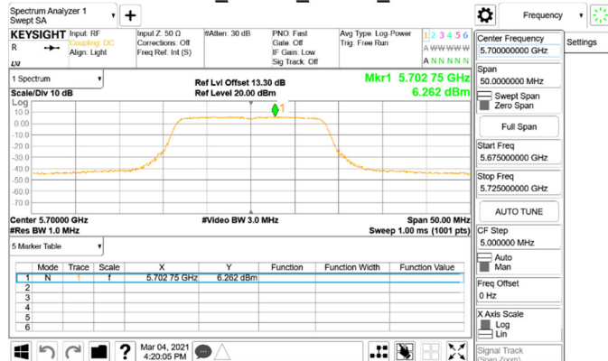
802.11a_20MHz_Chain0_5700MHz
