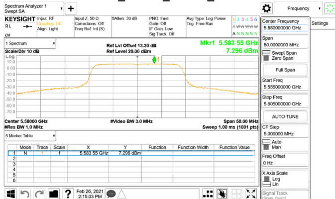
802.11n_20MHz_Chain0_5580MHz
