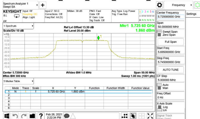
802.11n_20MHz_Chain0_5720MHz_UNII 3
