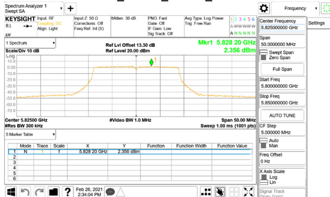
802.11n_20MHz_Chain0_5825MHz
