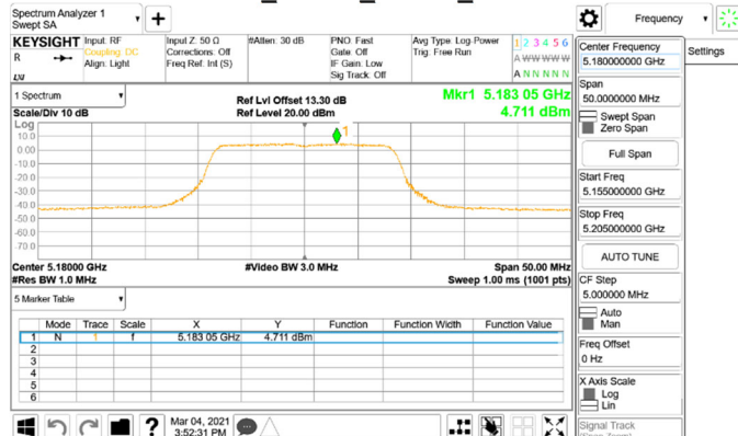
802.11a_20MHz_Chain1_5180MHz
