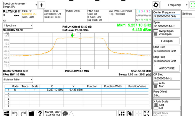
802.11a_20MHz_Chain1_5260MHz
