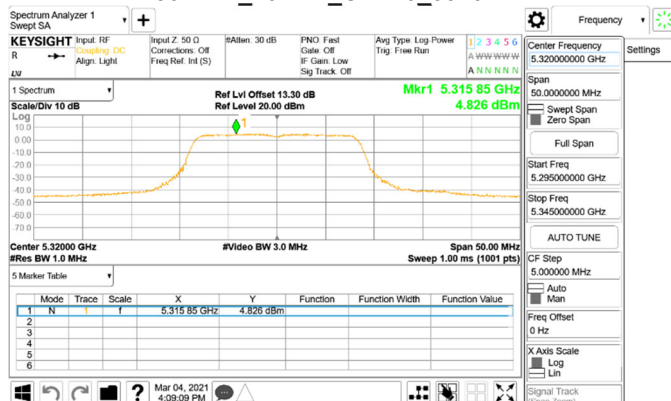
802.11a_20MHz_Chain0_5320MHz
