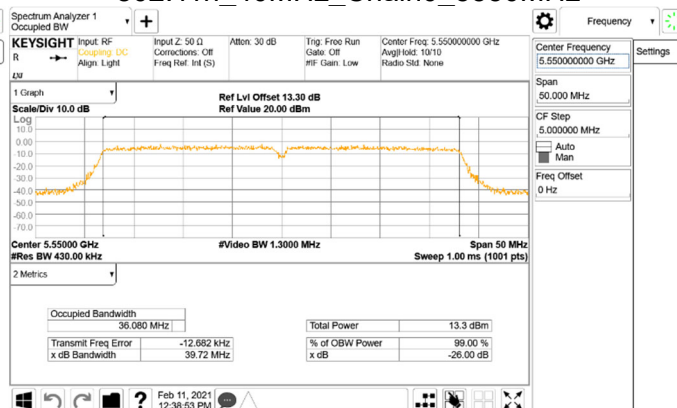
802.11n_40MHz_Chain0_5550MHz
