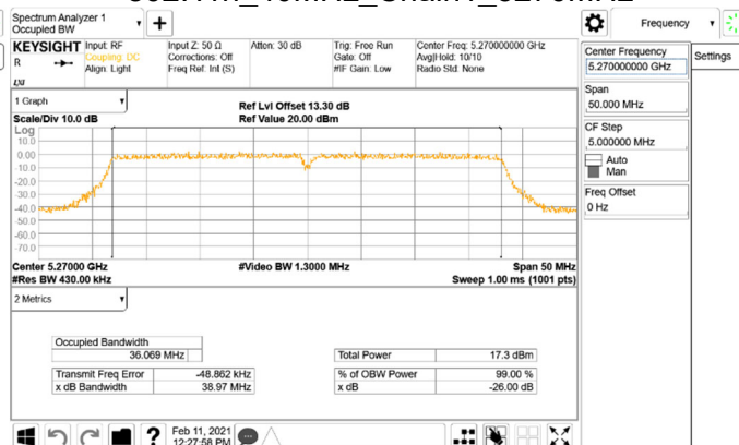
802.11n_40MHz_Chain1_5270MHz
