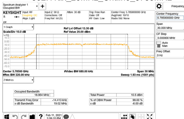
802.11ax_20MHz_Chain0_5785MHz
