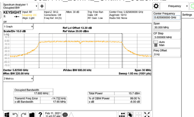
802.11n_20MHz_Chain1_5825MHz
