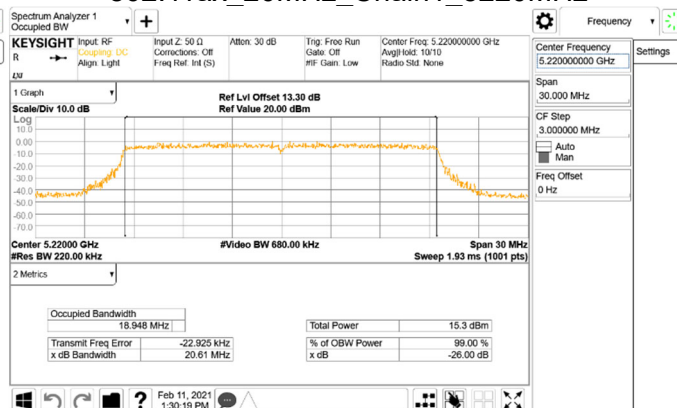
802.11ax_20MHz_Chain1_5220MHz
