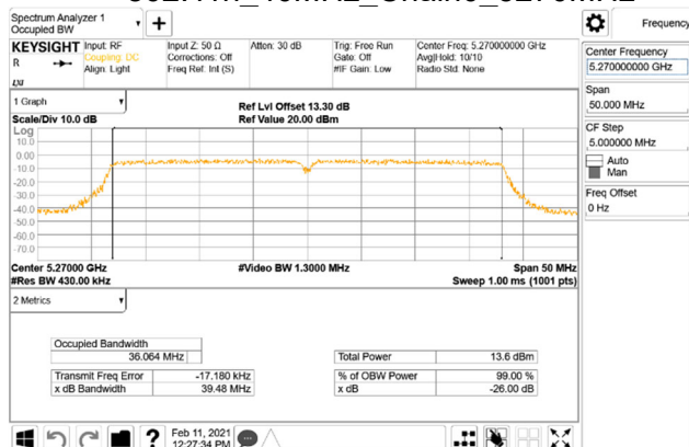
802.11n_40MHz_Chain0_5270MHz
