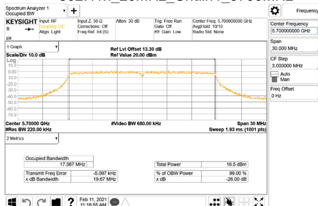
802.11n_20MHz_Chain1_5700MHz
