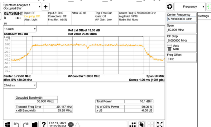
802.11n_40MHz_Chain1_5795MHz
