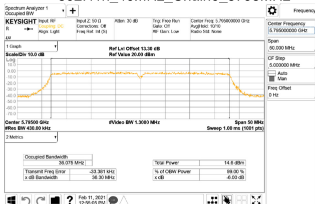
802.11n_40MHz_Chain0_5795MHz
