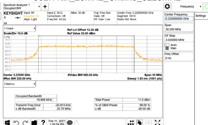
802.11ax_20MHz_Chain0_5220MHz
