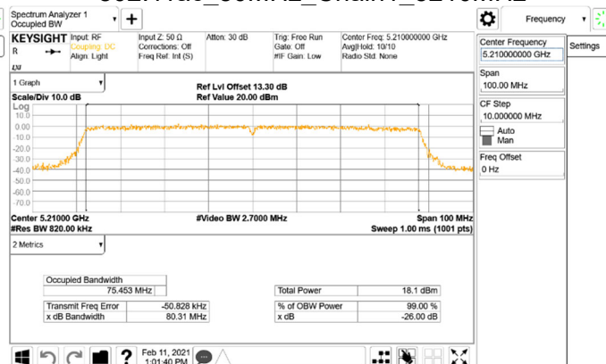
802.11ac_80MHz_Chain1_5210MHz
