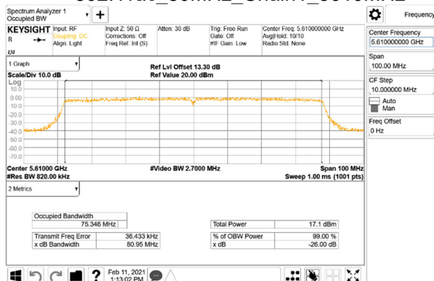
802.11ac_80MHz_Chain1_5610MHz
