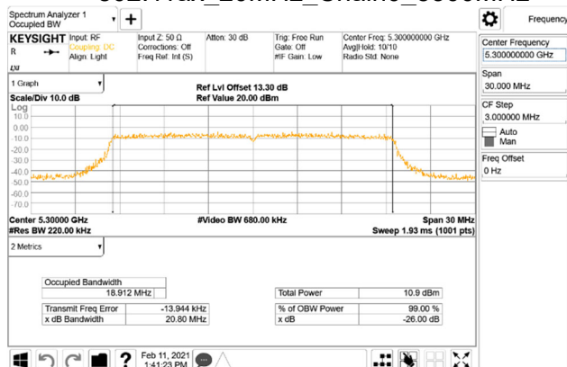
802.11ax_20MHz_Chain0_5300MHz
