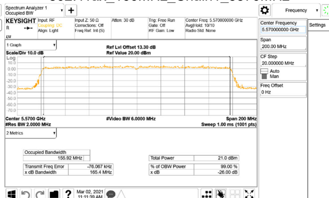
802.11ax_160MHz_Chain1_5570MHz
