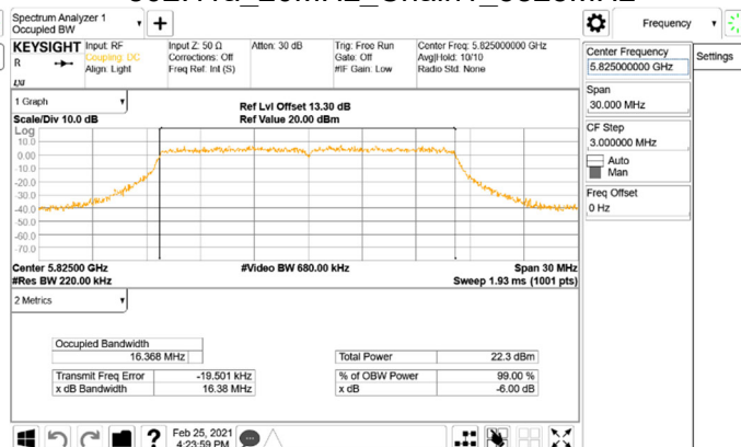
802.11a_20MHz_Chain1_5825MHz
