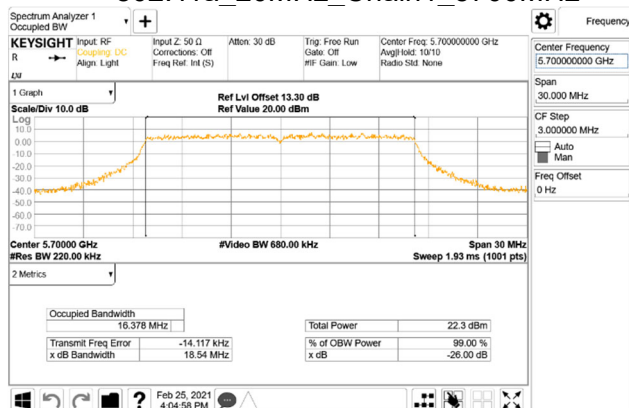
802.11a_20MHz_Chain1_5700MHz
