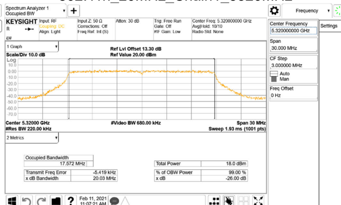
802.11n_20MHz_Chain1_5320MHz
