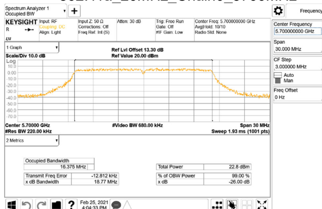
802.11a_20MHz_Chain0_5700MHz
