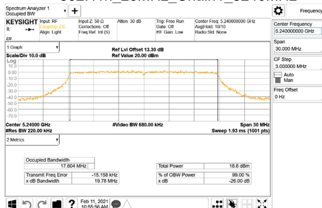
802.11n_20MHz_Chain1_5240MHz
