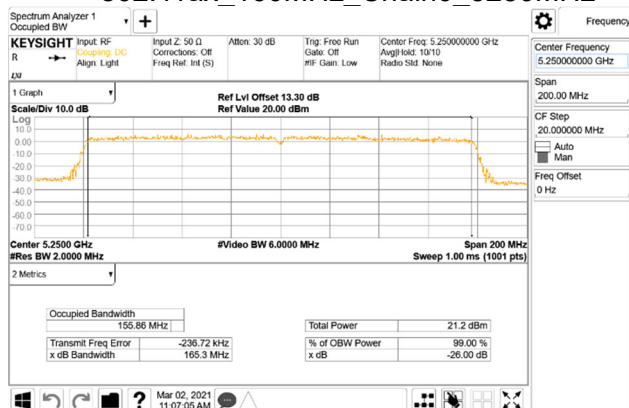
802.11ax_160MHz_Chain0_5250MHz
