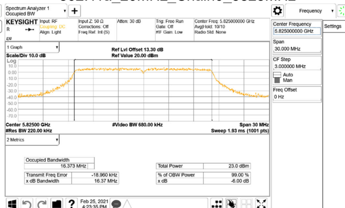
802.11a_20MHz_Chain0_5825MHz
