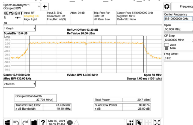
802.11ax_40MHz_Chain0_5510MHz
