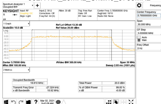
802.11ax_20MHz_Chain0_5785MHz
