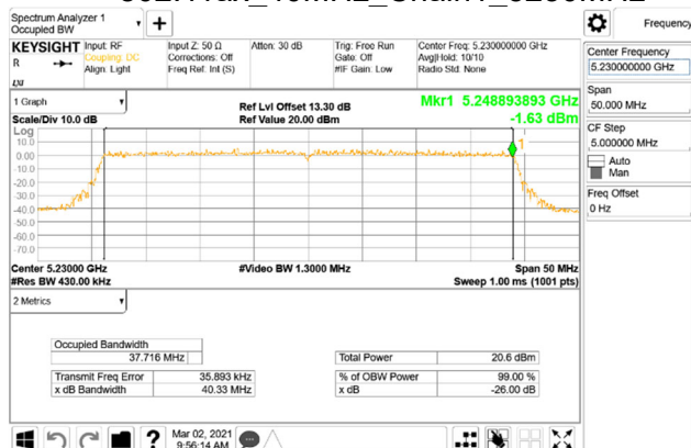
802.11ax_40MHz_Chain1_5230MHz
