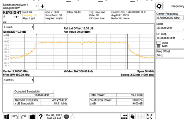
802.11ax_20MHz_Chain1_5785MHz
