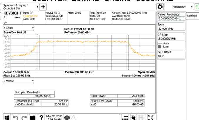
802.11ax_20MHz_Chain0_5580MHz
