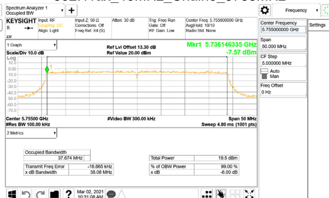
802.11ax_40MHz_Chain0_5755MHz
