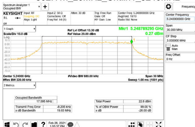
802.11n_20MHz_Chain1_5240MHz
