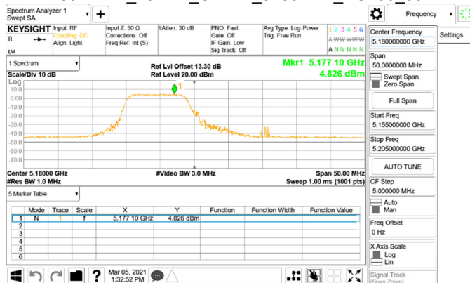
802.11ax_20MHz_Chain1_5180MHz_RU106_53
