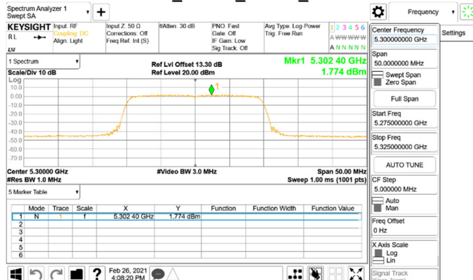
802.11ax_20MHz_Chain1_5300MHz
