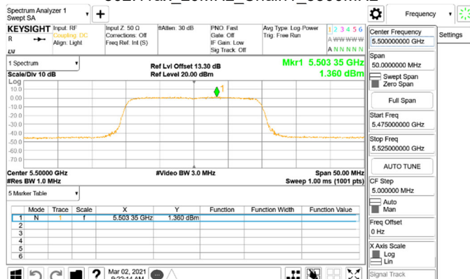
802.11ax_20MHz_Chain1_5500MHz_RU106_53
