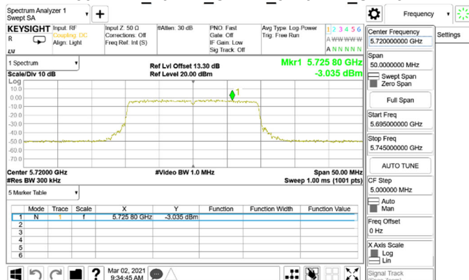
802.11ax_20MHz_Chain1_5720MHz_UNII 3
