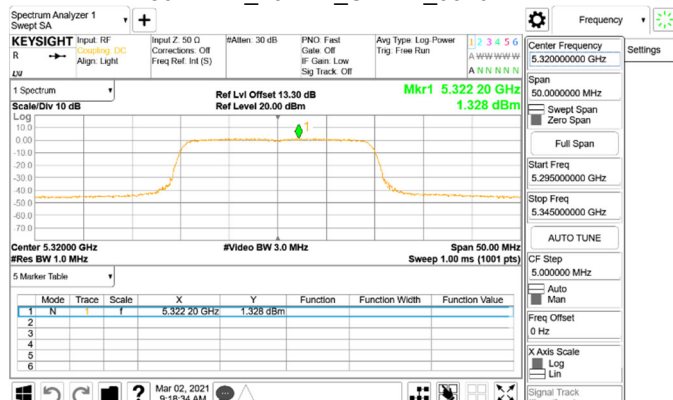
802.11ax_20MHz_Chain1_5320MHz_RU106_54
