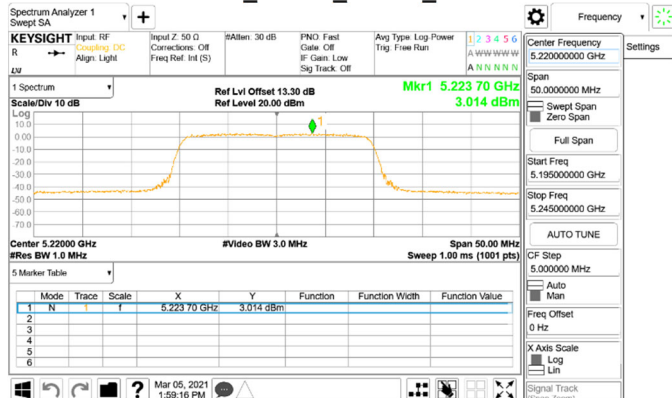
802.11ax_20MHz_Chain1_5220MHz
