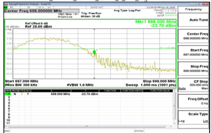
CP-OFDM_Band71_20MHz_QPSK_1_105_HighCH137600-688
