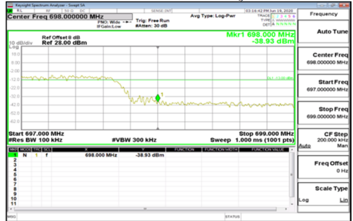
CP-OFDM_Band71_10MHz_QPSK_52_0_HighCH138600-693
