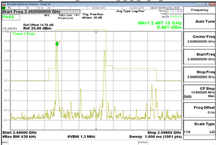
Mask_LTE\Band41_40MHz\QPSK_1_0_1_99_CH_Low2516
