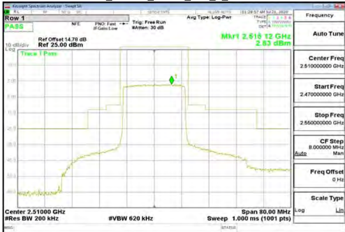
Band7_20MHz_QPSK_100_0_CH20850
