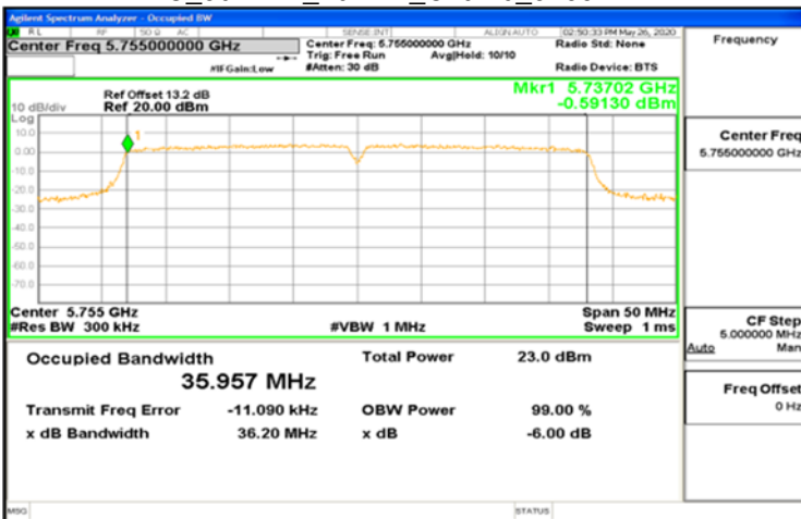
IC_802.11n_40MHz_Chain0_5755MHz
