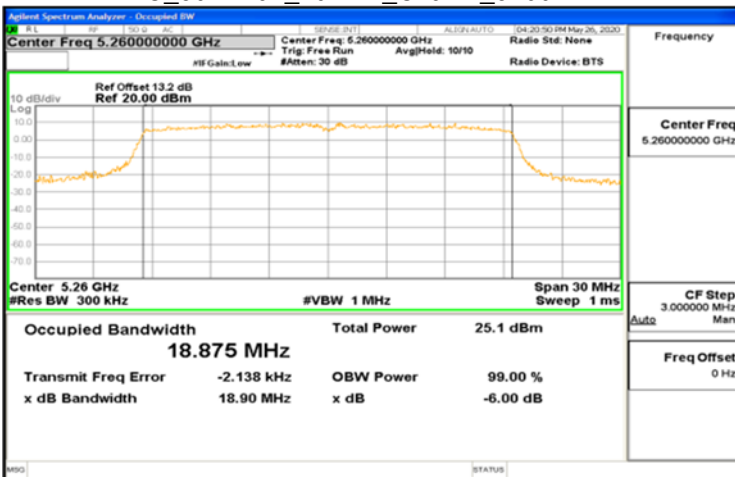
IC_802.11ax_20MHz_Chain1_5260MHz
