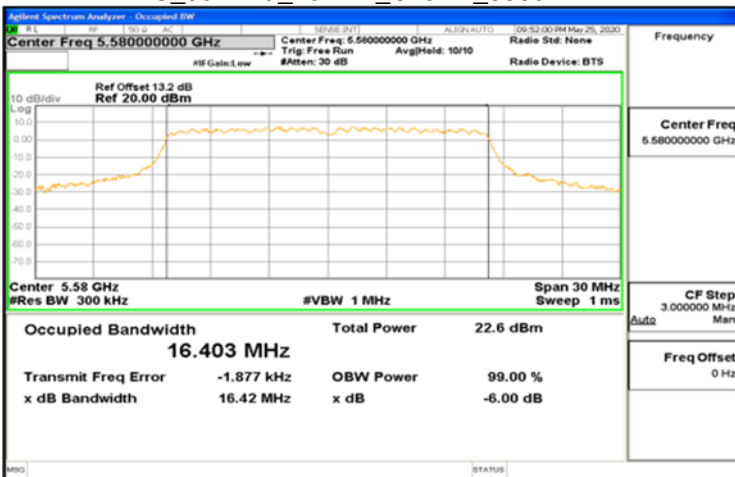
IC_802.11a_20MHz_Chain1_5580MHz
