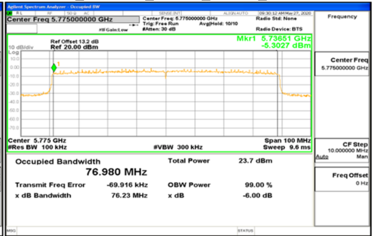
FCC_802.11ax_80MHz_Chain1_5775MHz
