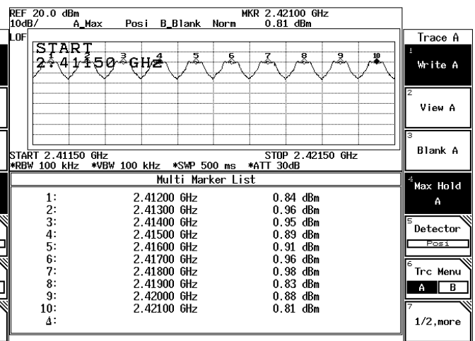
2412-2421MHz
