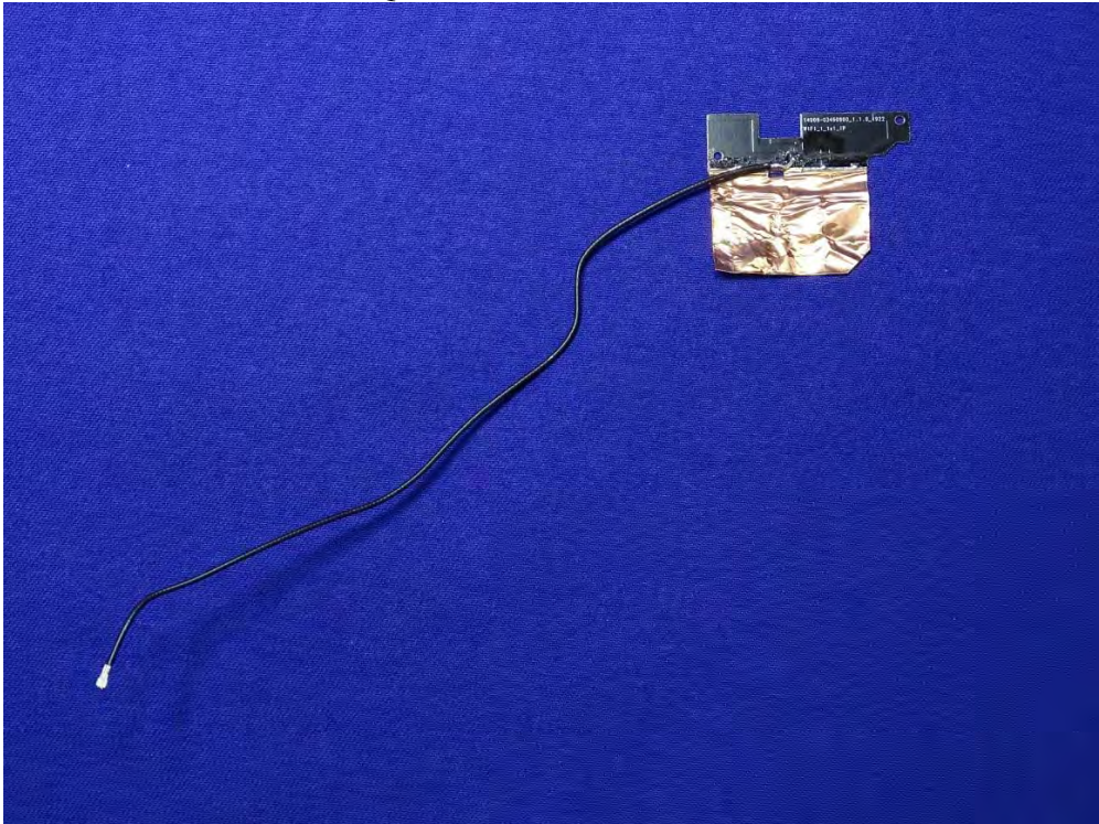
(64) EUT Photo_Antenna: INPAQ TX1 Main
