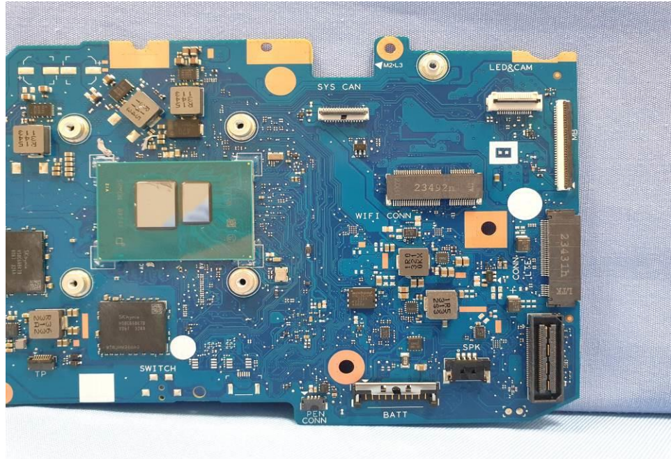
EUT Photo (50)
