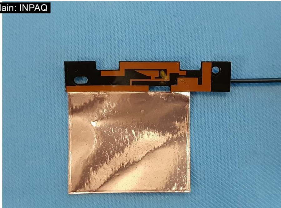
EUT Photo (20) WLAN antenna Main : INPAQ
