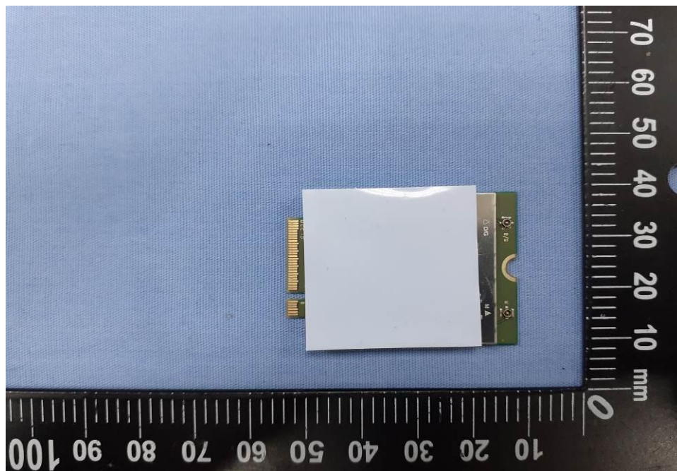
EUT Photo (8) WWAN module FM101-GL
