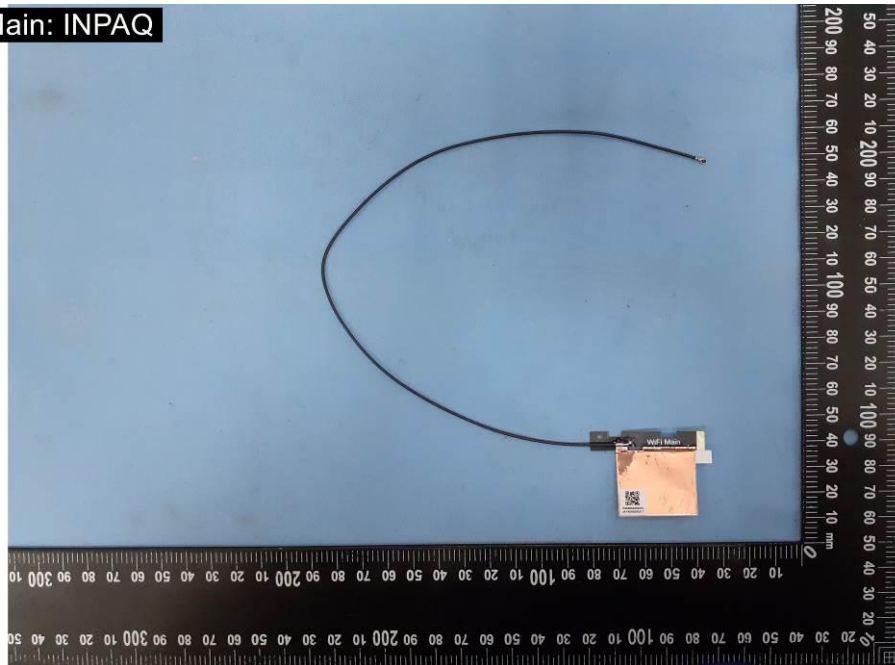
EUT Photo (18) WLAN antenna Main : INPAQ
