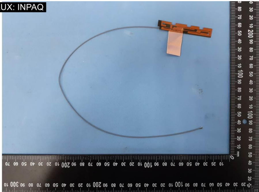
EUT Photo (32) WWAN antenna AUX : INPAQ
