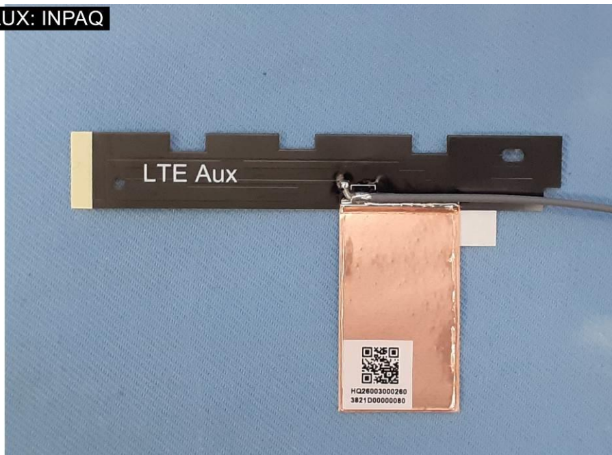
EUT Photo (30) WWAN antenna AUX : INPAQ
