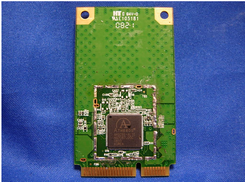
(44) EUT Photo
