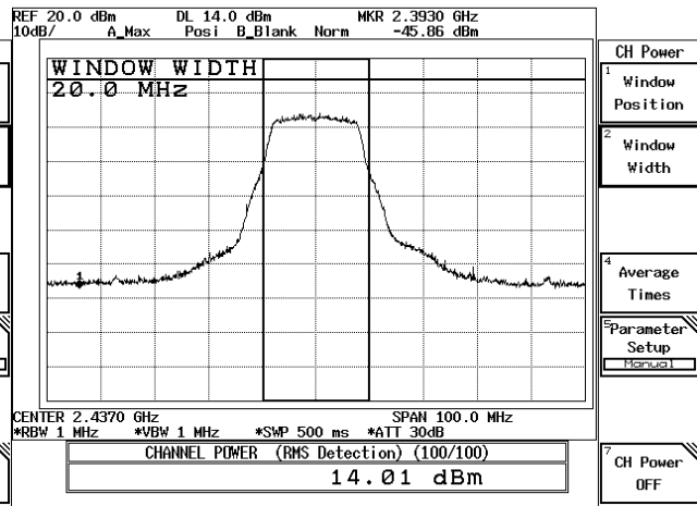
54Mbps-CH 06
