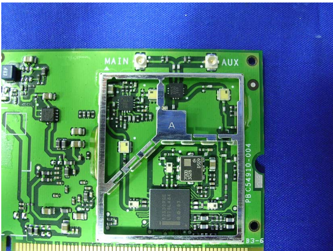
(20) EUT Photo
