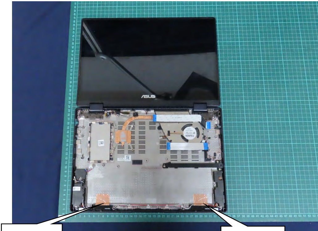
(20) EUT Photo
