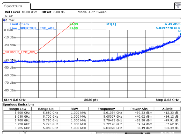
-BE-NR-LOW, SISO-A, 802.11ax20-HE0, Ch173
