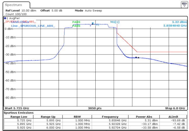
BE-NR-HIGH, MIMO-A, 802.11ax80-HE0, Ch171
