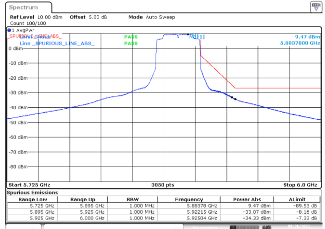
-BE-NR-HIGH, SISO-A, 802.11ax40-HE0, Ch175
