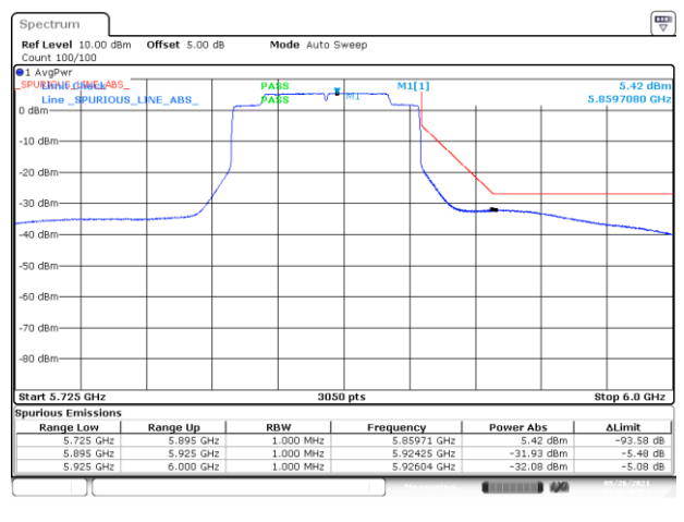
BE-NR-HIGH, MIMO-B, 802.11ax80-HE0, Ch171
