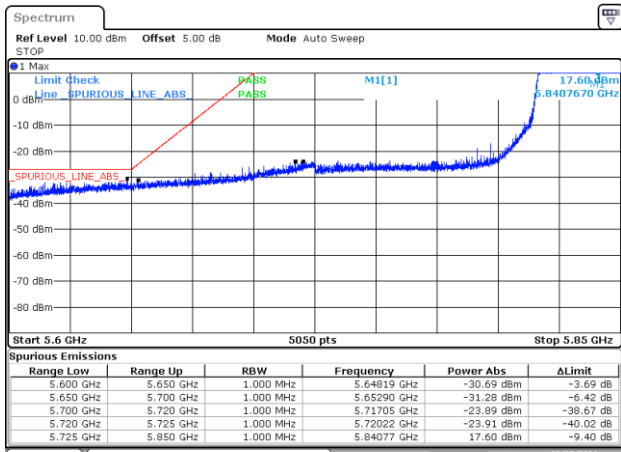
BE-NR-LOW, MIMO-A, 802.11ax80-HE0, Ch171
