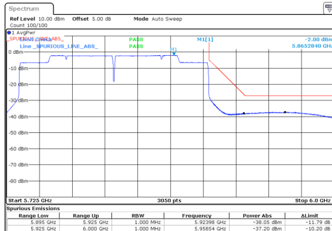
BE-NR-HIGH, MIMO-A, 802.11ax160-HE0, Ch163
