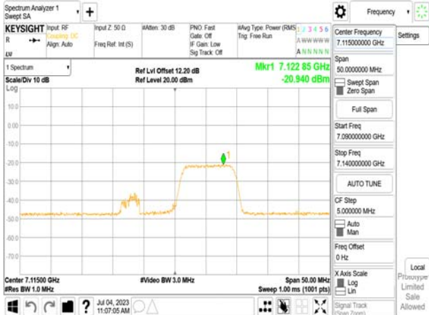
802.11be_20MHz_Chain0_7115MHz_RU106_54
