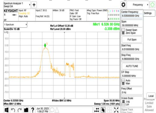
802.11be_20MHz_Chain1_6535MHz_RU26_0
