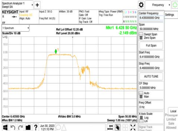
802.11be_20MHz_Chain0_6435MHz_106+26_MRU1
