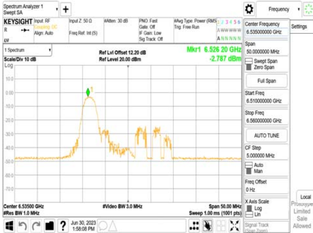
802.11be_20MHz_Chain0_6535MHz_RU52_37
