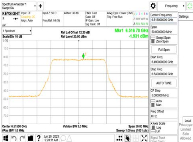
802.11be_20MHz_Chain1_6515MHz_106+26_MRU2
