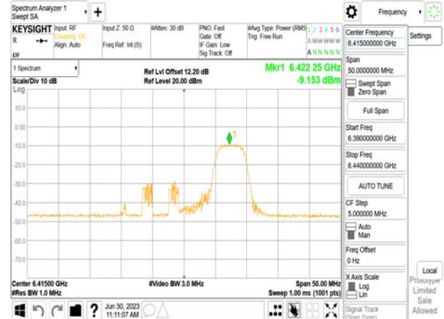
802.11be_20MHz_Chain1_6415MHz_RU52_40
