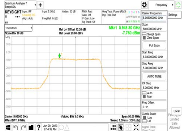
802.11be_20MHz_Chain1_5955MHz
