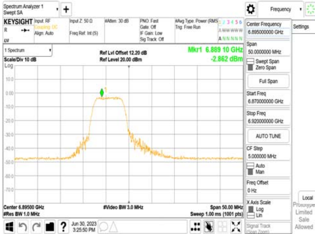
802.11be_20MHz_Chain0_6895MHz_RU106_53
