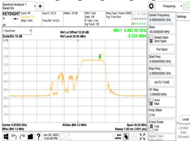
802.11be_20MHz_Chain0_6855MHz_RU26_8
