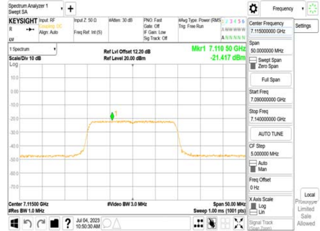
802.11be_20MHz_Chain1_7115MHz_106+26_MRU2
