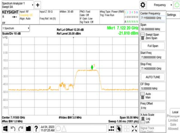
802.11be_20MHz_Chain1_7115MHz_RU26_8
