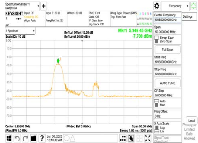
802.11be_20MHz_Chain0_5955MHz_RU52_37
