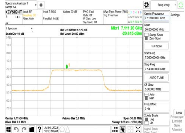
802.11be_20MHz_Chain0_7115MHz
