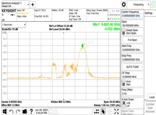
802.11be_20MHz_Chain1_6855MHz_RU52_40
