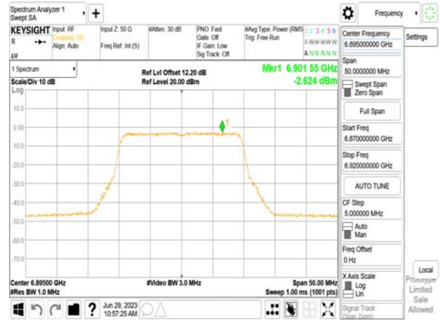
802.11be_20MHz_Chain0_6895MHz_106+26_MRU1
