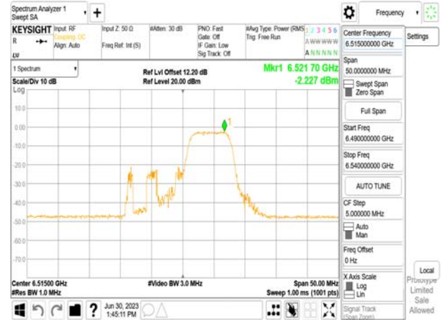
802.11be_20MHz_Chain1_6515MHz_RU106_54
