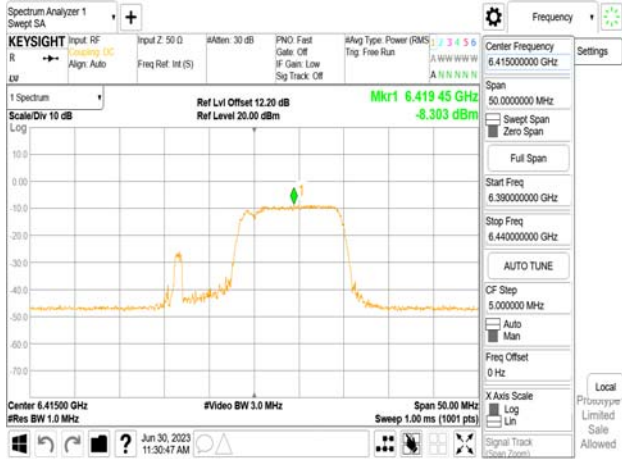
802.11be_20MHz_Chain1_6415MHz_52+26_MRU3
