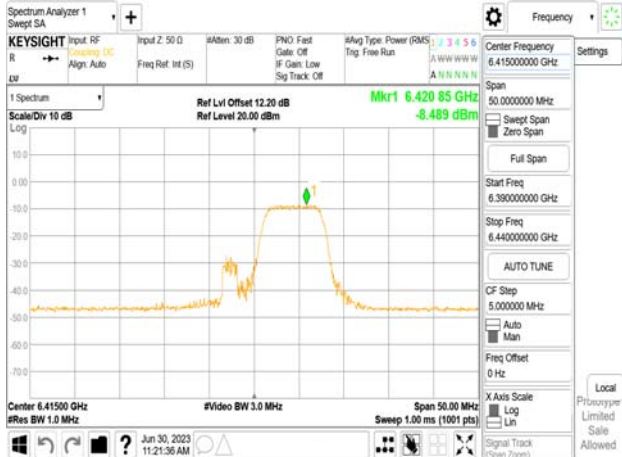
802.11be_20MHz_Chain1_6415MHz_52+26_MRU3
