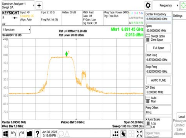
802.11be_20MHz_Chain1_6895MHz_RU26_0
