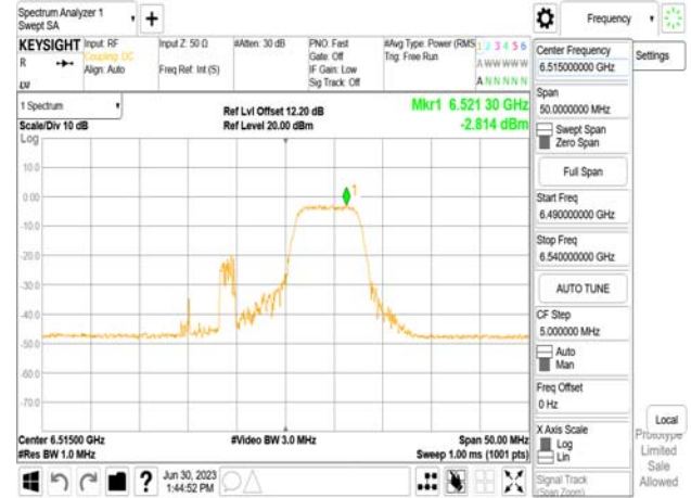
802.11be_20MHz_Chain0_6515MHz_RU106_54
