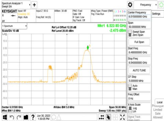
802.11be_20MHz_Chain0_6515MHz_RU52_40
