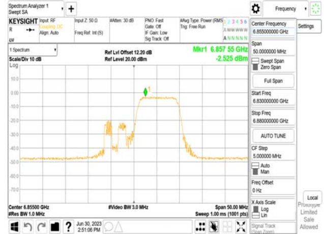
802.11be_20MHz_Chain1_6855MHz_RU106_54
