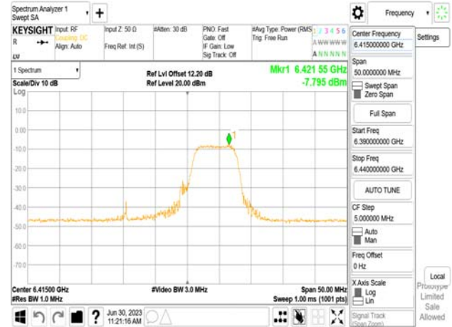
802.11be_20MHz_Chain0_6415MHz_RU106_54
