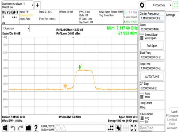
802.11be_20MHz_Chain1_7115MHz_RU106_54
