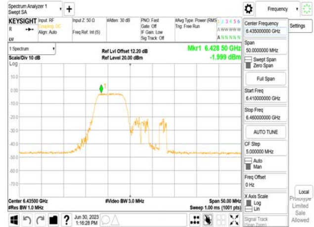
802.11be_20MHz_Chain0_6435MHz_RU106_53
