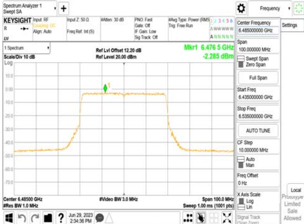
802.11be_40MHz_Chain0_6485MHz
