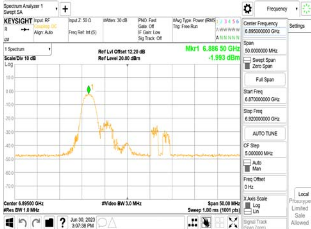
802.11be_20MHz_Chain0_6895MHz_RU26_0
