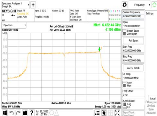
802.11ac_80MHz_Chain0_6385MHz
