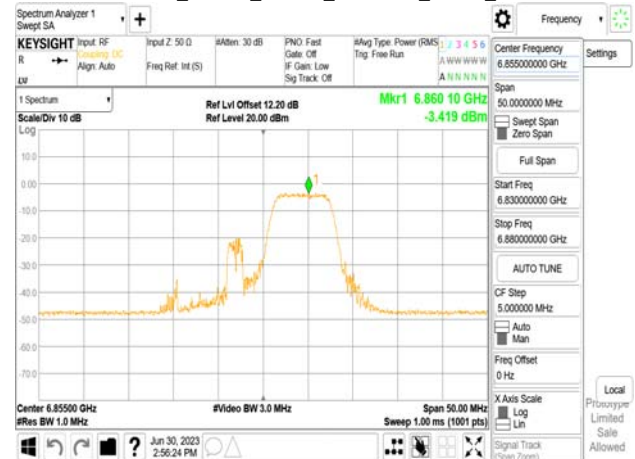
802.11be_20MHz_Chain0_6855MHz_52+26_MRU3
