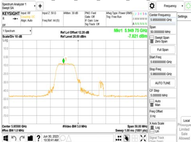
802.11be_20MHz_Chain0_5955MHz_52+26_MRU1
