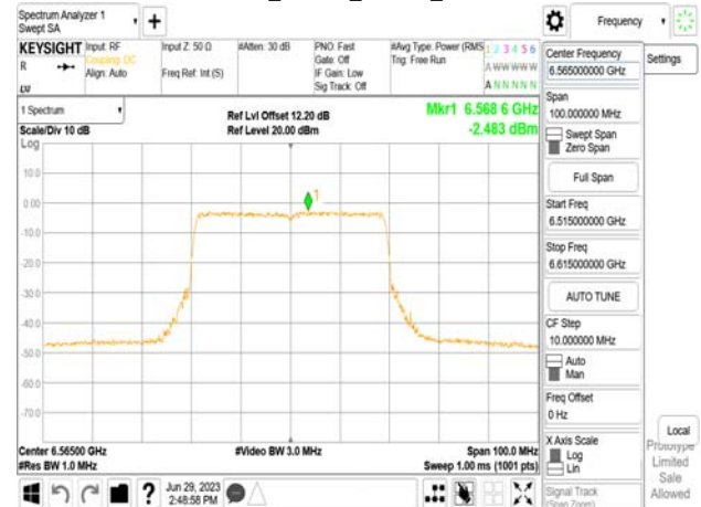
802.11be_40MHz_Chain1_6565MHz
