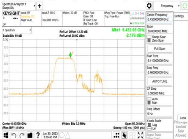
802.11be_20MHz_Chain1_6435MHz_52+26_MRU1
