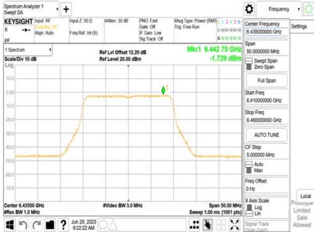
802.11be_20MHz_Chain1_6435MHz_106+26_MRU1
