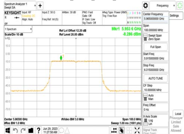
802.11be_40MHz_Chain1_5965MHz
