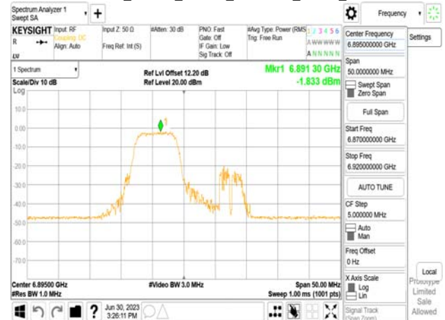
802.11be_20MHz_Chain1_6895MHz_52+26_MRU1
