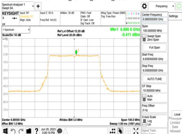
802.11be_40MHz_Chain1_6885MHz
