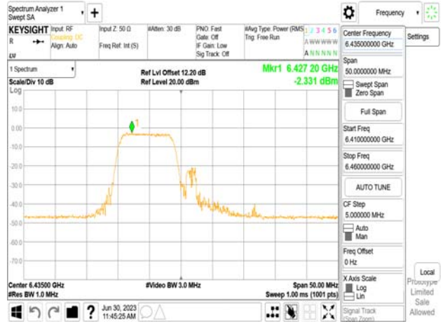
802.11be_20MHz_Chain1_6435MHz_RU26_0
