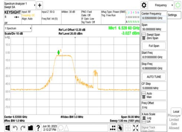
802.11be_20MHz_Chain1_6535MHz_RU106_53
