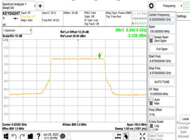
802.11be_40MHz_Chain0_6925MHz
