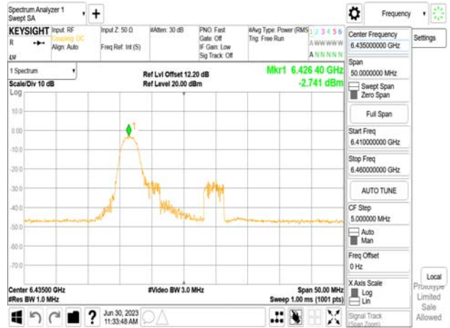
802.11be_20MHz_Chain1_6435MHz_RU52_37
