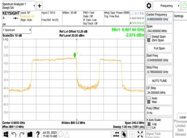
802.11be_160MHz_Chain1_6665MHz_RU996_67
