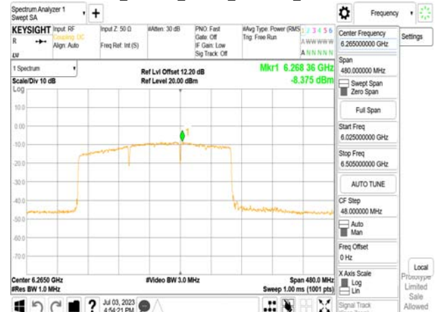
802.11be_320MHz_Chain0_6265MHz_3x996 MRU4
