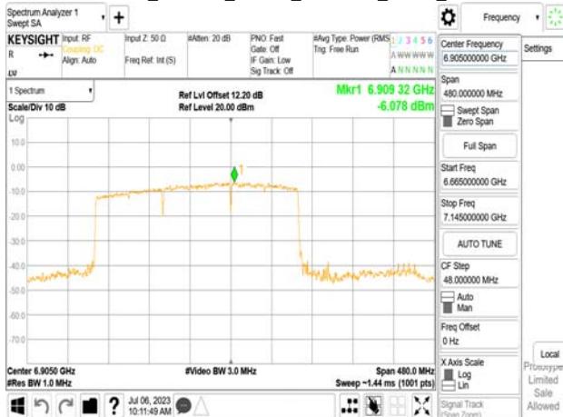
802.11be_320MHz_Chain1_6905MHz_3x996_MRU4
