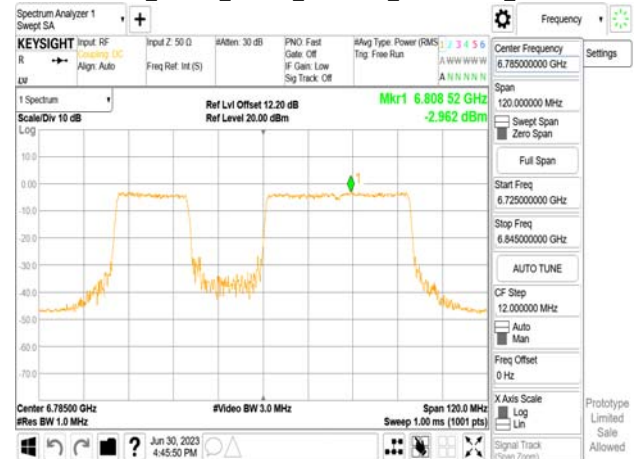
802.11be_80MHz_Chain1_6785MHz_RU484+242_Punc20
