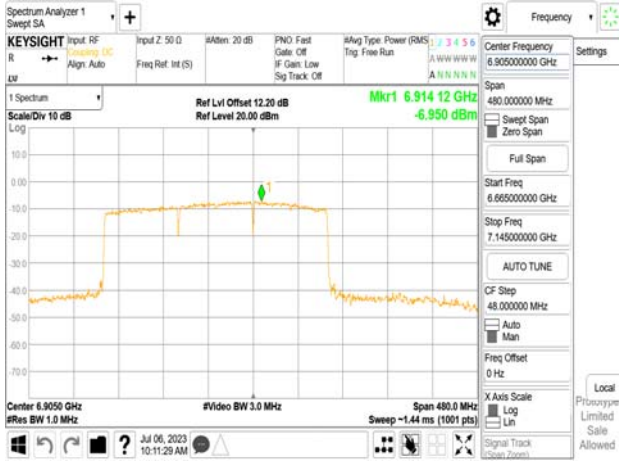
802.11be_320MHz_Chain0_6905MHz_3x996_MRU4
