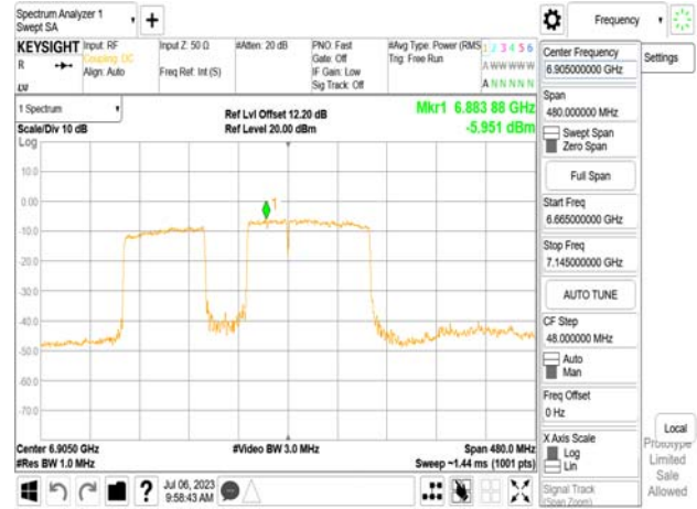
802.11be_320MHz_Chain1_6905MHz_RU996x2+484_Punc40
