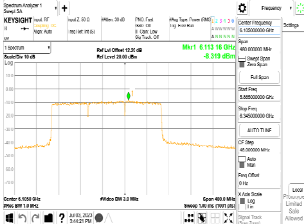
802.11be_320MHz_Chain0_6105MHz_3x996+484 MRU8
