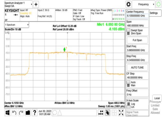
802.11be_320MHz_Chain1_6105MHz_2x996+484 MRU6
