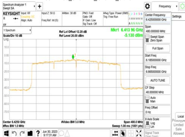
802.11be_320MHz_Chain1_6425MHz
