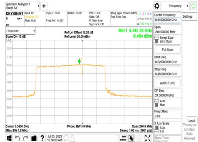
802.11be_160MHz_Chain0_6345MHz_RU996+484_Punc40
