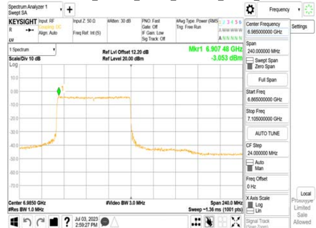
802.11be_160MHz_Chain0_6985MHz_RU996_67
