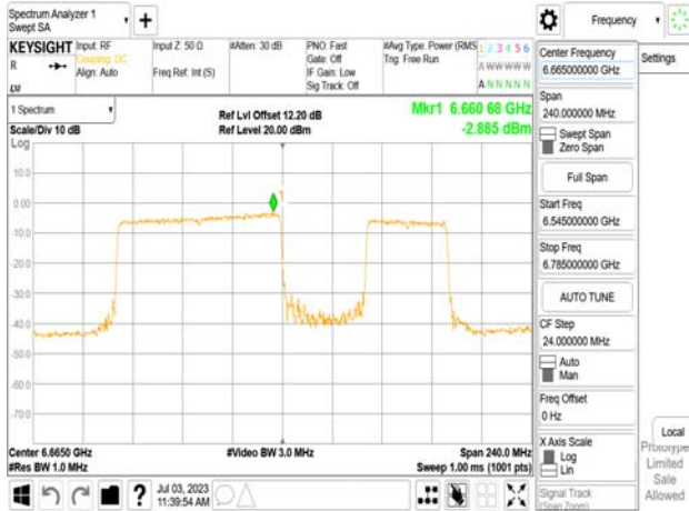
802.11be_160MHz_Chain0_6665MHz_RU996_67
