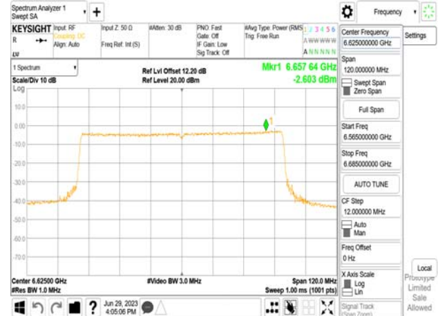
802.11be_80MHz_Chain0_6625MHz
