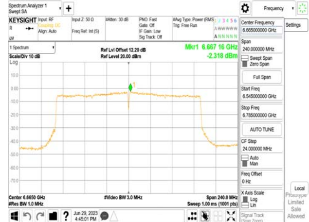
802.11be_160MHz_Chain1_6665MHz
