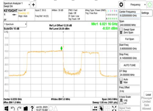
802.11be_160MHz_Chain1_6025MHz_RU996+484_Punct40
