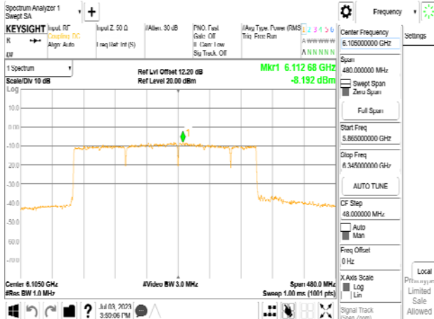
802.11be_320MHz_Chain0_6105MHz_RU996x2+484_Punc40
