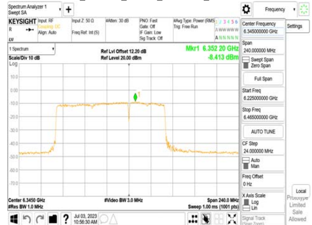
802.11be_160MHz_Chain1_6345MHz_996+484 MRU4
