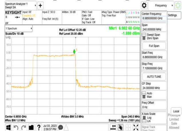
802.11be_160MHz_Chain1_6985MHz_RU996_67
