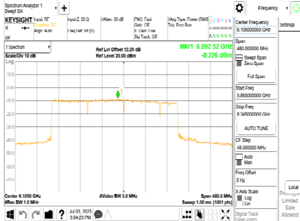
802.11be_320MHz_Chain1_6105MHz_RU996x2+484_Punc40
