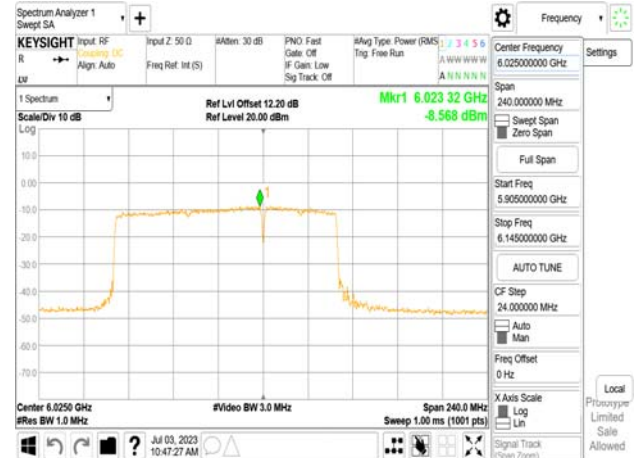
802.11be_160MHz_Chain0_6025MHz_RU996+484_Punc40
