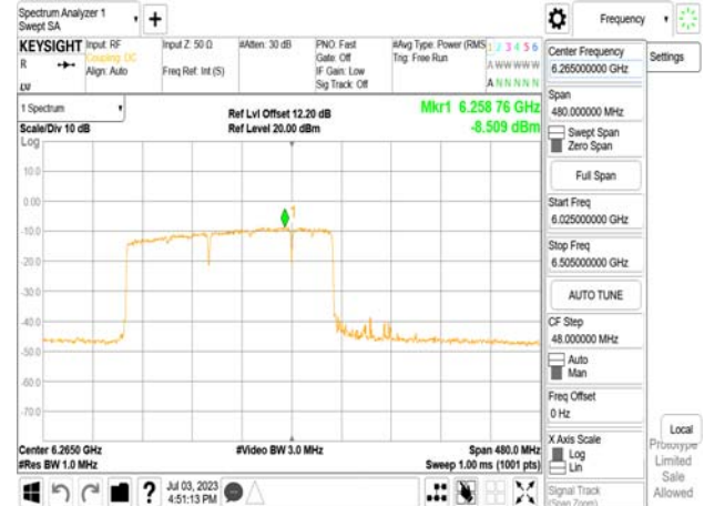
802.11be_320MHz_Chain1_6265MHz_3x996 MRU4
