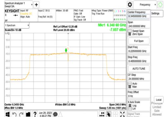
802.11be_160MHz_Chain0_6345MHz_996+484 MRU4
