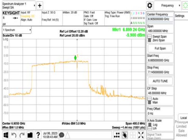
802.11be_320MHz_Chain1_6905MHz_3x996+484 MRU8
