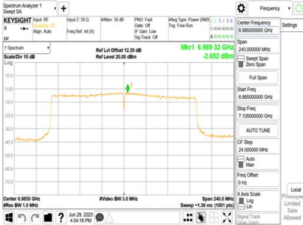
802.11be_160MHz_Chain0_6985MHz_996+484_MRU4
