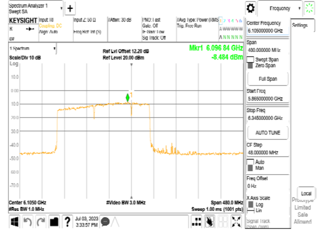
802.11be_320MHz_Chain1_6105MHz_2x996+484 MRU6
