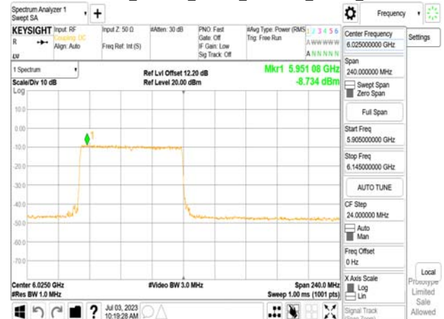
802.11be_160MHz_Chain0_6025MHz_RU996_67
