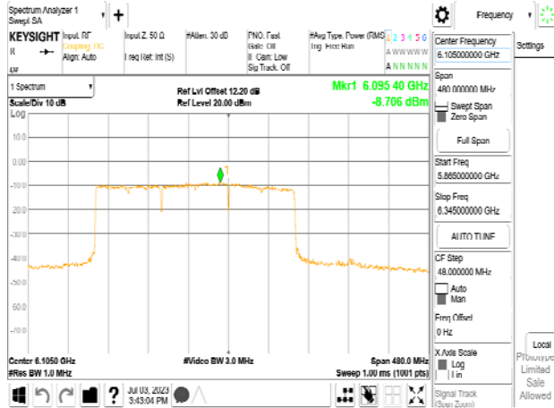
802.11be_320MHz_Chain1_6105MHz_3x996+484 MRU8
