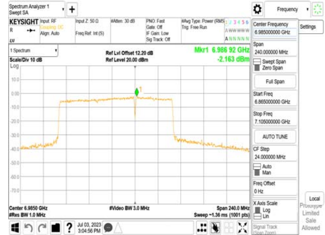
802.11be_160MHz_Chain1_6985MHz_RU996+484_Punc40
