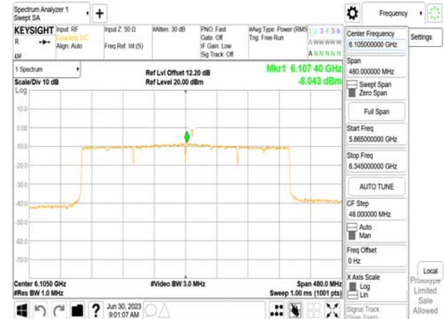
802.11be_320MHz_Chain0_6105MHz_2x996+484 MRU6
