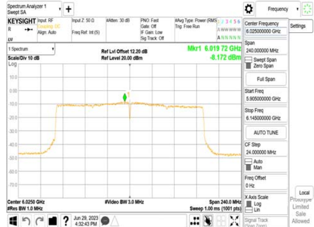
802.11be_160MHz_Chain1_6025MHz_996+484_MRU4
