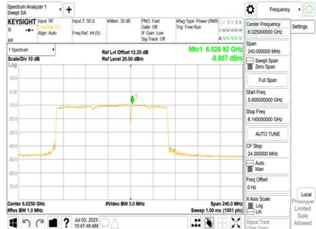
802.11be_160MHz_Chain1_6025MHz_RU996+484_Punct40
