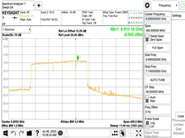
802.11be_320MHz_Chain0_6905MHz_3x996+484 MRU8
