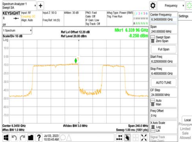
802.11be_160MHz_Chain1_6345MHz_RU996_67
