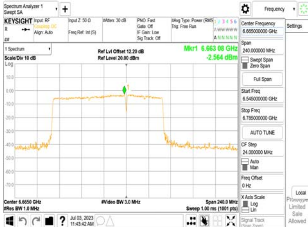
802.11be_160MHz_Chain1_6665MHz_RU996+484_Punc40
