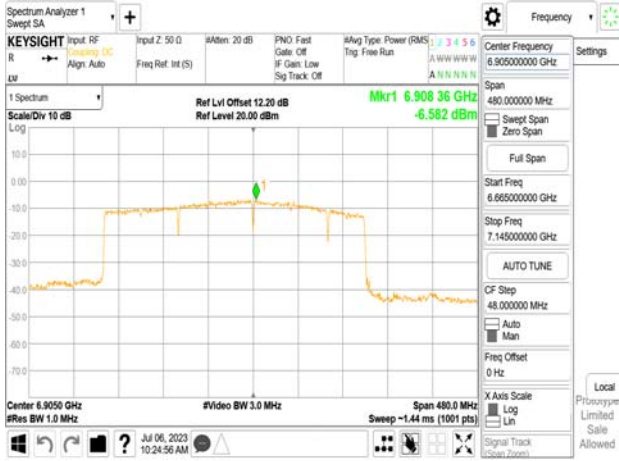
802.11be_320MHz_Chain0_6905MHz_3x996_MRU4
