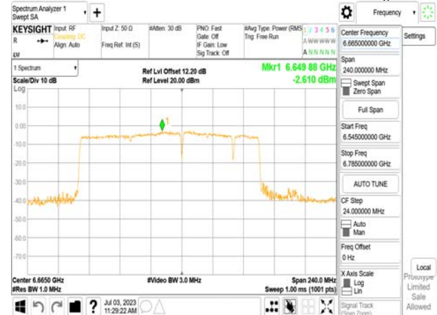
802.11be_160MHz_Chain1_6665MHz_SU_Punct20_Mid3
