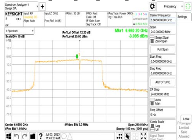
802.11be_160MHz_Chain0_6665MHz_996+484_MRU4
