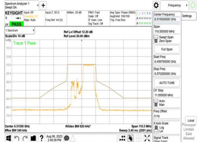
802.11be_20MHz_Chain0_6515MHz_RU106_54
