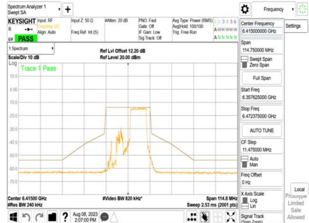
802.11be_20MHz_Chain0_6415MHz_RU26_8
