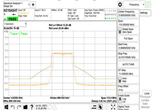
802.11be_20MHz_Chain1_5955MHz
