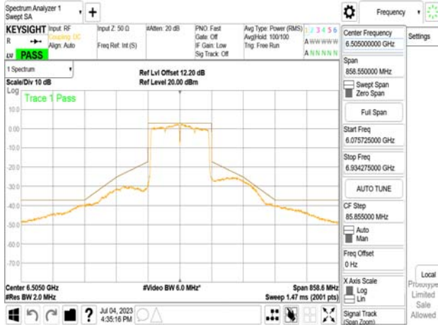
802.11ac_160MHz_Chain1_6505MHz
