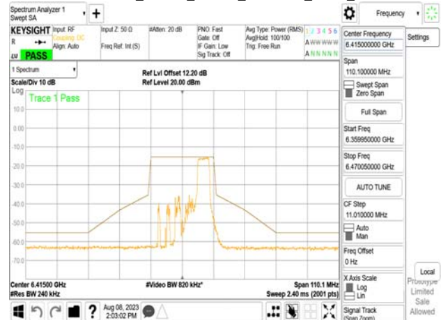
802.11be_20MHz_Chain1_6415MHz_RU52_40
