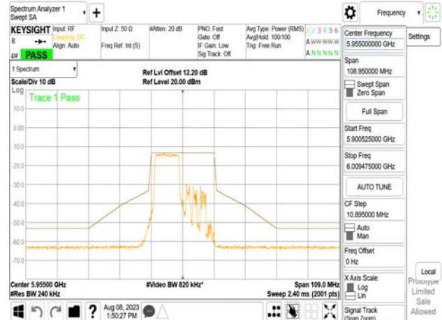
802.11be_20MHz_Chain0_5955MHz_RU26_0
