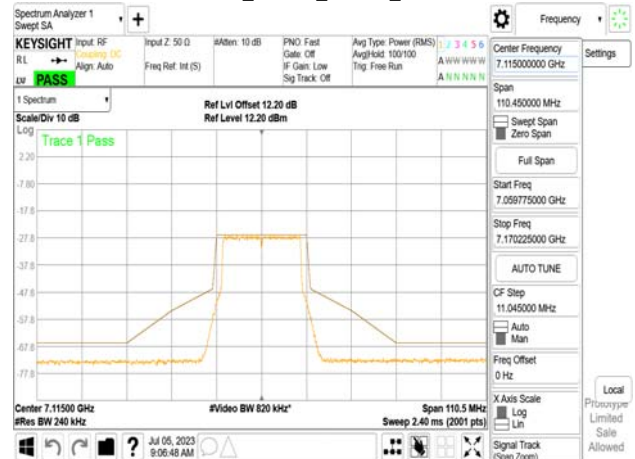
802.11be_20MHz_Chain0_7115MHz
