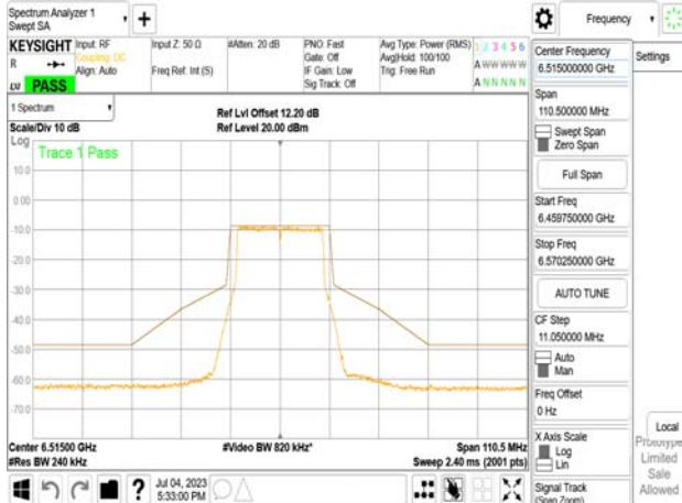
802.11be_20MHz_Chain0_6515MHz
