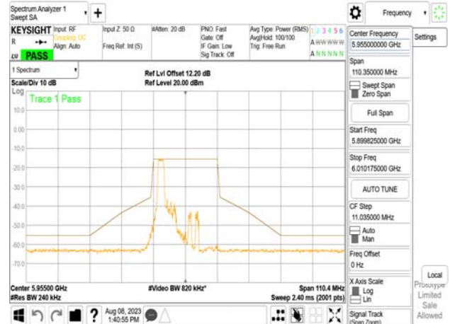
802.11be_20MHz_Chain1_5955MHz_RU52_37
