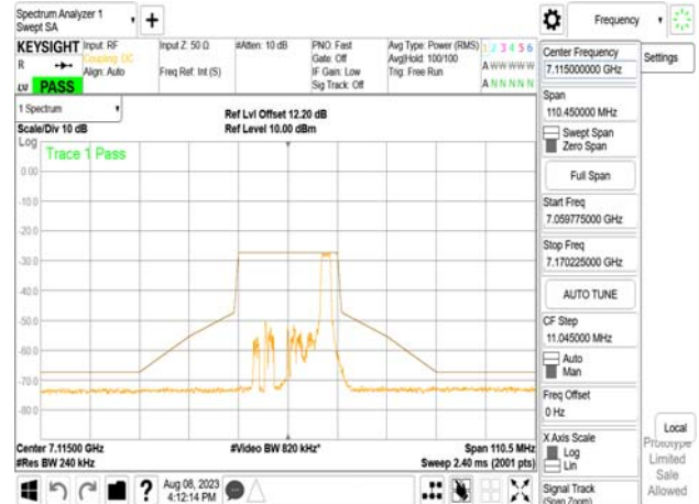
802.11be_20MHz_Chain0_7115MHz_RU52_40
