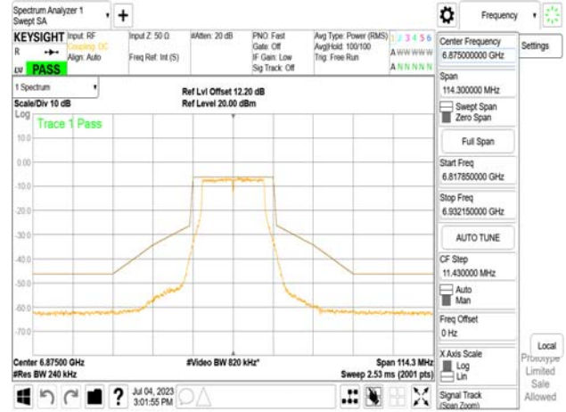
802.11n_20MHz_Chain0_6875MHz
