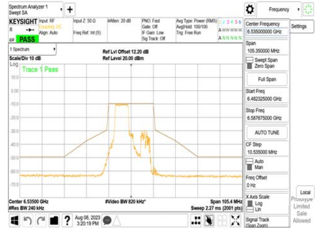
802.11be_20MHz_Chain0_6535MHz_RU106_53
