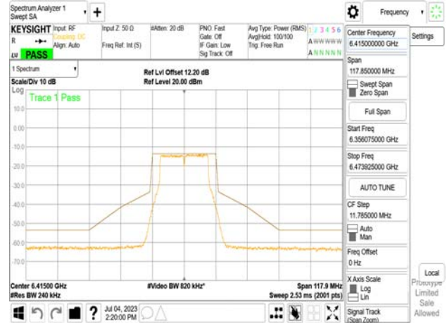
802.11n_20MHz_Chain1_6415MHz
