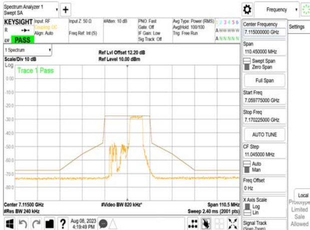
802.11be_20MHz_Chain0_7115MHz_RU106_54
