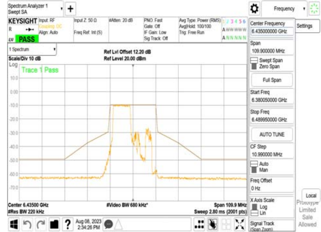
802.11be_20MHz_Chain0_6435MHz_RU26_0
