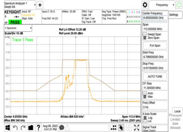
802.11be_20MHz_Chain0_6855MHz_52+26_MRU3
