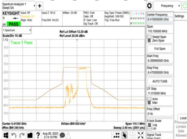
802.11be_20MHz_Chain1_6415MHz_52+26_MRU3
