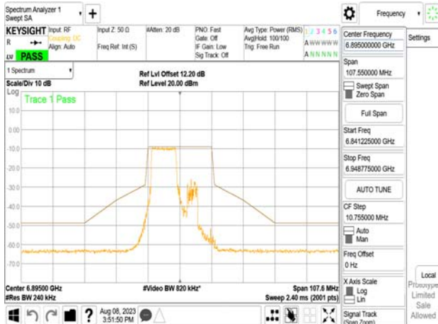
802.11be_20MHz_Chain0_6895MHz_RU26_0
