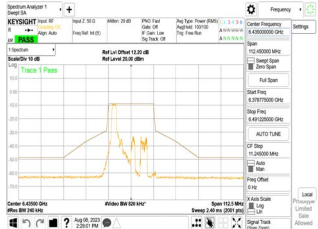
802.11be_20MHz_Chain1_6435MHz_RU52_37
