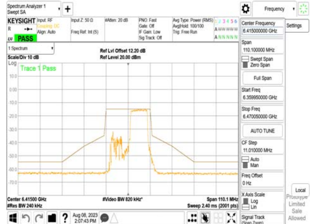
802.11be_20MHz_Chain1_6415MHz_RU26_8
