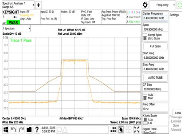
802.11be_20MHz_Chain0_6435MHz_106+26_MRU1
