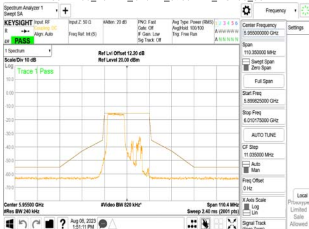
802.11be_20MHz_Chain1_5955MHz_RU106_53
