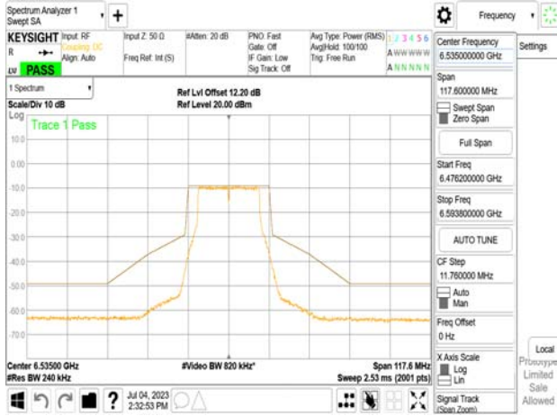
802.11n_20MHz_Chain0_6535MHz
