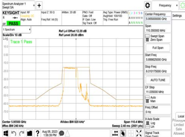
802.11be_20MHz_Chain1_5955MHz_52+26_MRU1
