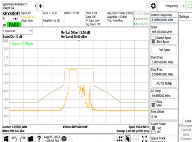
802.11be_20MHz_Chain0_5955MHz_52+26_MRU1
