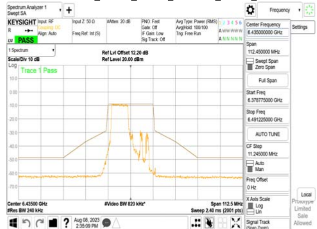
802.11be_20MHz_Chain1_6435MHz_RU26_0
