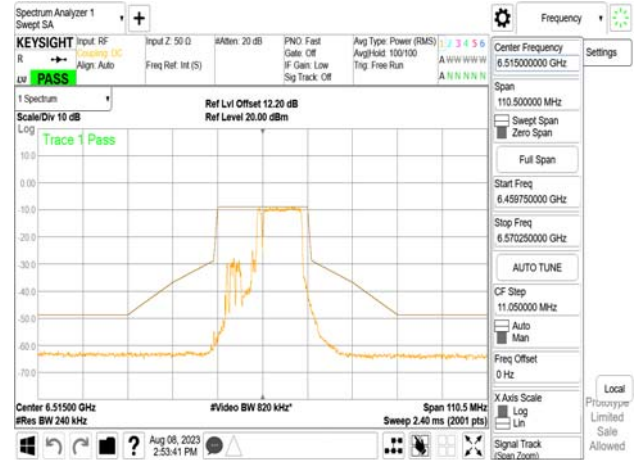
802.11be_20MHz_Chain0_6515MHz_52+26_MRU3
