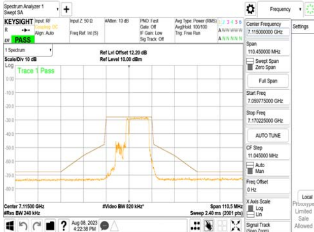
802.11be_20MHz_Chain0_7115MHz_52+26_MRU3
