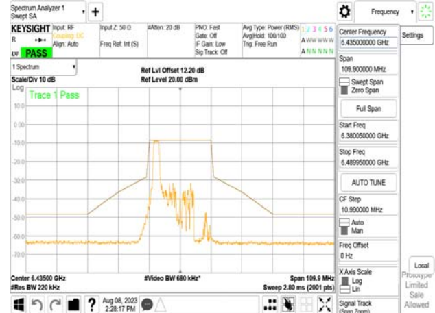
802.11be_20MHz_Chain0_6435MHz_RU26_0
