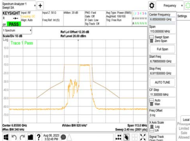
802.11be_20MHz_Chain0_6855MHz_RU26_8
