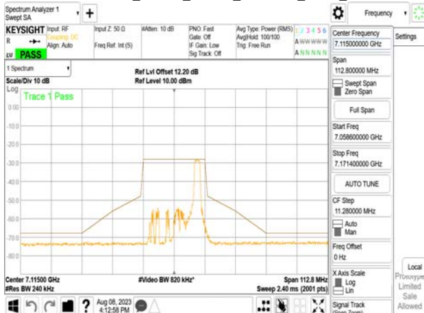
802.11be_20MHz_Chain1_7115MHz_RU26_8
