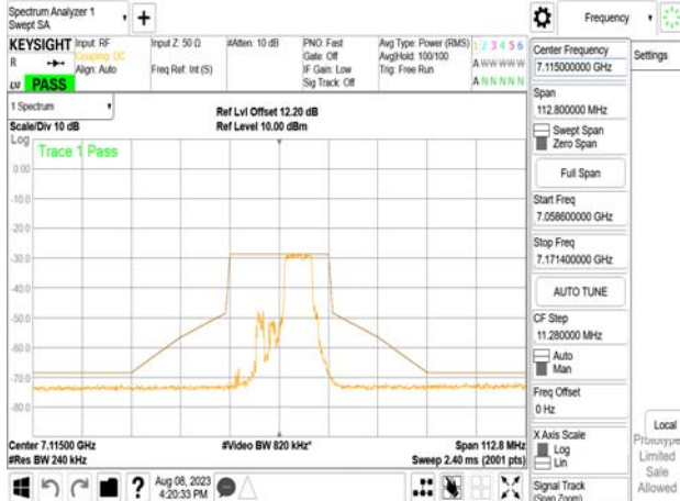
802.11be_20MHz_Chain1_7115MHz_RU106_54
