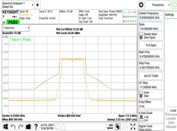
802.11be_20MHz_Chain1_6535MHz_106+26_MRU1
