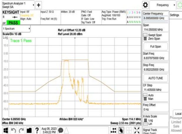
802.11be_20MHz_Chain1_6895MHz_RU52_37
