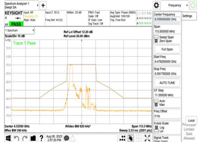
802.11be_20MHz_Chain1_6535MHz_RU26_0
