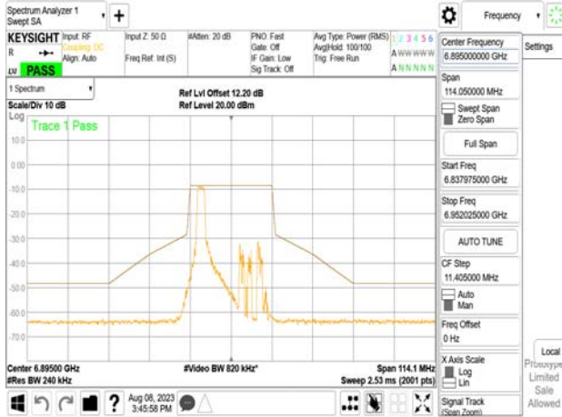
802.11be_20MHz_Chain1_6895MHz_RU52_37
