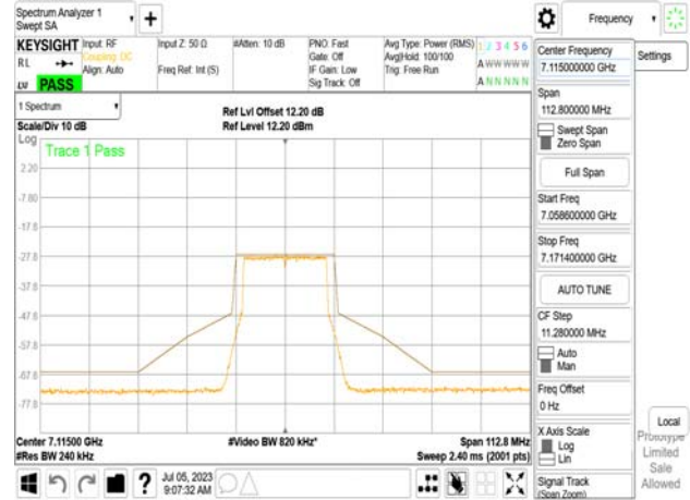
802.11be_20MHz_Chain1_7115MHz_106+26_MRU2
