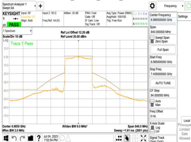
802.11be_160MHz_Chain1_6985MHz
