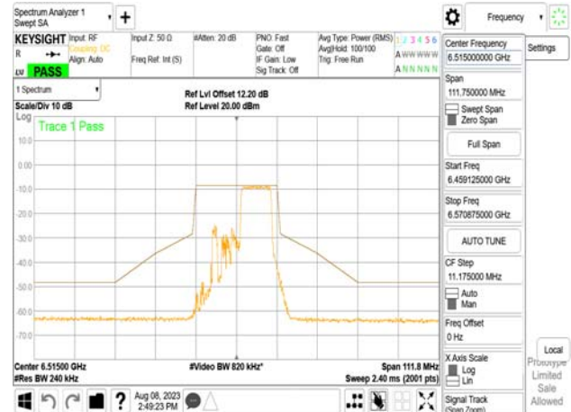
802.11be_20MHz_Chain1_6515MHz_RU26_8
