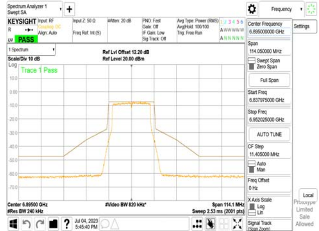
802.11be_20MHz_Chain1_6895MHz_106+26_MRU1
