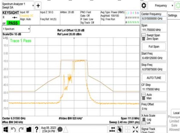
802.11be_20MHz_Chain1_6515MHz_106+26_MRUC
