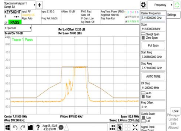
802.11be_20MHz_Chain1_7115MHz_106+26_MRU2
