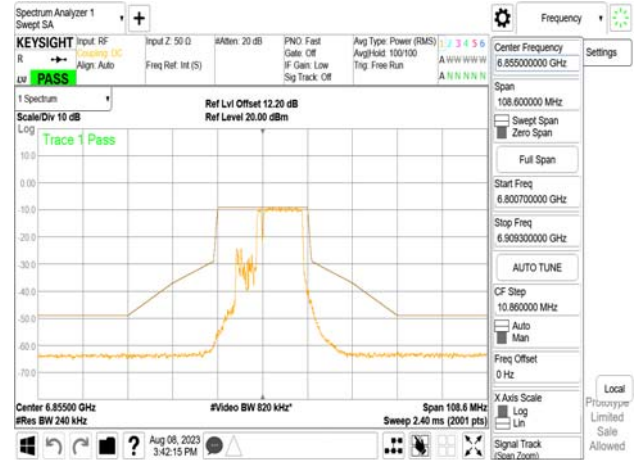
802.11be_20MHz_Chain1_6855MHz_52+26_MRU3
