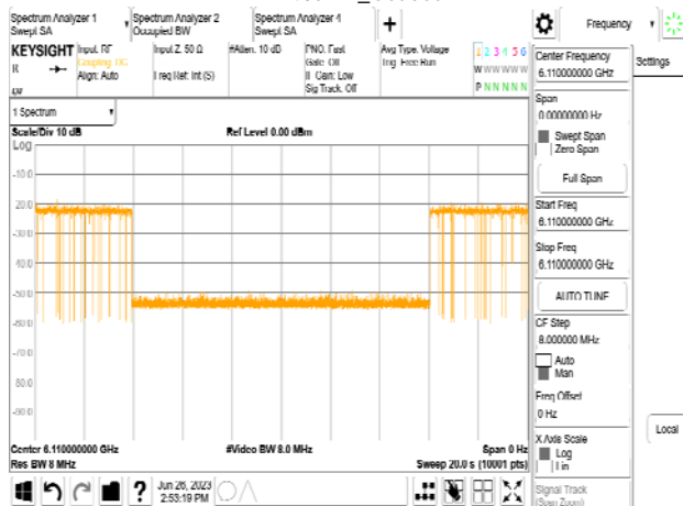
802.11be_320MHz_CF 6265MHz_Interference_6110MHz_-73.48dBm_Minimal
