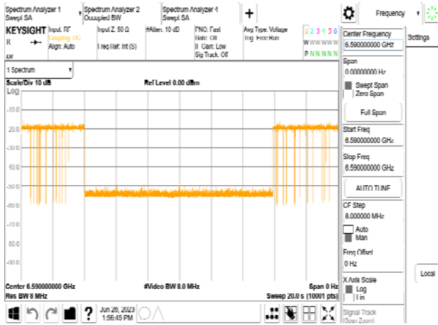
802.11be_320MHz_CF 6745MHz_Interference_6590MHz_-76.36dBm_Minimal
