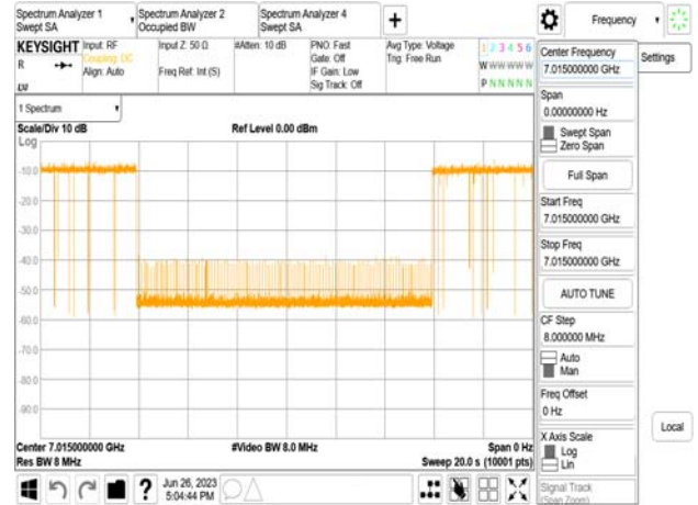
802.11be_20MHz_CF 7015MHz_Interference_7015MHz_-74.75dBm_Minimal
