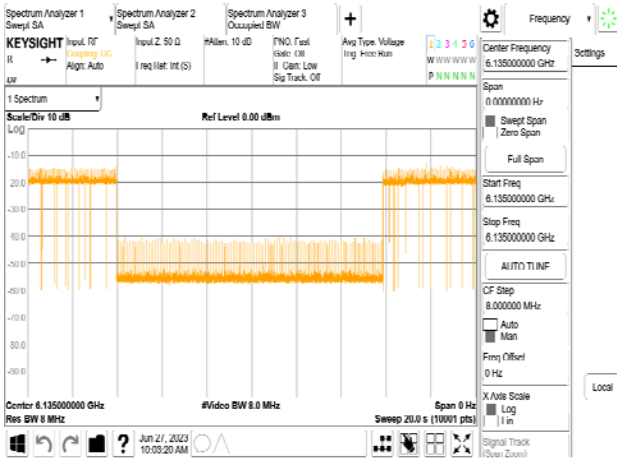
802.11be_20MHz_CF 6135MHz_Interference_6135MHz_-75.25dBm_Minimal
