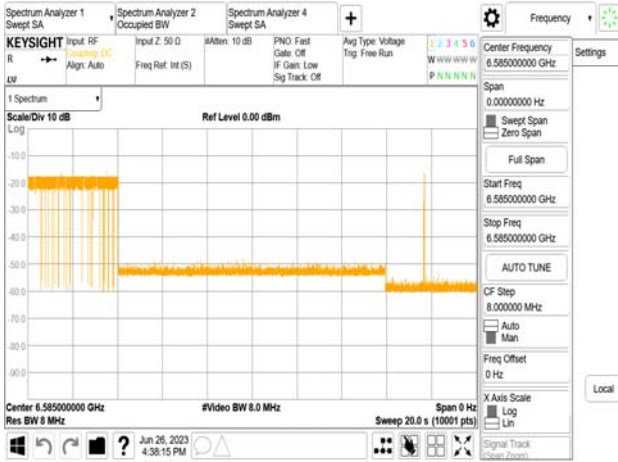
802.11be_320MHz_CF 6585MHz_Interference_6585MHz_-71.32dBm_Minimal
