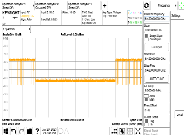
802.11be_320MHz_CF 6265MHz_Interference_6420MHz_-74.28dBm_Minimal
