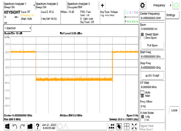
802.11be_20MHz_CF 6455MHz_Interference_6455MHz_-76.49dBm_Minimal
