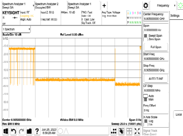
802.11be_320MHz_CF 6905MHz_Interference_6905MHz_-71.76dBm_Minimal
