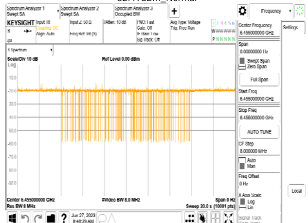
802.11be_20MHz_CF 6455MHz_Interference_6455MHz_-82.49dBm_Normal
