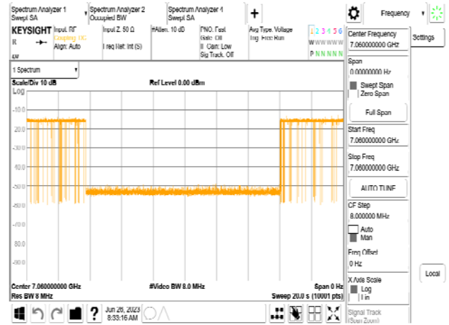
802.11be_320MHz_CF 6905MHz_Interference_7060MHz_-74.96dBm_Minimal
