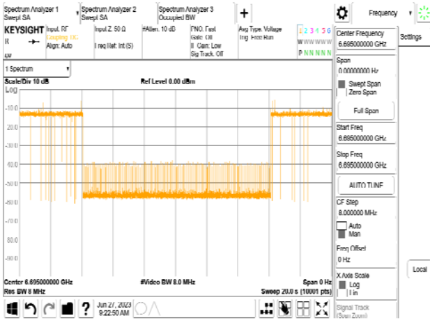
802.11be_20MHz_CF 6695MHz_Interference_6695MHz_-78.47dBm_Minimal
