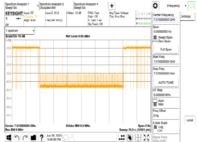
802.11be_20MHz_CF 7015MHz_Interference_7015MHz_-79.75dBm_Normal
