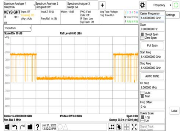
802.11be_320MHz_CF 6585MHz_Interference_6430MHz_-76.43dBm_Minimal
