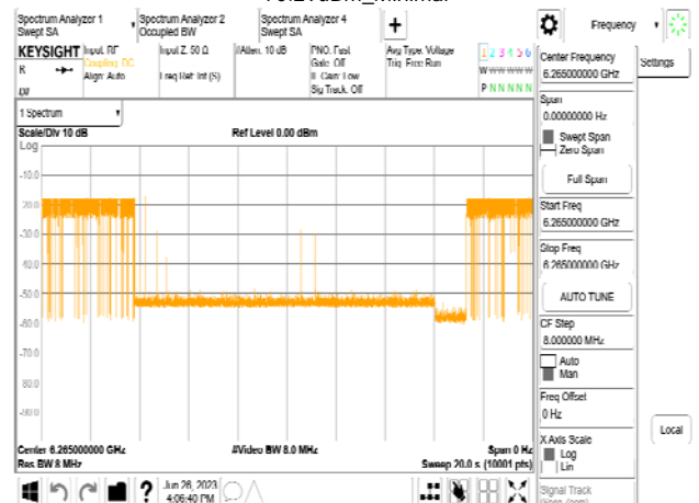
802.11be_320MHz_CF 6265MHz_Interference_6265MHz_-81.29dBm_Normal
