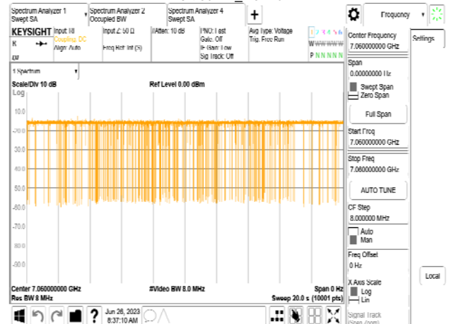
802.11be_320MHz_CF 6905MHz_Interference_7060MHz_-78.96dBm_Normal
