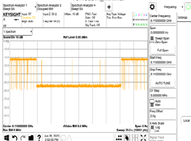
802.11be_320MHz_CF 6265MHz_Interference_6110MHz_-76.48dBm_Normal
