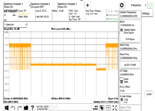
802.11be_320MHz_CF 6265MHz_Interference_6265MHz_-70.29dBm_Minimal
