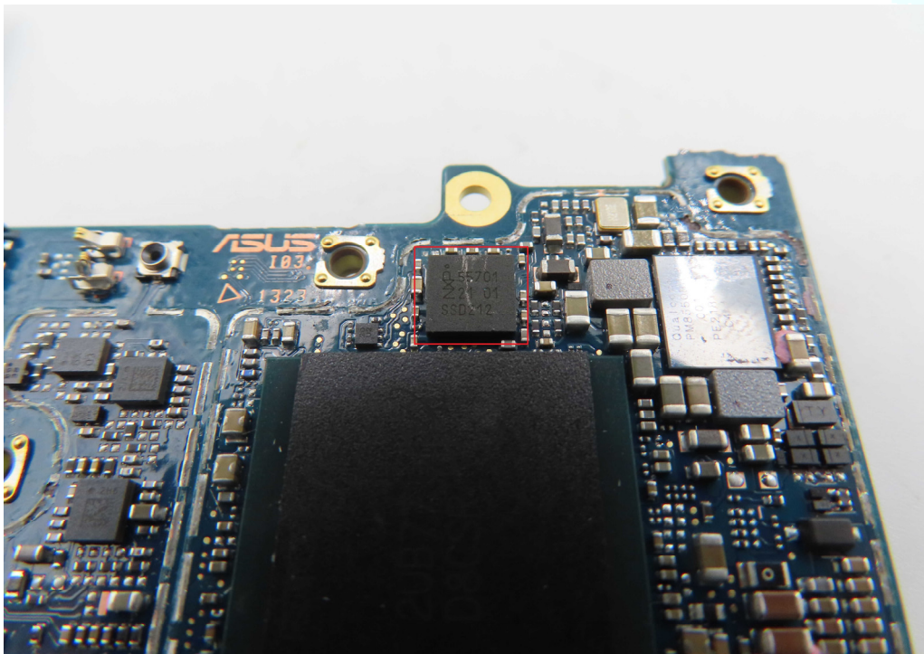
NFC Module
