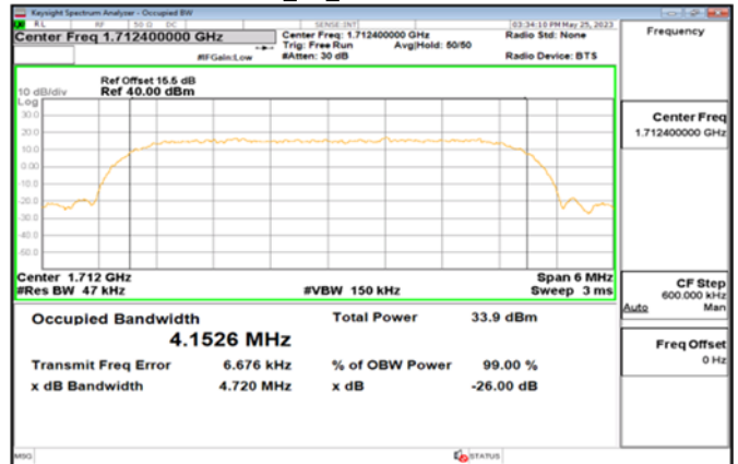
WCDMA_B4_LowCH1312-1712.4
