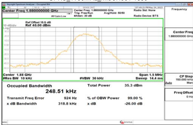
GPRS_1900MHz_MidCH661-1880
