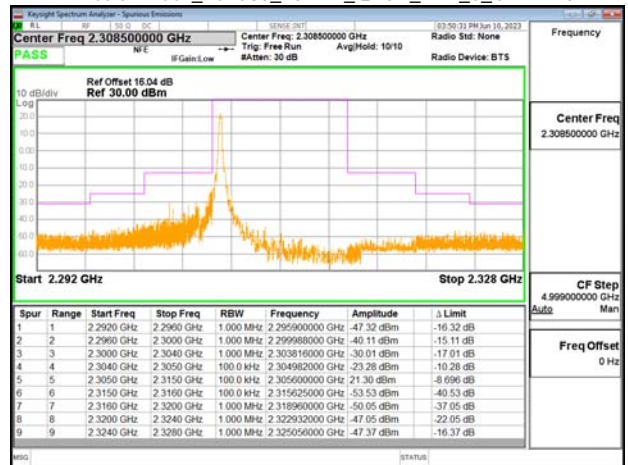
Emission Mask_Band30_10MHz_QPSK_RB1_49_CH27710
