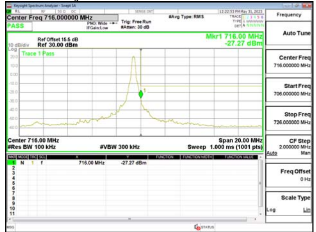
Band Edge_Band17_10MHz_QPSK_RB1_49_CH23800
