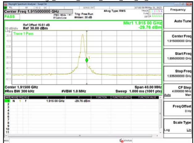
Band Edge_Band25_20MHz_QPSK_RB1_99_CH26590
