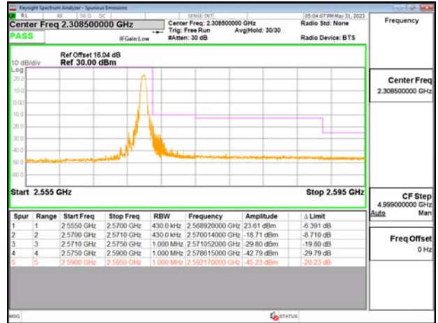
Emission Mask_Band7_20MHz_QPSK_RB1_99_CH21350
