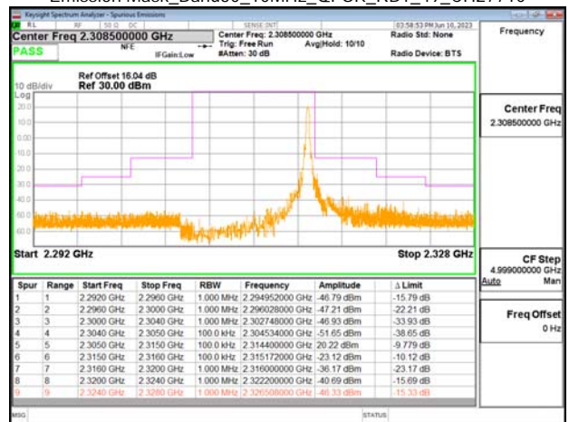
Emission Mask_Band30_10MHz_QPSK_RB1_49_CH27710
