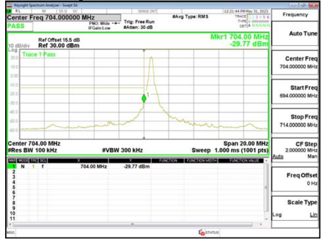
Band Edge_Band17_10MHz_QPSK_RB1_49_CH23800
