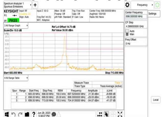
Band71_15MHz_DFT_s_OFDM_SCS15kHz_BPSK_RB1_78_CH138100
