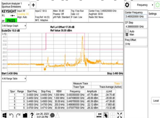
Band77-Part27_20MHz_DFT_s_OFDM_SCS30kHz_BPSK_RB1_50_CH630668
