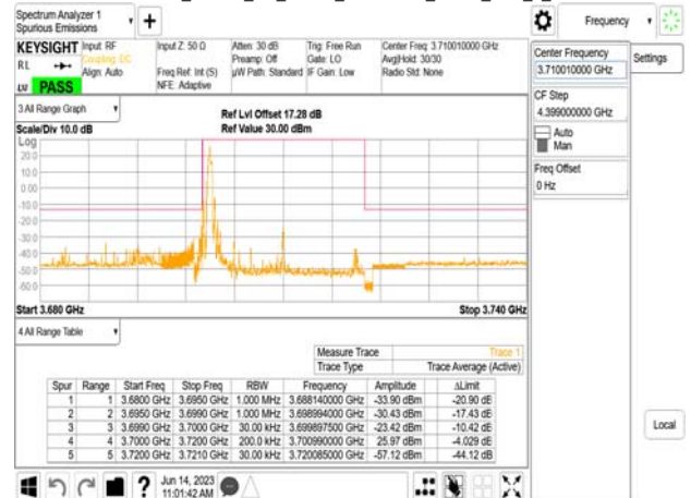
Band77-Part27_20MHz_CP_OFDM_SCS30kHz_QPSK_RB1_0_CH647334
