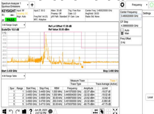
Band77-Part27_20MHz_CP_OFDM_SCS30kHz_QPSK_RB1_0_CH630668
