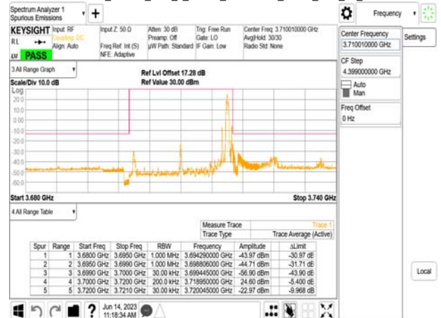
Band77-Part27_20MHz_DFT_s_OFDM_SCS30kHz_BPSK_RB1_50_CH647334
