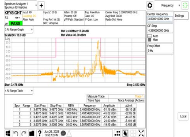
Band77-Part27_15MHz_CP_OFDM_SCS30kHz_QPSK_RB1_37_CH63166
