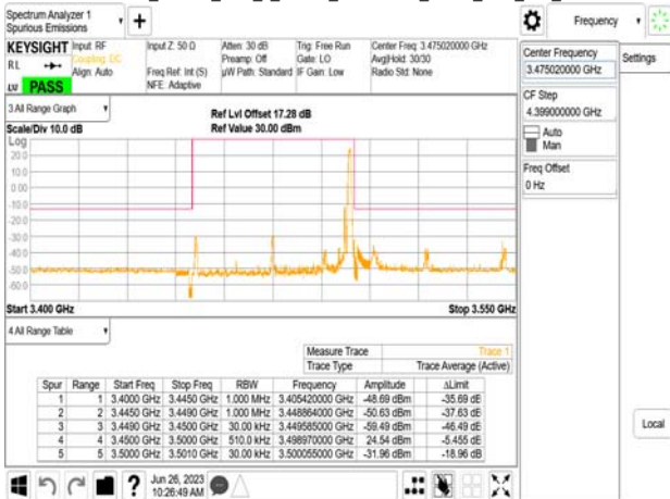
Band77-Part27_50MHz_DFT_s_OFDM_SCS30kHz_BPSK_RB1_132_CH631668
