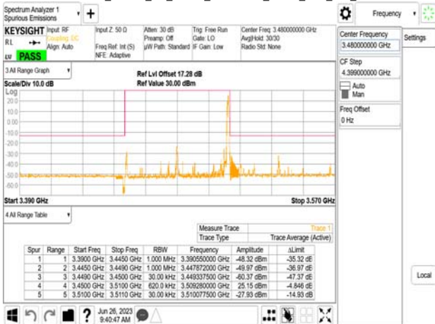
Band77-Part27_60MHz_CP_OFDM_SCS30kHz_QPSK_RB1_161_CH632000
