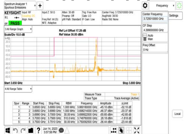
Band77-Part27_50MHz_CP_OFDM_SCS30kHz_QPSK_RB1_132_CH648334
