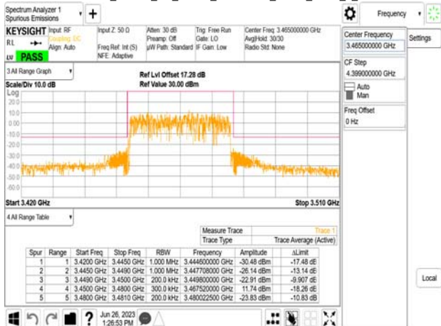
Band77-Part27_30MHz_CP_OFDM_SCS30kHz_QPSK_RB78_0_CH631000
