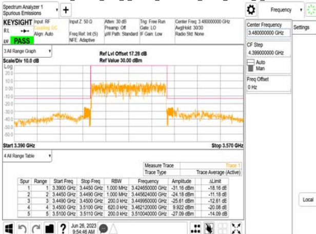
Band77-Part27_60MHz_DFT_s_OFDM_SCS30kHz_BPSK_RB162_0_CH632000
