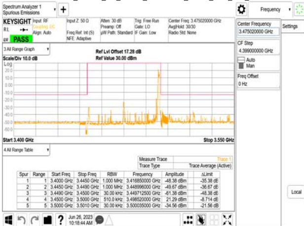
Band77-Part27_50MHz_CP_OFDM_SCS30kHz_QPSK_RB1_132_CH631668
