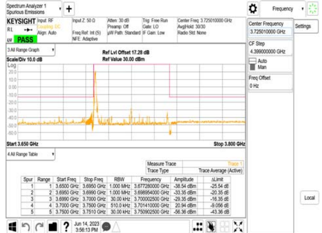
Band77-Part27_50MHz_CP_OFDM_SCS30kHz_QPSK_RB1_0_CH648334
