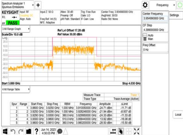
Band77-Part27_50MHz_CP_OFDM_SCS30kHz_QPSK_RB1_0_CH61668
