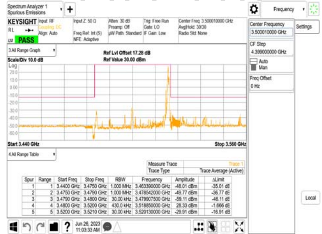
Band77-Part27_40MHz_CP_OFDM_SCS30kHz_QPSK_RB1_105_CH635332
