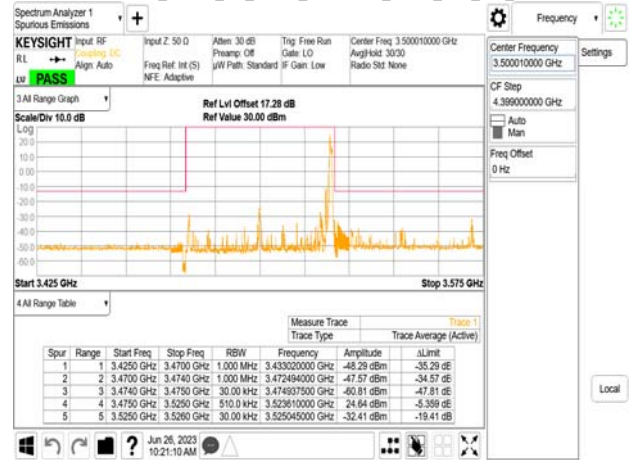
Band77-Part27_50MHz_CP_OFDM_SCS30kHz_QPSK_RB1_132_CH635000
