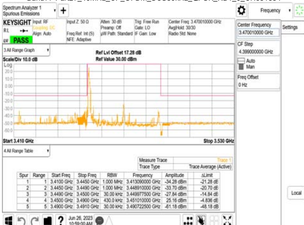
Band77-Part27_40MHz_CP_OFDM_SCS30kHz_QPSK_RB1_0_CH631334
