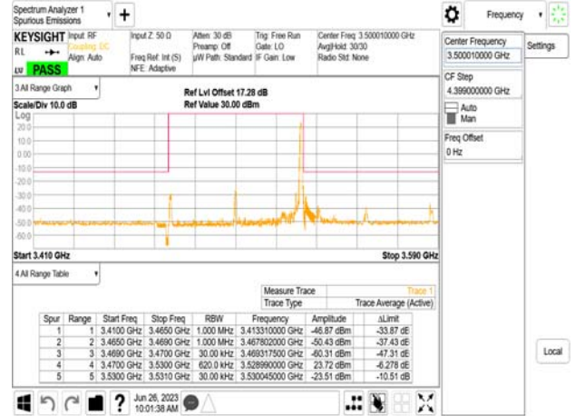
Band77-Part27_60MHz_DFT_s_OFDM_SCS30kHz_BPSK_RB1_161_CH634666
