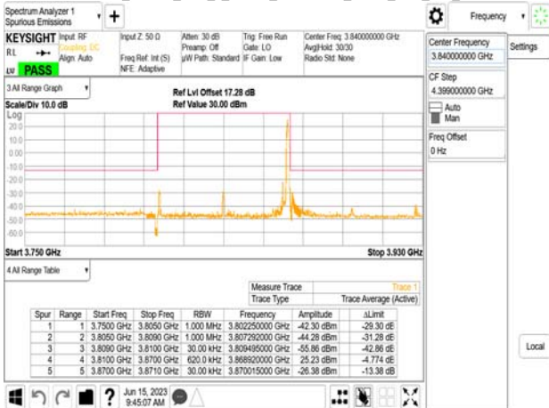
Band77-Part27_60MHz_DFT_s_OFDM_SCS30kHz_BPSK_RB1_161_CH663332
