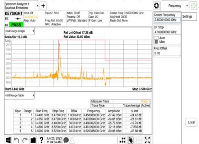
Band77-Part27_40MHz_CP_OFDM_SCS30kHz_QPSK_RB1_0_CH635332
