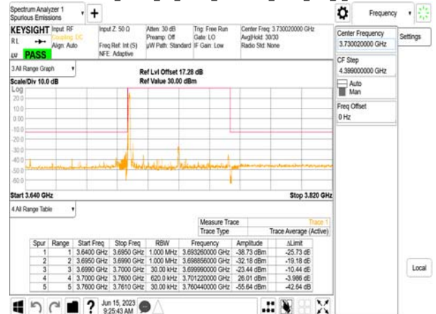
Band77-Part27_60MHz_CP_OFDM_SCS30kHz_QPSK_RB1_0_CH648668
