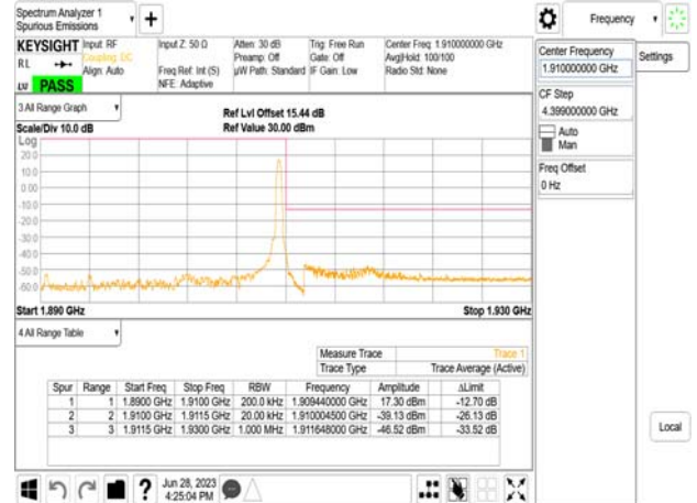
Band2_20MHz_CP_OFDM_SCS15kHz_QPSK_RB1_105_CH380000
