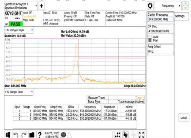
Band5_15MHz_CP_OFDM_SCS15kHz_QPSK_RB1_78_CH168300
