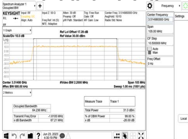
Band77-Part27_70MHz_DFT_s_OFDM_SCS30kHz_QPSK_RB180_0_CH634332
