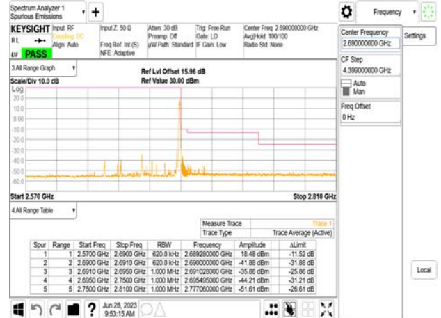
Band41_60MHz_CP_OFDM_SCS30kHz_QPSK_RB1_161_CH531996
