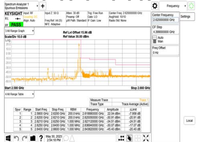
Band38_20MHz_CP_OFDM_SCS30kHz_QPSK_RB1_50_CH522000
