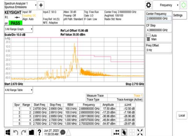
Band41_10MHz_CP_OFDM_SCS30kHz_QPSK_RB1_23_CH537000
