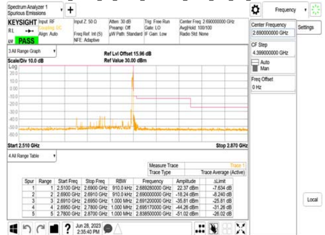
Band41_90MHz_CP_OFDM_SCS30kHz_QPSK_RB1_244_CH528996
