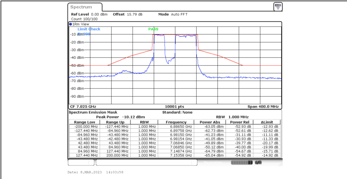
11BE80MIMO_Ant4_7025_Large RU 484+242_4
