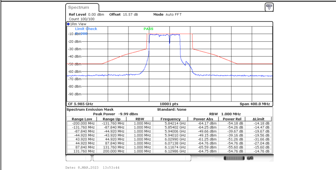
11BE80MIMO_Ant4_5985_Puncturing 20M_1
