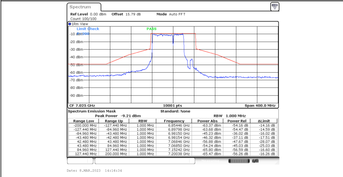
11BE80MIMO_Ant4_7025_Puncturing 20M_1
