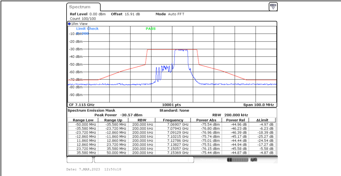
11BE20MIMO_Ant4_7115_106+26_OFDMA_2
