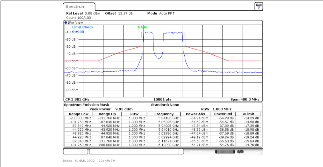
11BE80MIMO_Ant4_5985_Large RU 484+242_4
