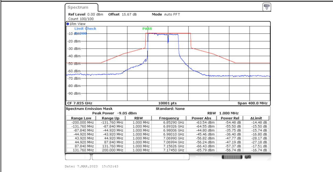
11BE80MIMO_Ant4_7025_Large RU 484+242_2
