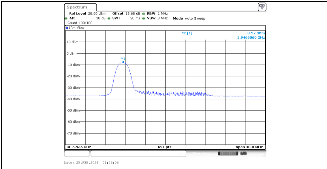
11BE20MIMO_Ant5_5955_52Tone_RU37
