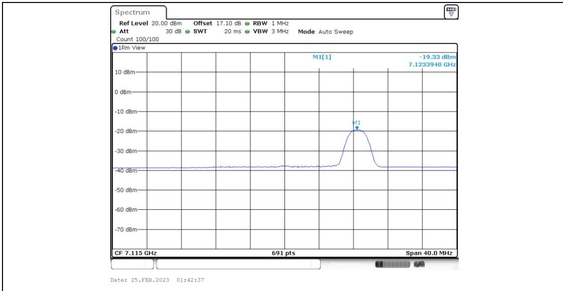
11BE20MIMO_Ant5_7115_52Tone_RU40
