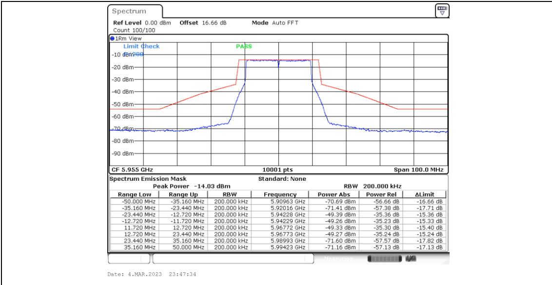
11B20MIMO_Ant2_5955
