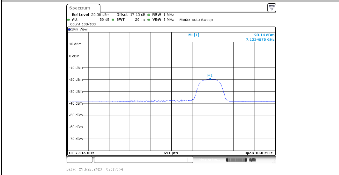
11BE20MIMO_Ant5_7115_106Tone_RU54
