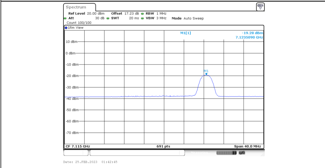
11BE20MIMO_Ant6_7115_52Tone_RU40
