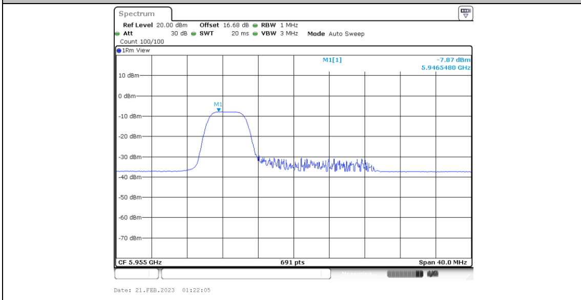
11BE20MIMO_Ant5_5955_106Tone_RU53
