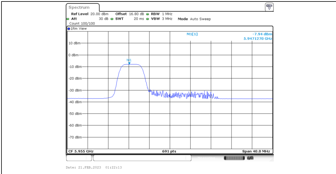
11BE20MIMO_Ant6_5955_106Tone_RU53
