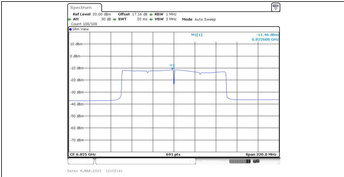
11BE160MIMO_Ant2_6825
