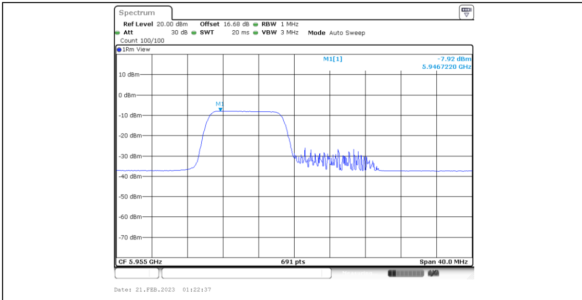
11BE20MIMO_Ant6_5955_26Tone_RU0
