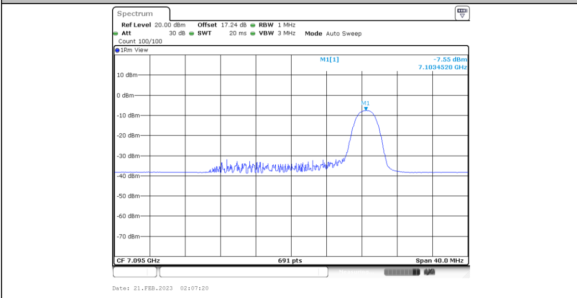
11BE20MIMO_Ant6_7095_52Tone_RU40
