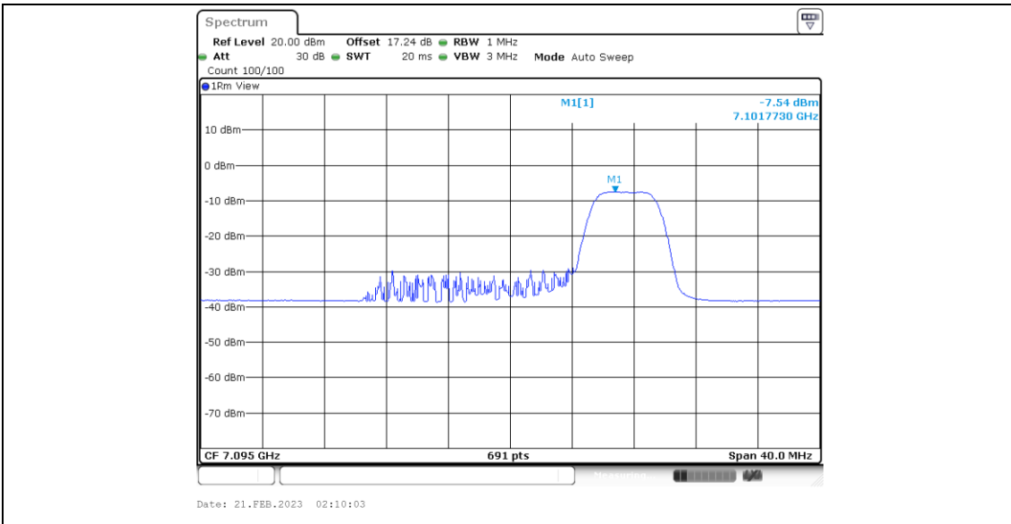
11BE20MIMO_Ant6_7095_106Tone_RU54
