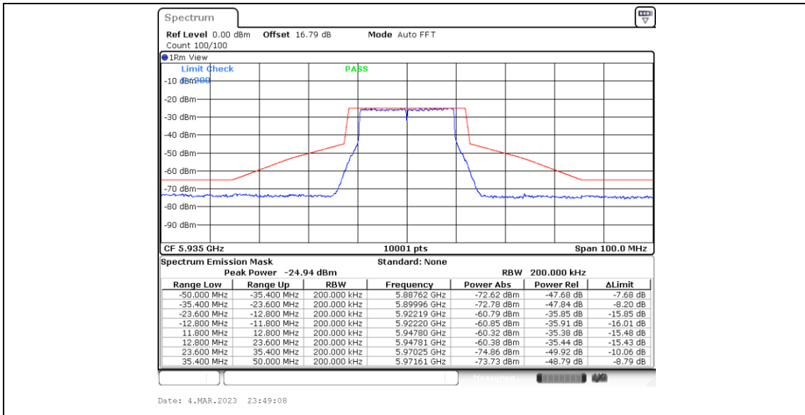
11BE20MIMO_Ant2_5935
