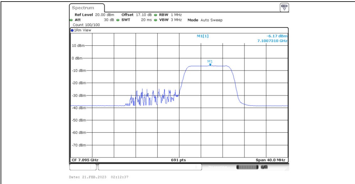
11BE20MIMO_Ant6_7095_26Tone_RU8
