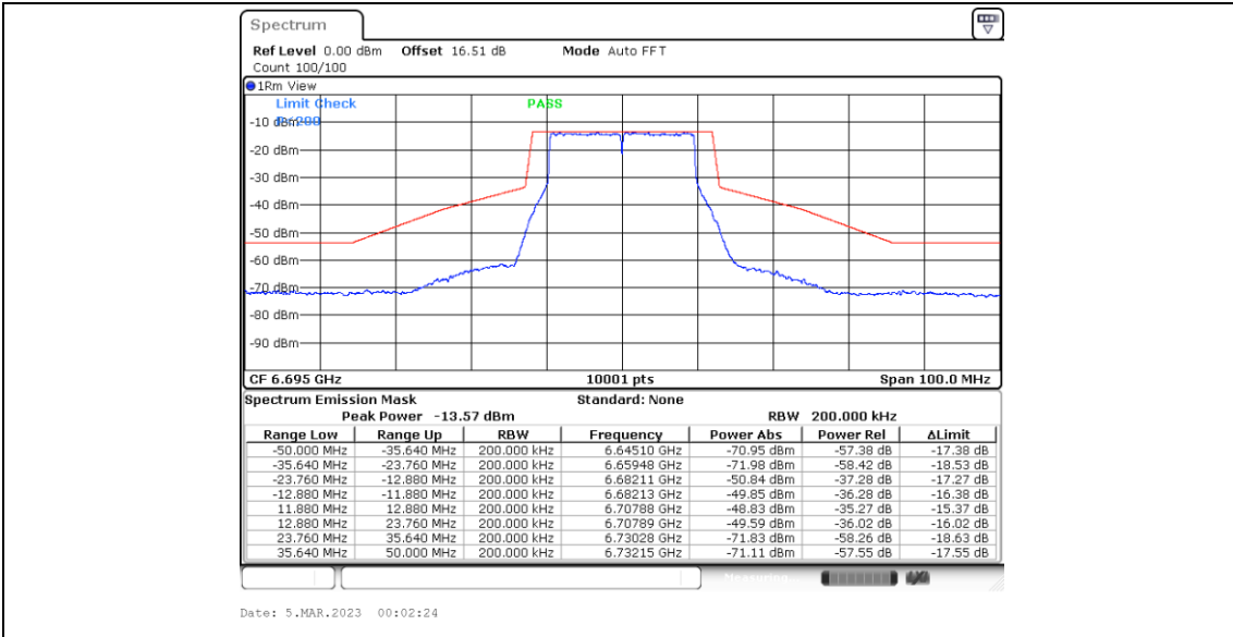
11BE20MIMO_Ant6_6695
