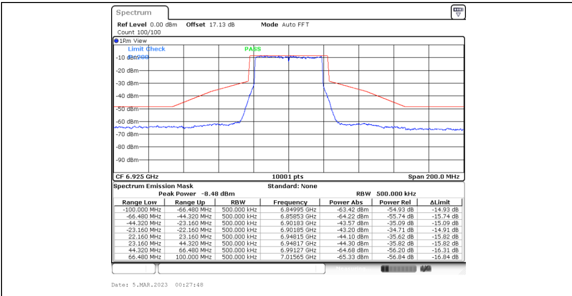
11BE40MIMO_Ant6_6925
