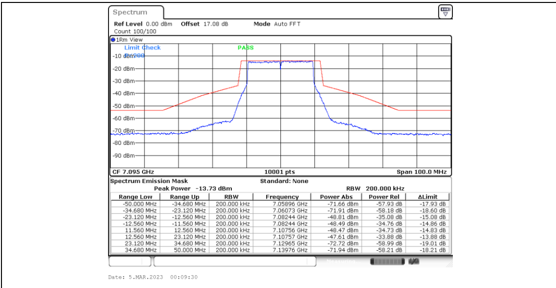
11B20MIMO_Ant6_7095
