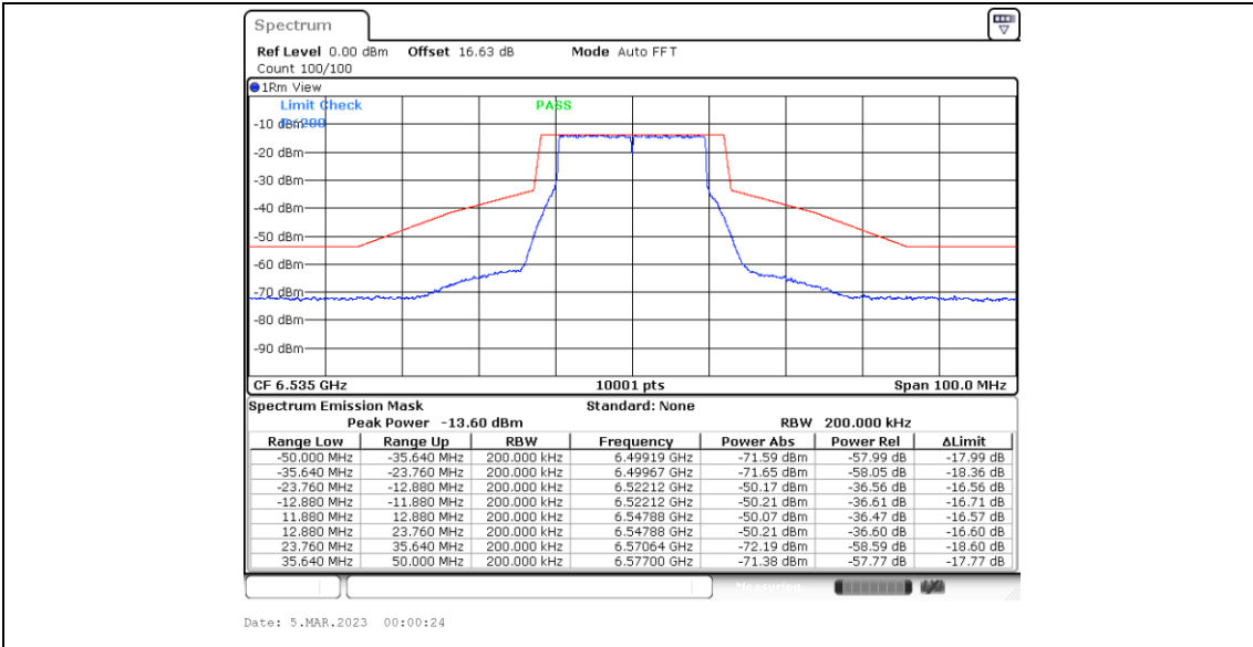
11BE20MIMO_Ant6_6535
