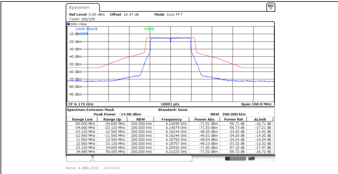
11BE20MIMO_Ant6_6175
