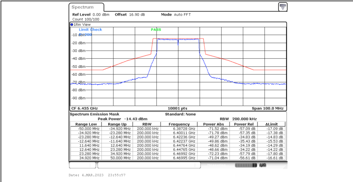
11BE20MIMO_Ant6_6435
