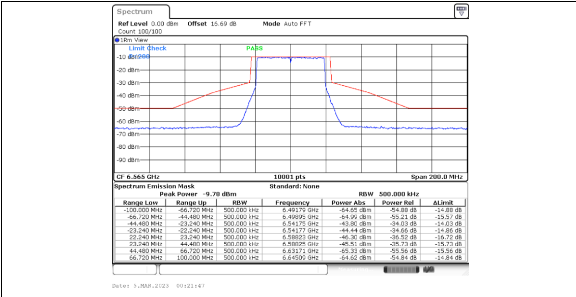
11BE40MIMO_Ant6_6565
