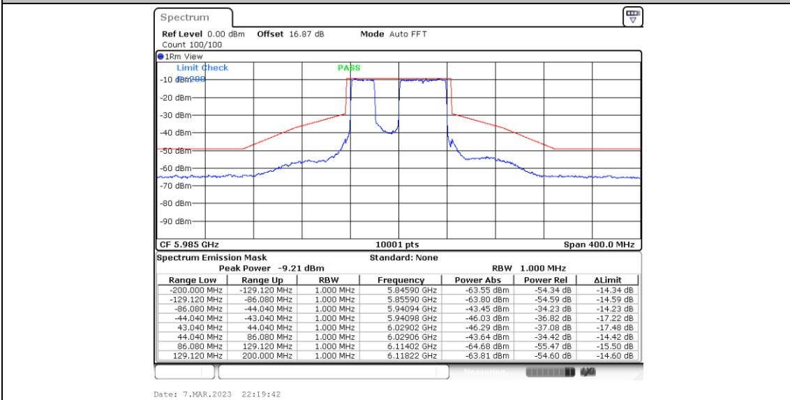
11BE80MIMO_Ant6_5985_Puncturing 20M_3
