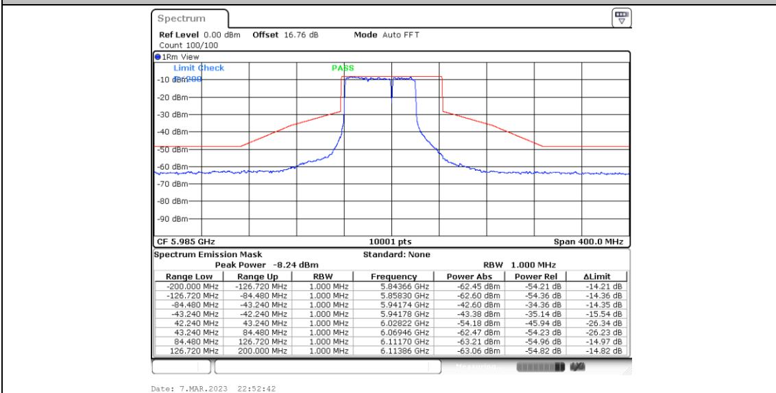
11BE80MIMO_Ant6_5985_Large RU 484+242_2
