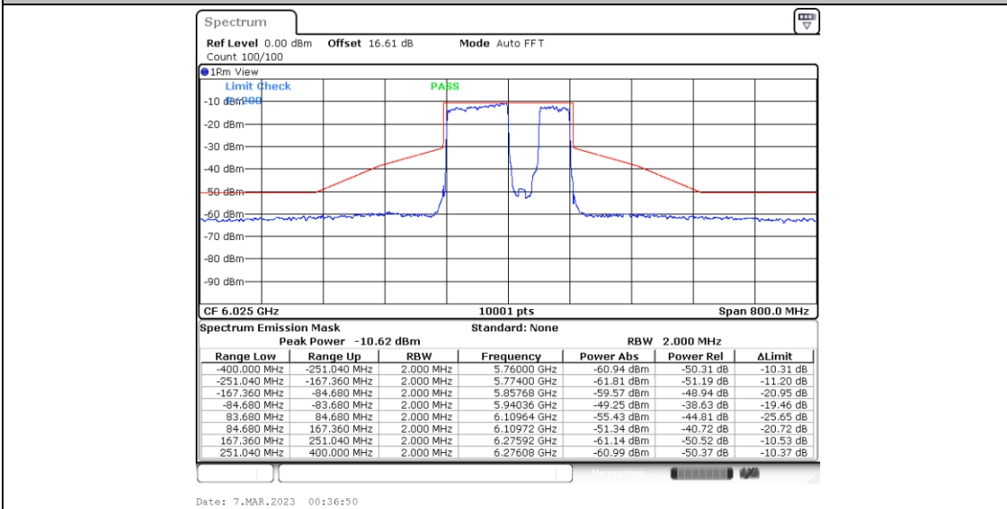
11BE160MIMO_Ant6_6025_Large RU 996+484_4
