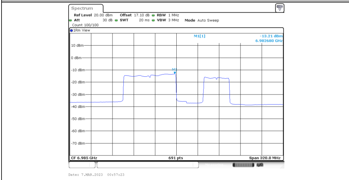
11BE160MIMO_Ant6_6985_Large RU 996+484_4
