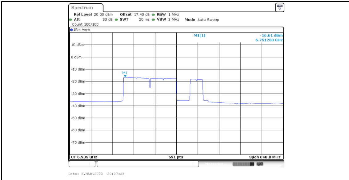
11BE320MIMO_Ant6_6905_Puncturing 80M+40M_8
