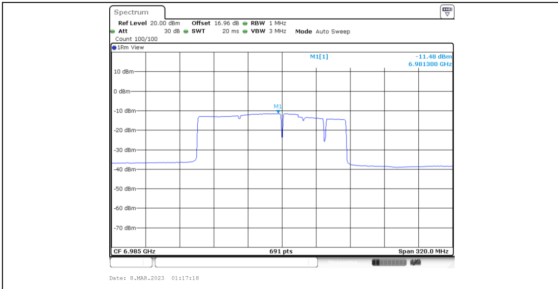
11BE160MIMO_Ant6_6985_Large RU 996+484_3
