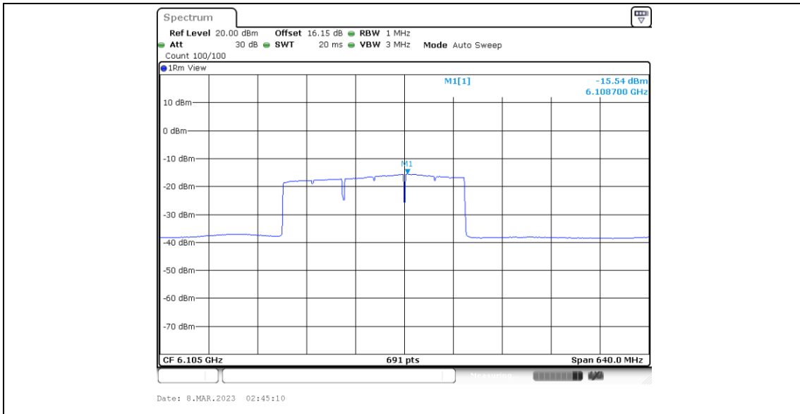
11BE320MIMO_Ant5_6105_Puncturing 40M_1
