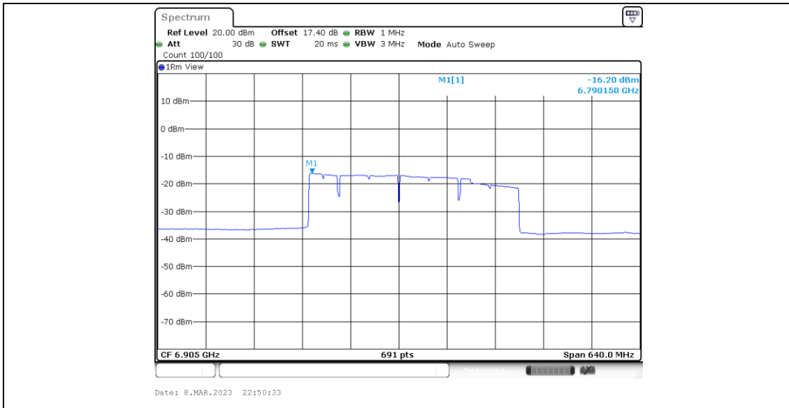
11BE320MIMO_Ant6_6905_Puncturing 40M_2
