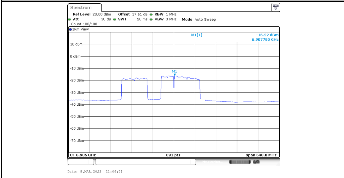
11BE320MIMO_Ant6_6905_Large RU 996*2+484_6
