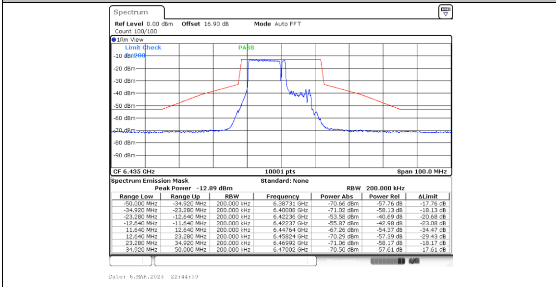
11BE20MIMO_Ant6_6435_52+26_OFDMA_1
