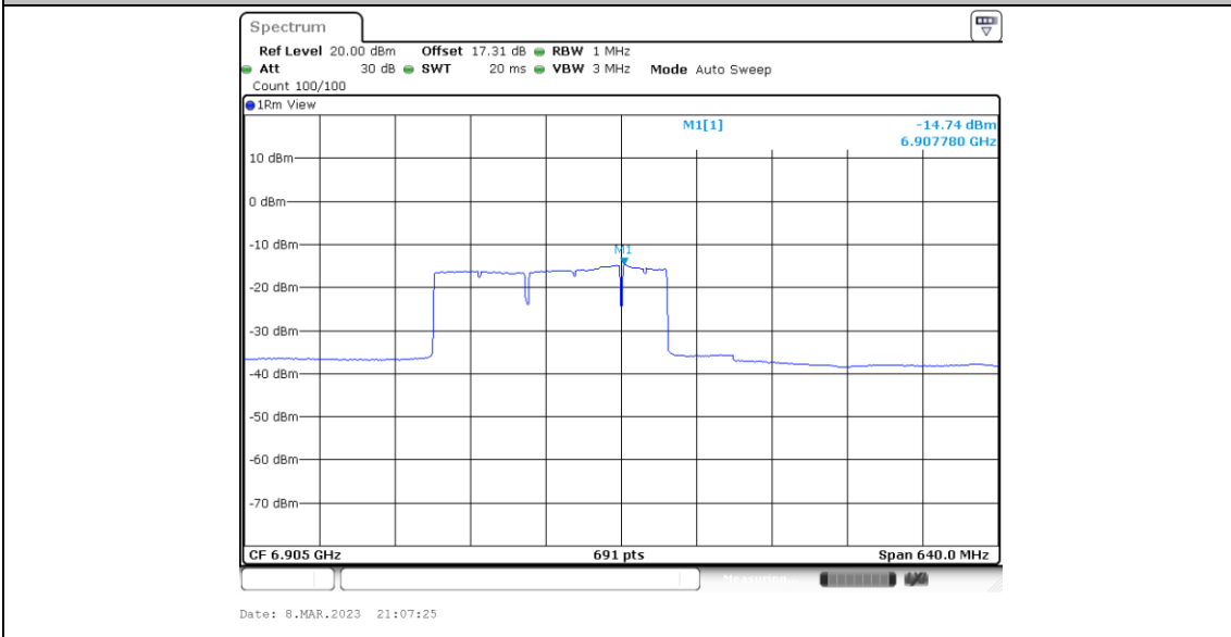
11BE320MIMO_Ant5_6905_Large RU 996*3_4
