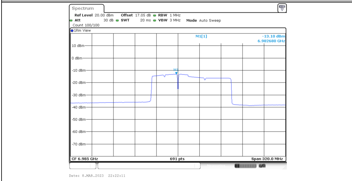
11BE160MIMO_Ant6_6985_Puncturing 40M_2
