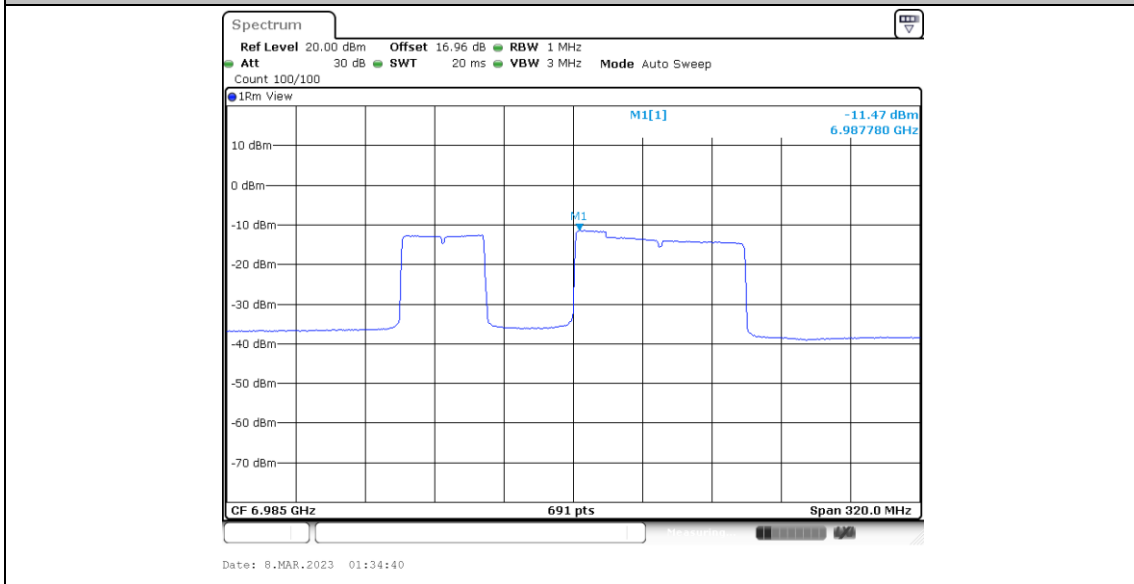
11BE160MIMO_Ant5_6985_Puncturing 40M_3
