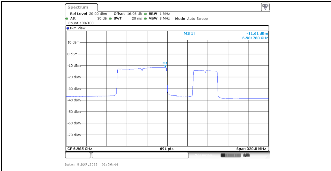
11BE160MIMO_Ant5_6985_Puncturing 40M_4
