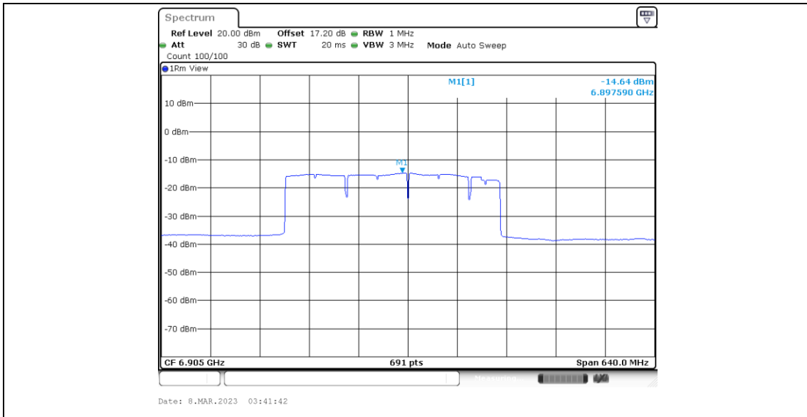
11BE320MIMO_Ant6_6905_Large RU 996*2+484_3
