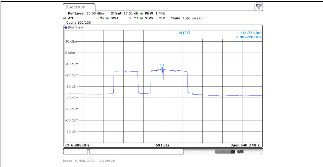
11BE320MIMO_Ant5_6905_Large RU 996*2+484_6
