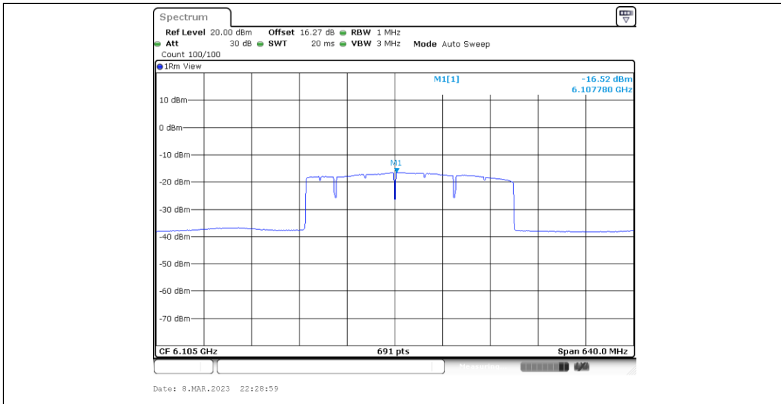
11BE320MIMO_Ant6_6105_Puncturing 40M_2
