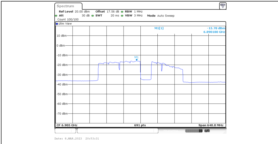
11BE320MIMO_Ant6_6905_Large RU 996*3+484_8
