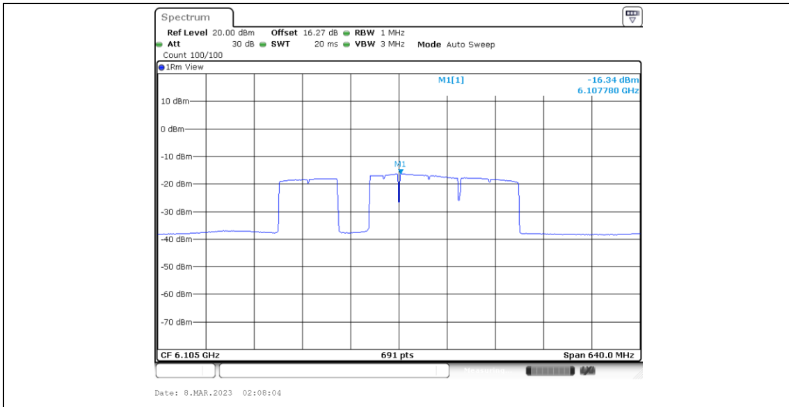
11BE320MIMO_Ant6_6105_Puncturing 40M_6
