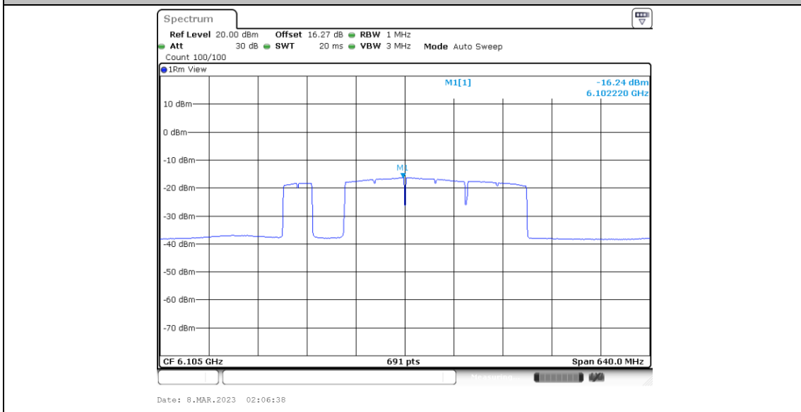
11BE320MIMO_Ant6_6105_Puncturing 40M_3
