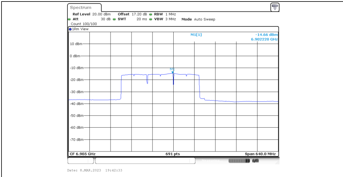
11BE320MIMO_Ant5_6905_Puncturing 40M_1
