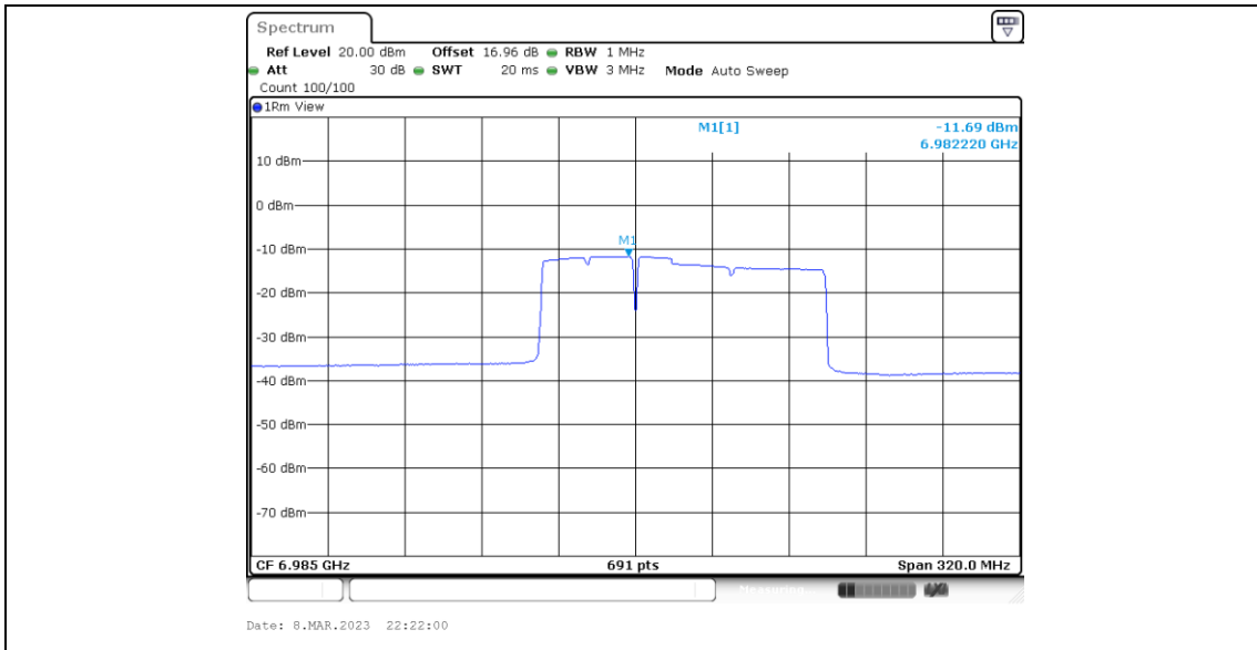
11BE160MIMO_Ant5_6985_Puncturing 40M_2
