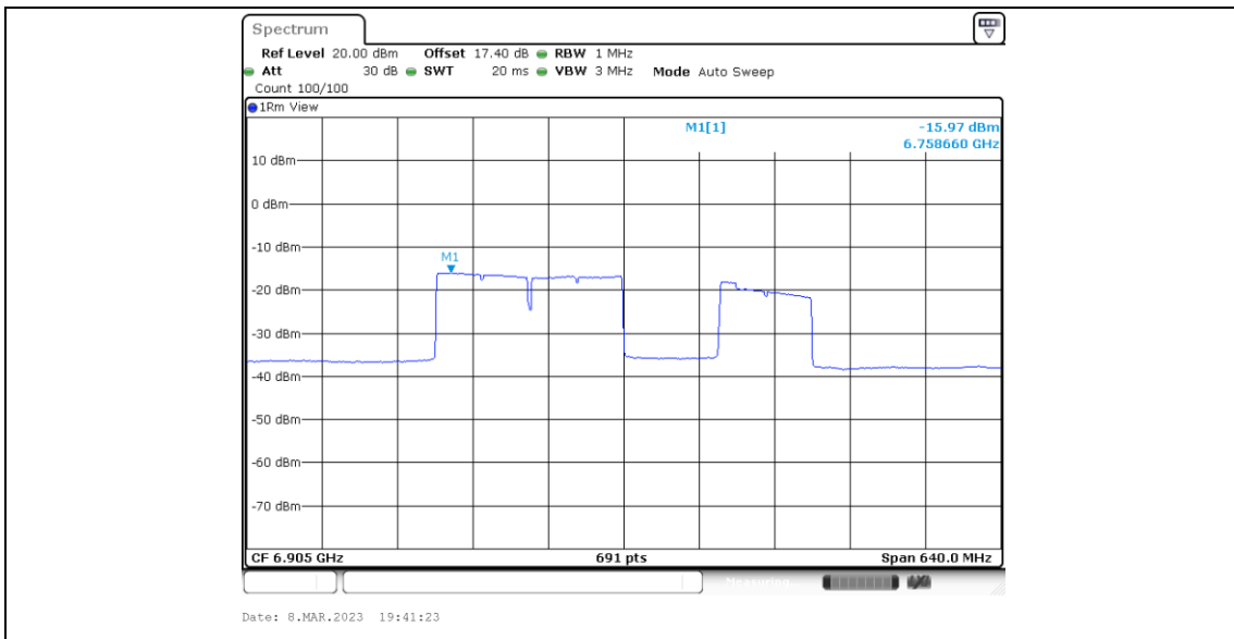
11BE320MIMO_Ant6_6905_Puncturing 80M_4
