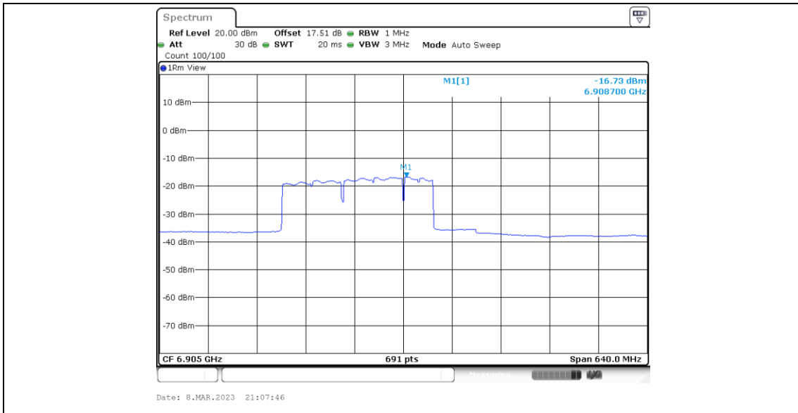
11BE320MIMO_Ant6_6905_Large RU 996*3_4
