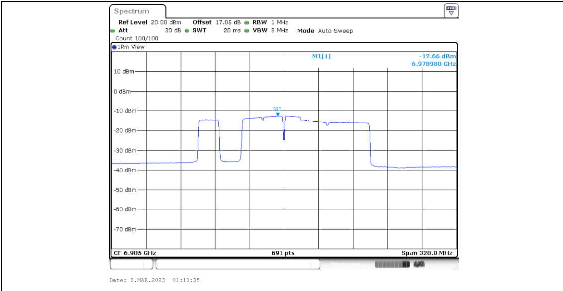
11BE160MIMO_Ant6_6985_Puncturing 20M_4
