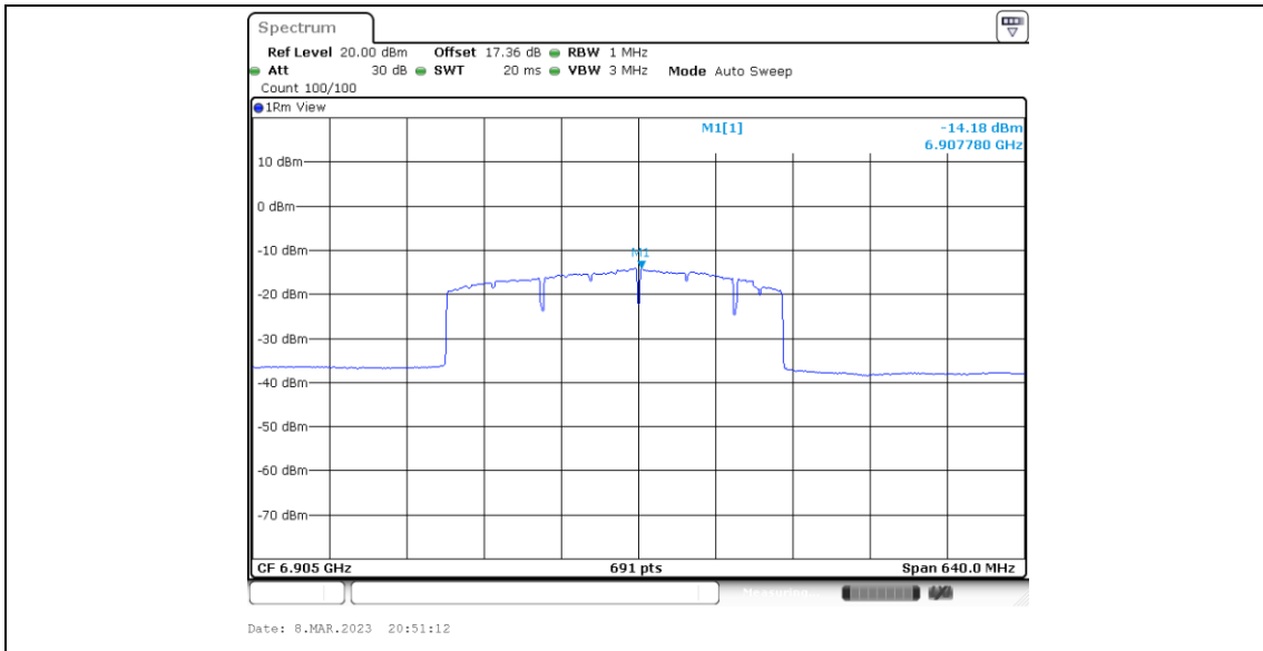
11BE320MIMO_Ant5_6905_Puncturing 80M+40M_1
