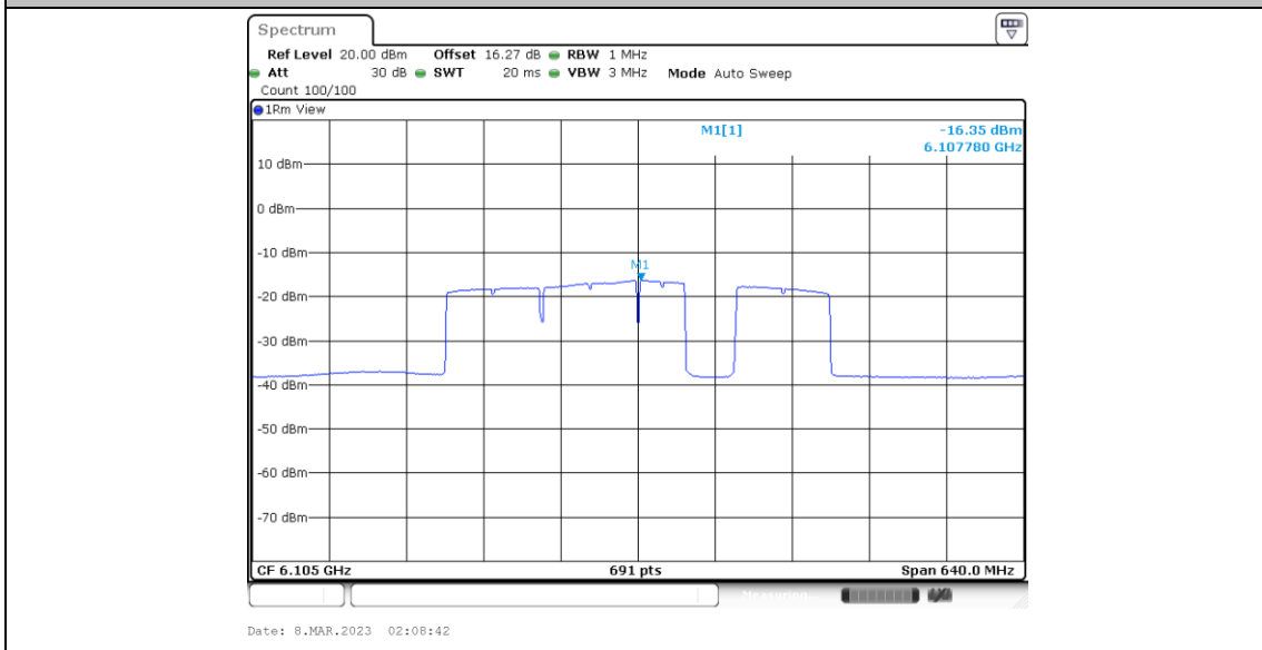
11BE320MIMO_Ant6_6105_Puncturing 40M_7
