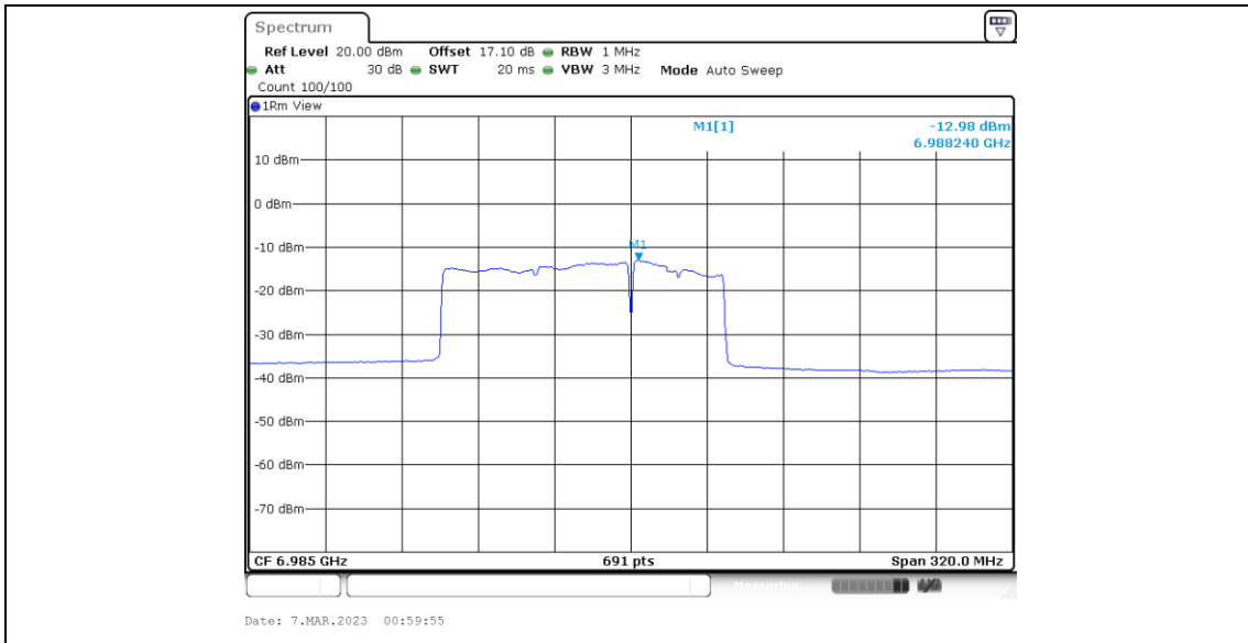
11BE160MIMO_Ant6_6985_Puncturing 40M_1
