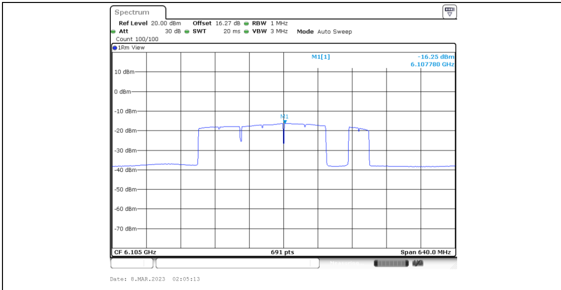
11BE320MIMO_Ant6_6105_Puncturing 40M_8
