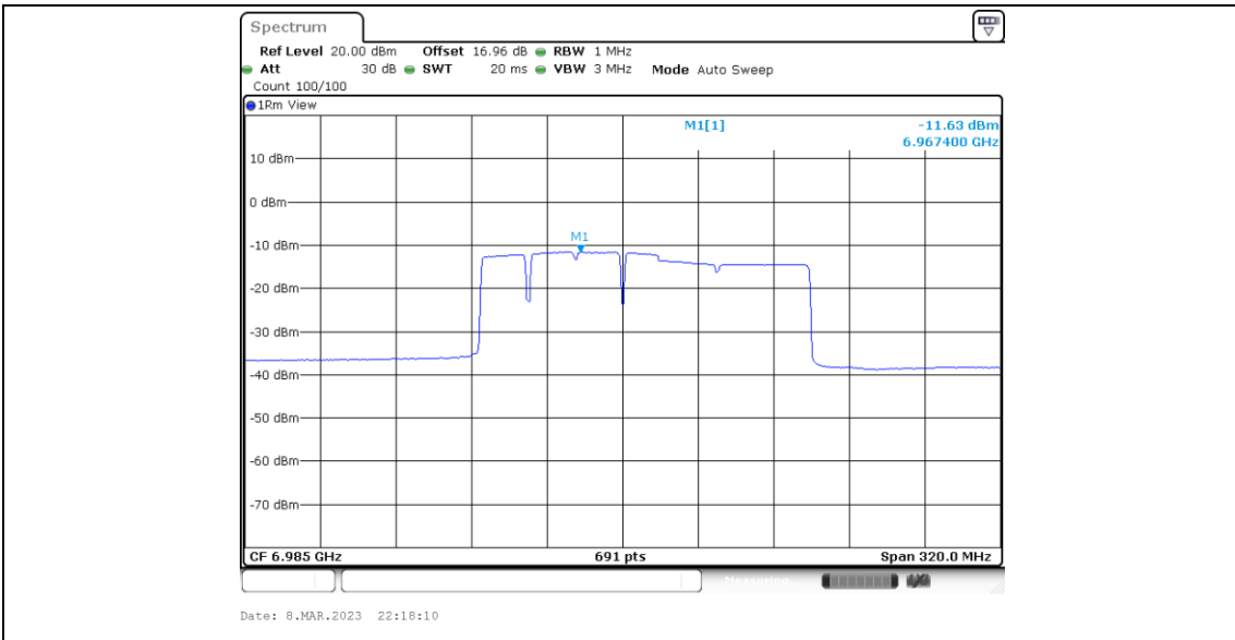
11BE160MIMO_Ant5_6985_Puncturing 20M_2
