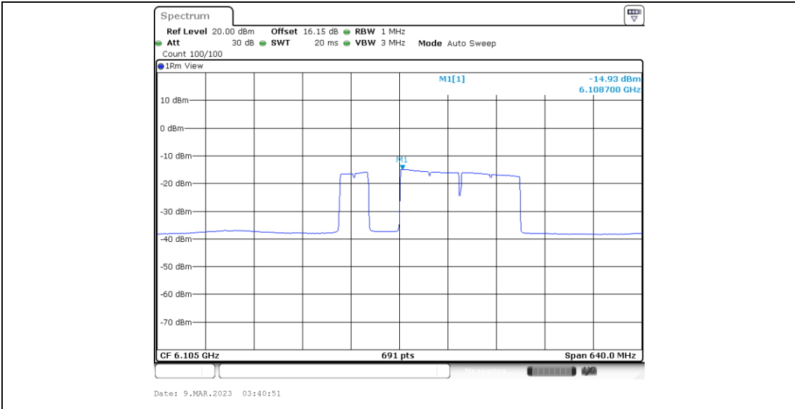
11BE320MIMO_Ant5_6105_Puncturing 80M_1
