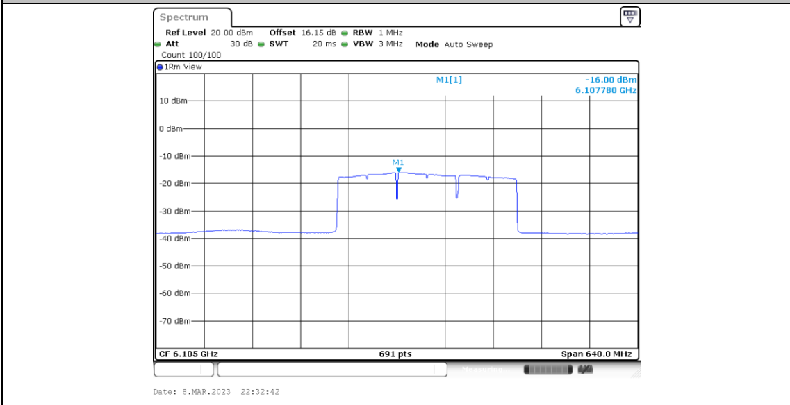
11BE320MIMO_Ant5_6105_Puncturing 80M_2
