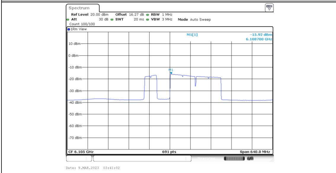
11BE320MIMO_Ant6_6105_Puncturing 80M_1
