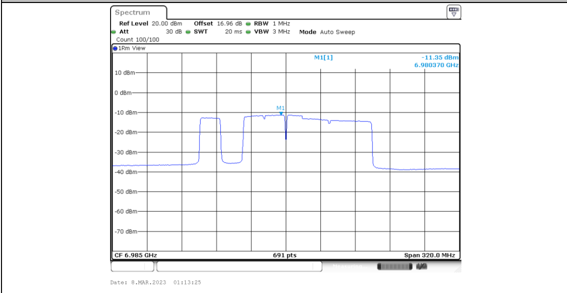
11BE160MIMO_Ant5_6985_Puncturing 20M_4
