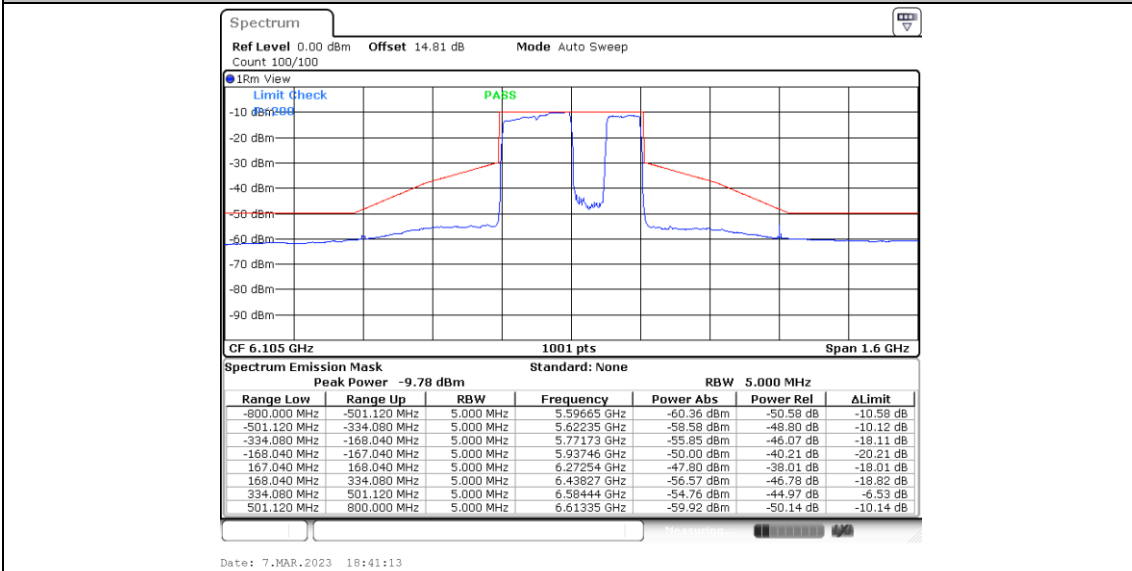
11BE320MIMO_Ant5_6105_Puncturing 80M_4
