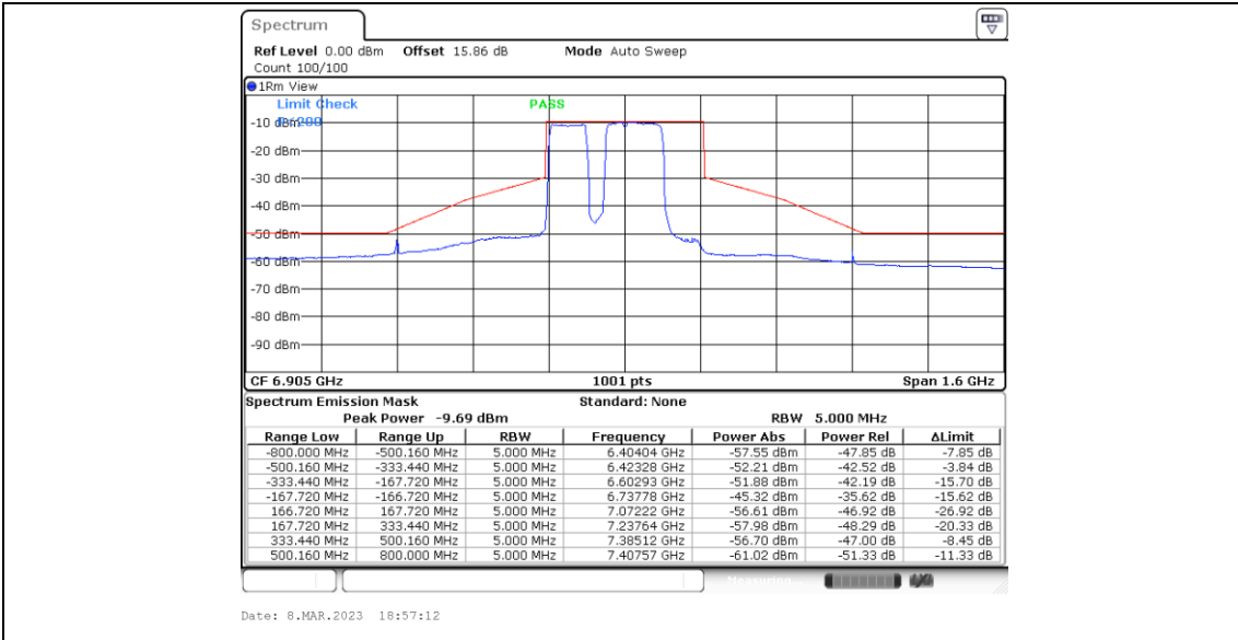
11BE320MIMO_Ant5_6905_Large RU 996*2+484_6
