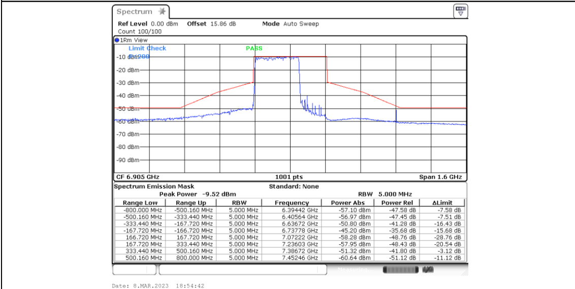
11BE320MIMO_Ant5_6905_Large RU 996*3_4
