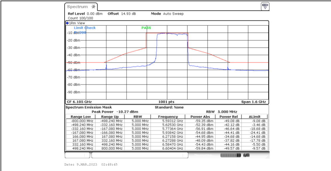
11BE320MIMO_Ant4_6105_Puncturing 80M_2
