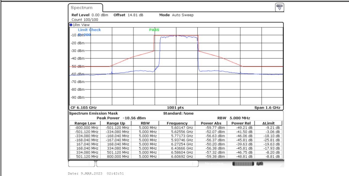
11BE320MIMO_Ant5_6105_Puncturing 40M_2
