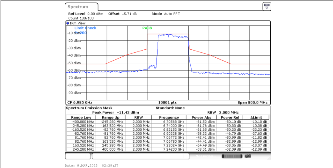
11BE160MIMO_Ant4_6985_Puncturing 40M_2
