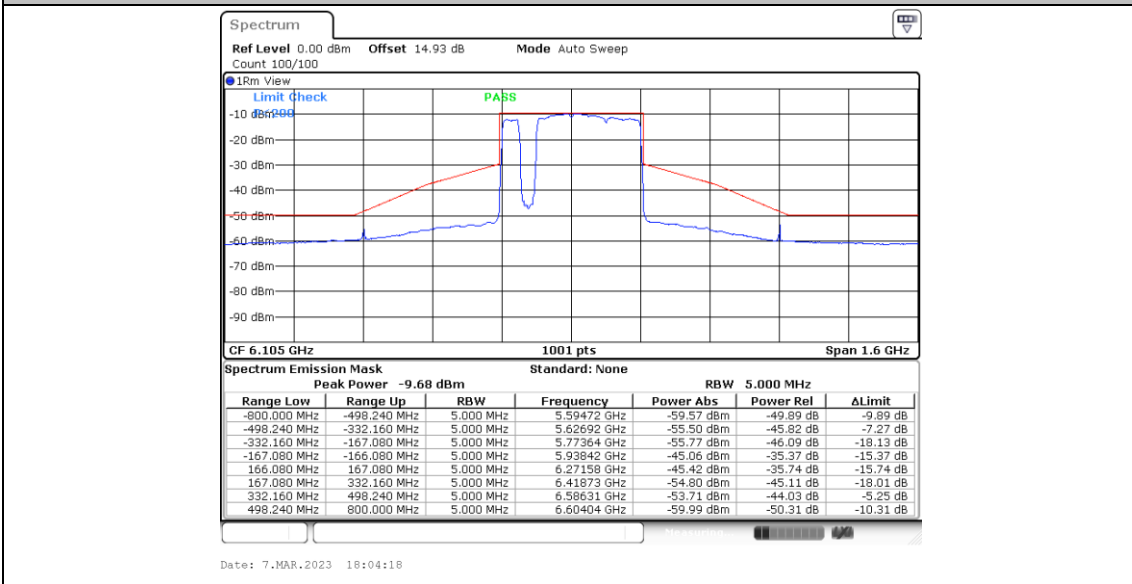
11BE320MIMO_Ant4_6105_Puncturing 40M_3
