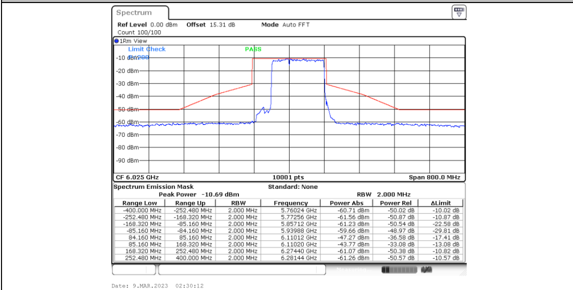
11BE160MIMO_Ant4_6025_Puncturing 40M_2
