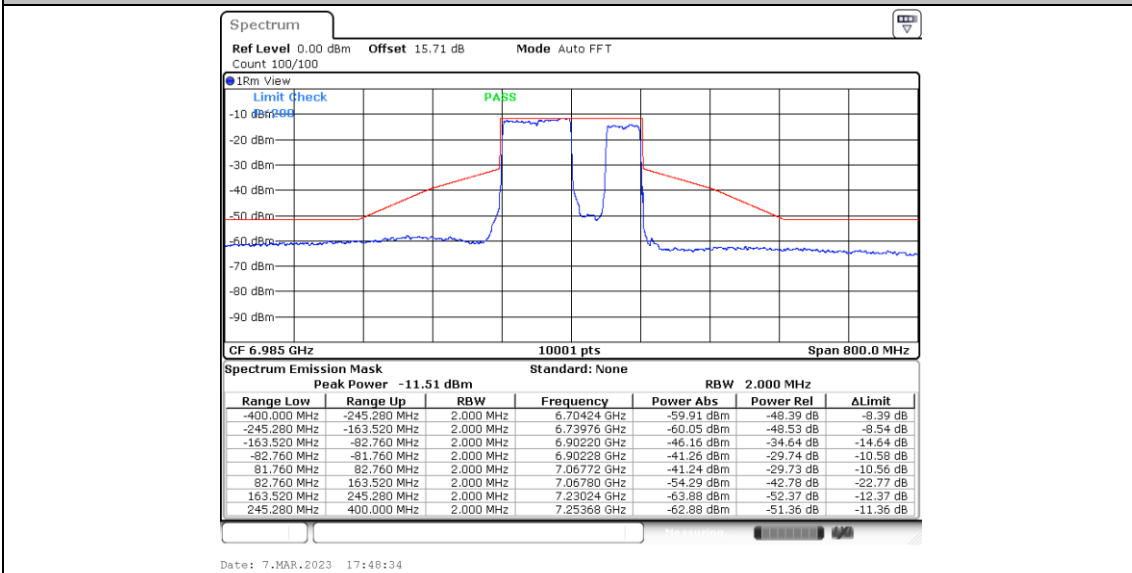
11BE160MIMO_Ant4_6985_Puncturing 40M_4
