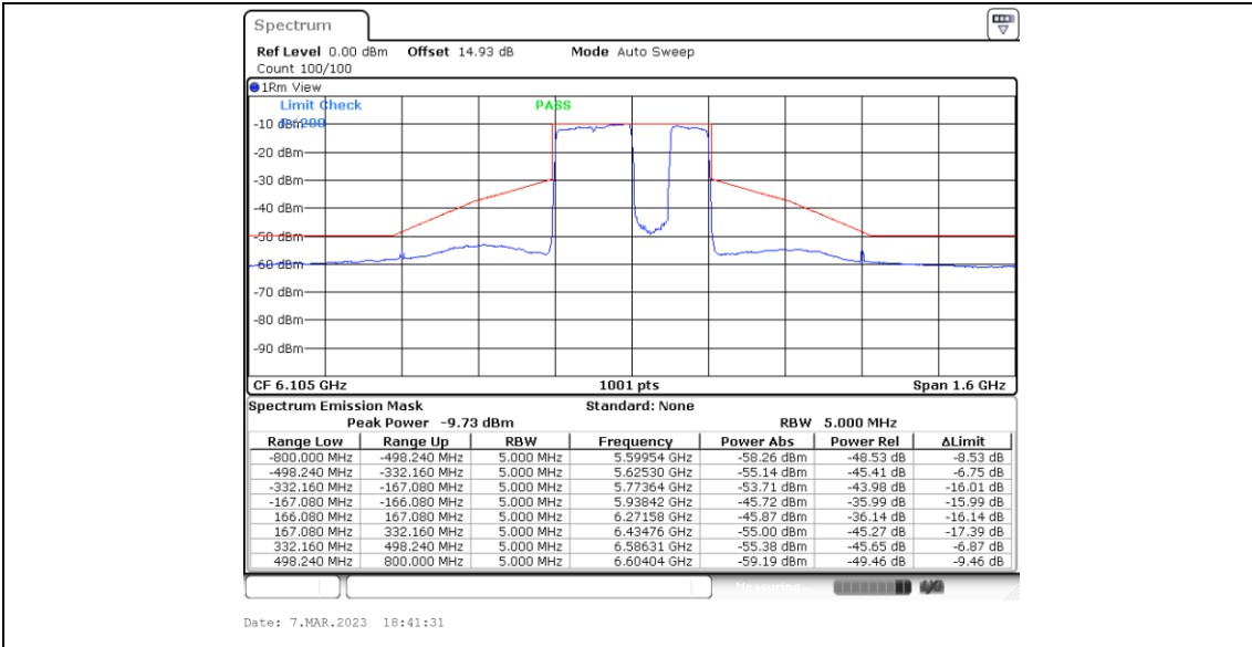
11BE320MIMO_Ant4_6105_Puncturing 80M_4
