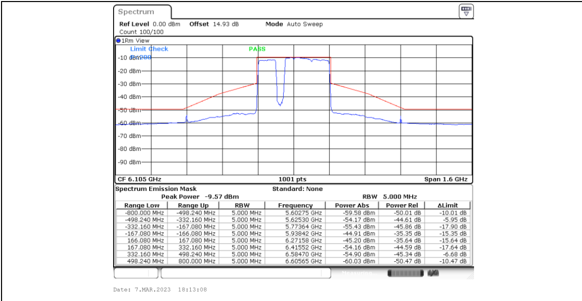
11BE320MIMO_Ant4_6105_Puncturing 40M_6
