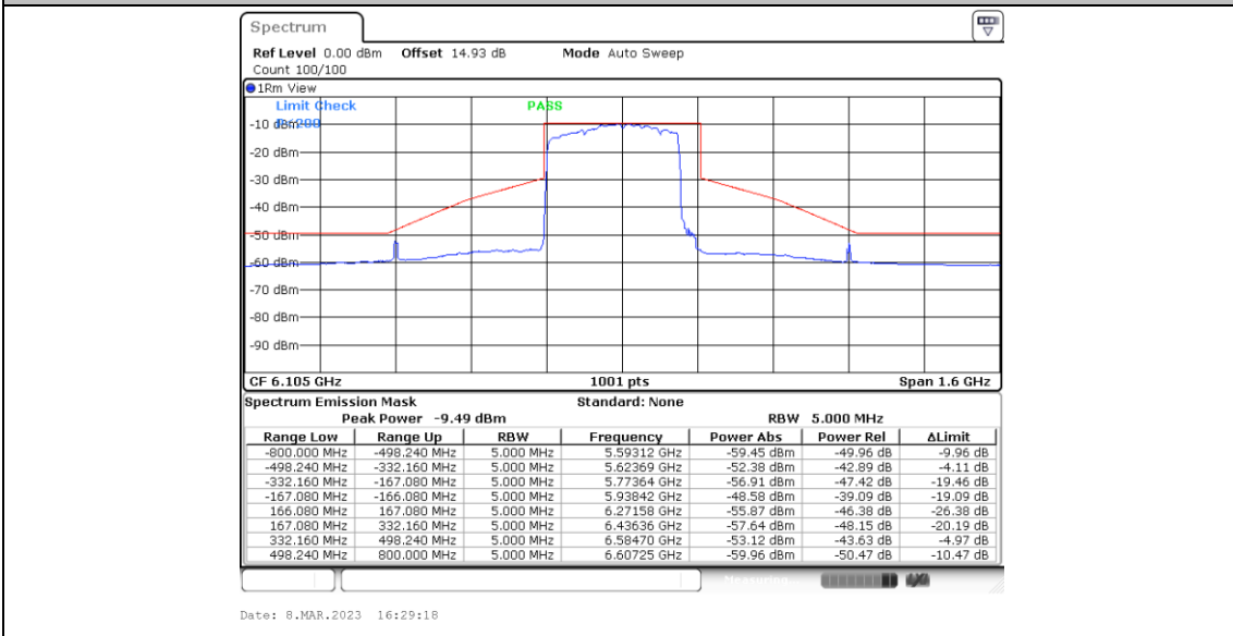
11BE320MIMO_Ant4_6105_Puncturing 80M+40M_1
