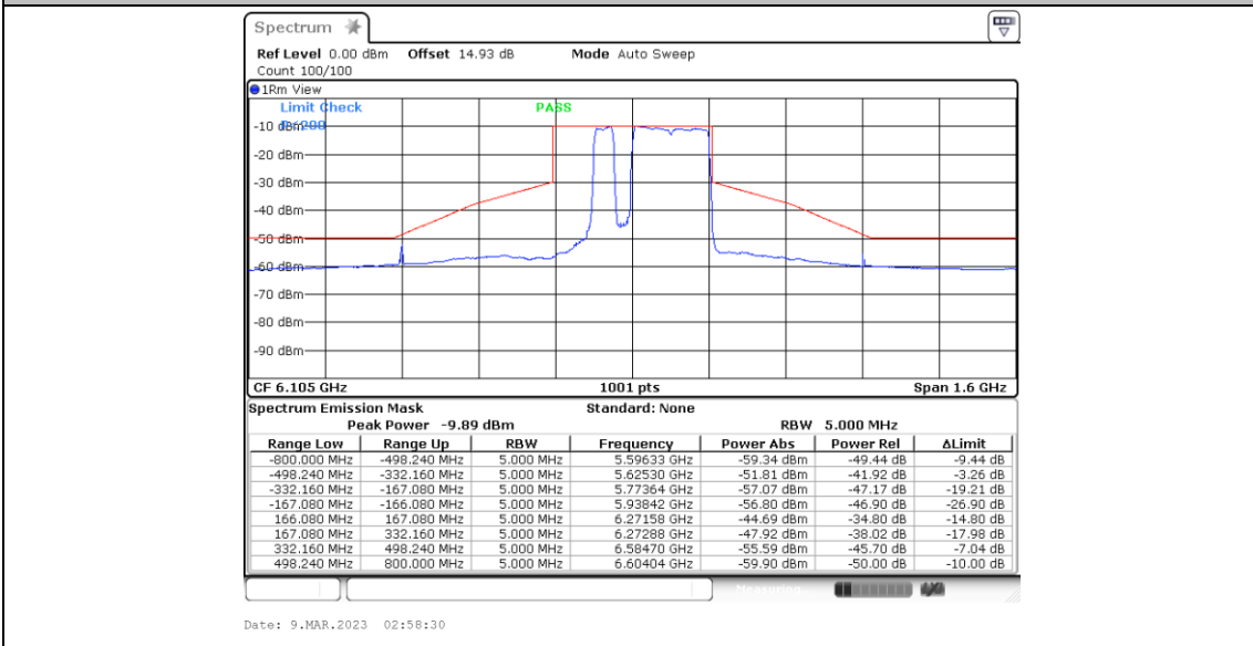
11BE320MIMO_Ant4_6105_Puncturing 80M_1
