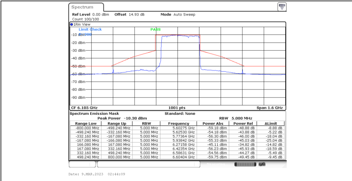
11BE320MIMO_Ant4_6105_Puncturing 40M_2
