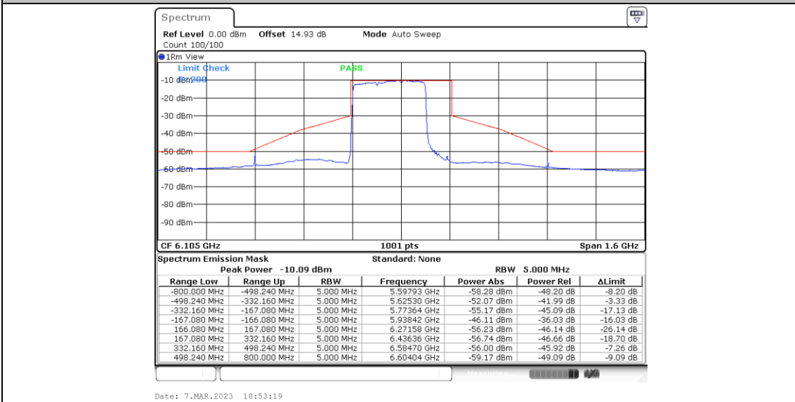
11BE320MIMO_Ant4_6105_Puncturing 40M_1
