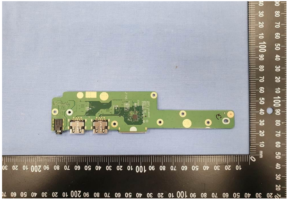
EUT Photo (12)
