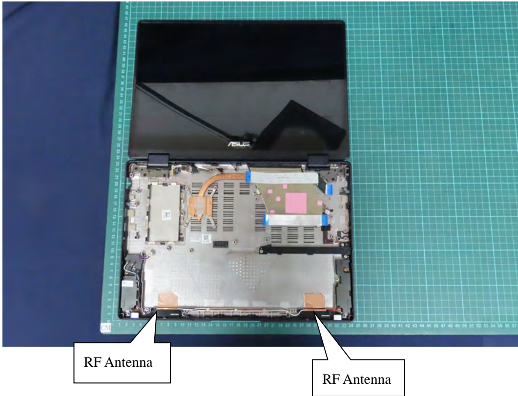
(21) EUT Photo
