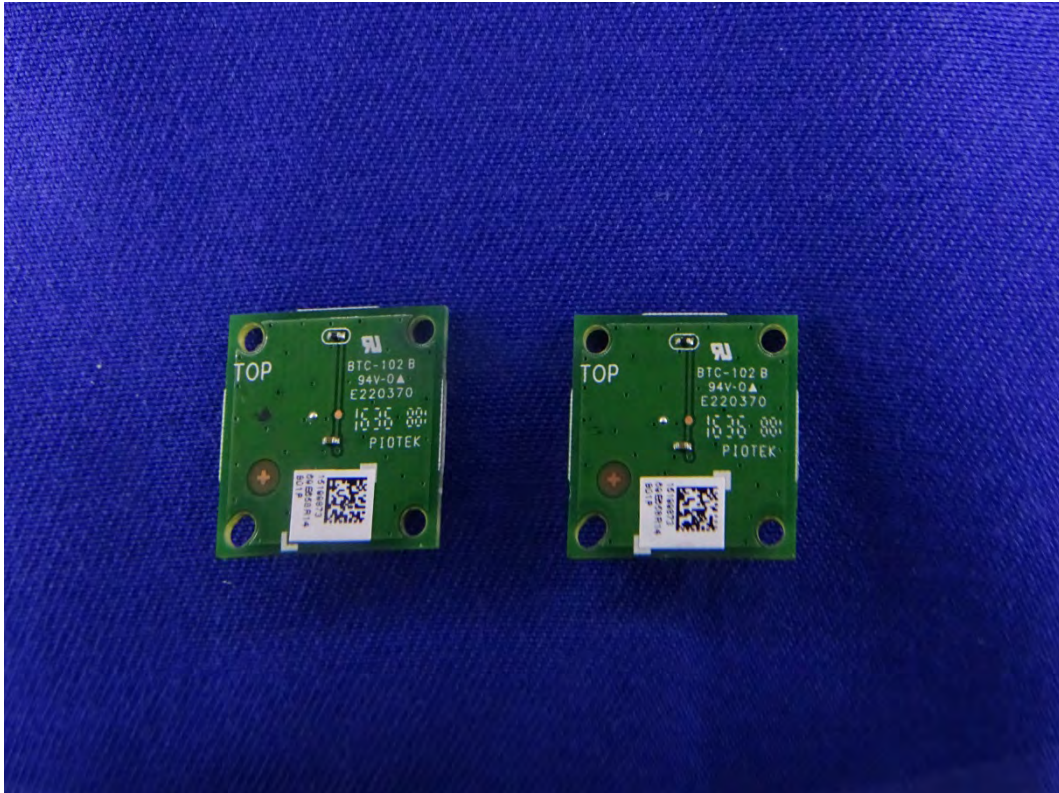
(129) EUT Photo
