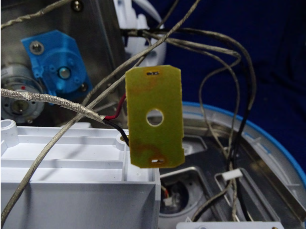
(133) EUT Photo
