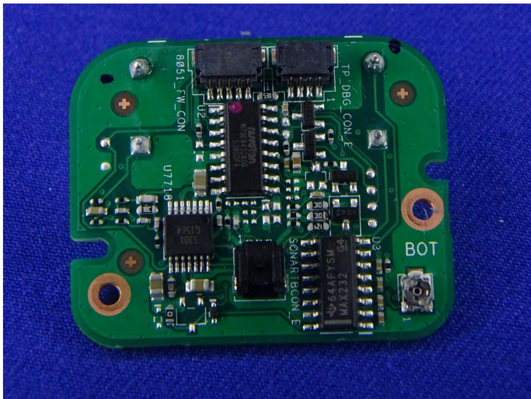
(74) EUT Photo
